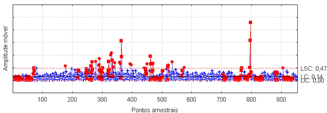
Figura 37 – Gráfico \overline{MR} do índice de acidez, considerando os dados originais
