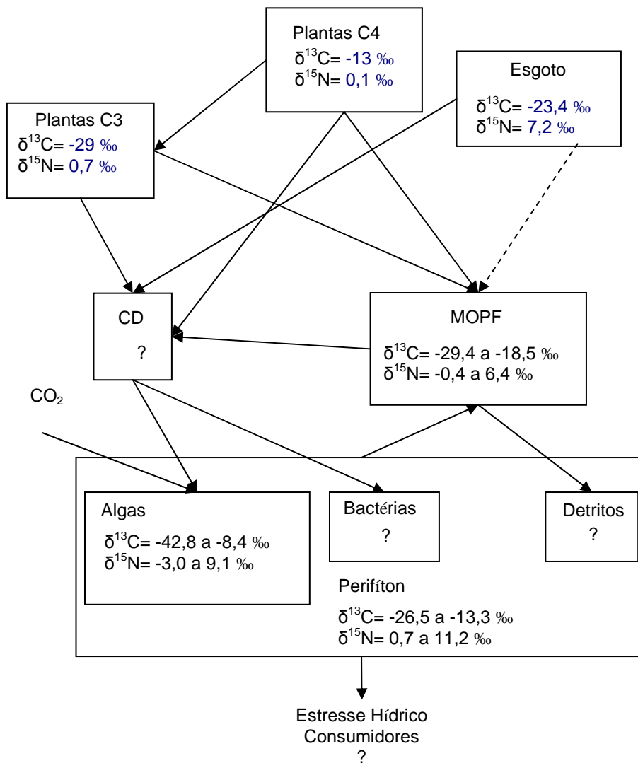
Figura 25. Resumo dos valores das composições isotópicas no modelo conceitual. Os valores de algas filamentosas foram colocadas no compartimento do perifíton. Os valores de esgoto, plantas C3 e C4 foram de dados da literatura. As interrogações mostram as lacunas do conhecimento. A linha tracejada mostra que o material particulado não é formado, ou sua maior parte não é formada, pelas fontes antropogênicas. Os valores em azul são Detweiler (2005).
