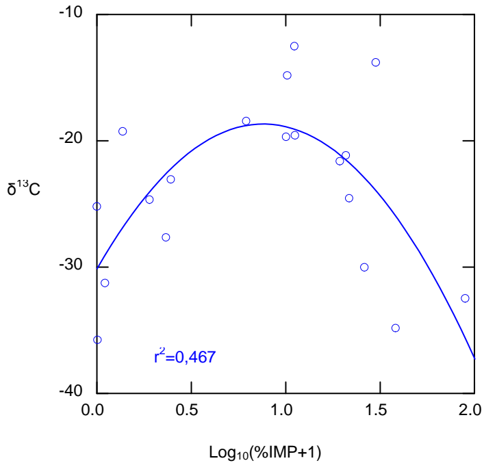
Figura 23. Regressão não-linear entre \delta^{13}\text{C} das algas filamentosas e \text{Log}_{10}(\% \text{IMP}+1) da Bacia Hidrográfica Guapi-Macacu. O modelo utilizado foi uma função quadrática y=a*x^2+b*x+c . O vértice da curva que representa a mudança da variação de \delta^{13}\text{C} equivale a \delta^{13}\text{C}=-18,53 e \text{Log}_{10}(\% \text{IMP}+1)=0,87 que tem impacto equivalente a 6,58%. O valor de c equivale a \delta^{13}\text{C} na ausência de impacto que é -29,985.
