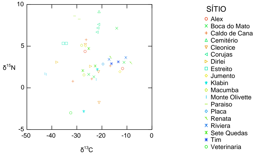
Figura 15. Valores de \delta^{13}\text{C} e \delta^{15}\text{N} em per mil (‰) das algas filamentosas agrupadas por sítio amostral. Legenda à direita do gráfico. Existe uma maior proximidade em relação aos sítios amostrados que em relação aos agrupamentos taxonômicos.
