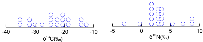
Figura 17. Gráficos de densidade de pontos das variáveis testadas lado a lado com a densidade de pontos das variáveis transformadas para o teste. Todos os valores foram logaritmizados com exceção de \delta^{13}\text{C} e \delta^{15}\text{N} das algas filamentosas.
