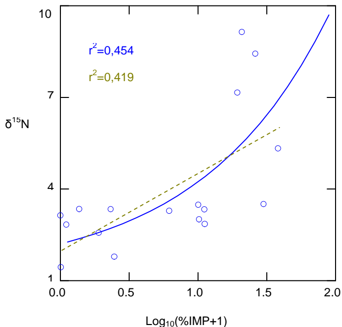
Figura 24. Comparação das regressões. Regressão não-linear entre \delta^{15}\text{N} das algas filamentosas e \text{Log}_{10}(\% \text{IMP}+1) na Bacia Hidrográfica Guapi-Macacu. O modelo exponencial representado pela linha azul explica melhor o modelo linear representado pela linha tracejada amarela (maior r^2 mostrado no gráfico). O modelo utilizado foi uma função exponencial y=a*x^b+c . O valor de c representa o \delta^{15}\text{N} na ausência de impacto e equivale a 1,29. Não foram incluídos neste gráfico os pontos referentes aos sítios KL e VE os quais ficam fora da escala do modelo.
