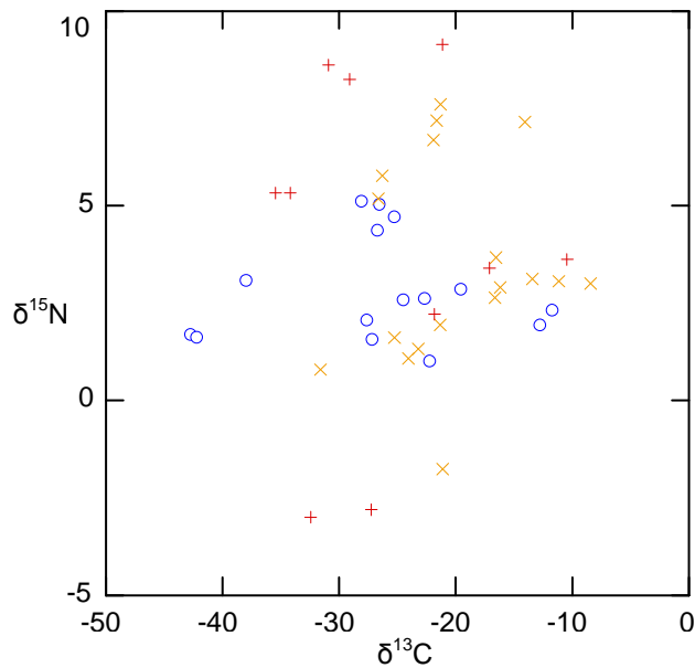
Figura 16. Média dos valores de \delta^{13}\text{C} e \delta^{15}\text{N} das algas filamentosas em per mil (‰). Dos 25 riachos apenas 19 apresentaram espécimes de algas. Os sítios foram agrupados pela classificação a priori . Legenda: Sítios de Referência (○), Intermediários (×) e Impactados (+).
