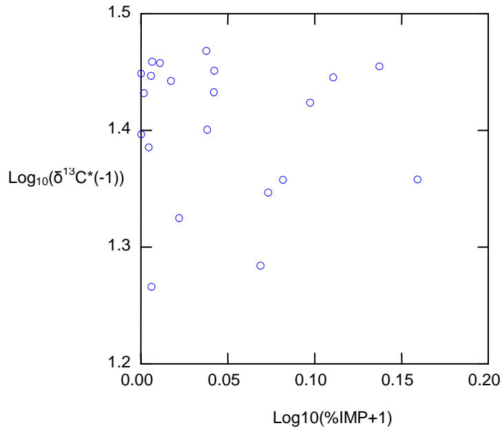
Figura 21. Valores de \text{Log}_{10}(\delta^{13}\text{C}^*(-1)) contra \text{Log}_{10}(\% \text{IMP}+1) . A disposição dos pontos não sugere nenhuma relação de dependência entre esta variável resposta e a variável independente que descreve impacto da Bacia Hidrográfica Guapi-Macacu.
