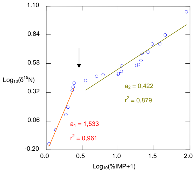
Figura 20. Interpretação da relação não-linear entre \text{Log}_{10}(\delta^{15}\text{N}) em relação a \text{Log}_{10}(\% \text{IMP}+1) . Os intervalos foram separados pelo ponto de inflexão indicado no gráfico pela seta. Nota-se que o valor de \text{Log}_{10}(\% \text{IMP}+1)=0,4 equivalente a \% \text{IMP}=1,5\% separa o comportamento da função. Antes desse ponto o coeficiente de inclinação equivale a a_1=1,533 e depois a a_2=0,422 .
