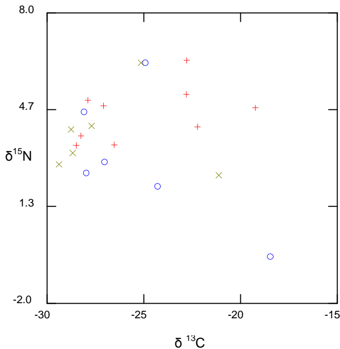
Figura 10. Valores de \delta^{13}\text{C} e \delta^{15}\text{N} em per mil (‰) do MOPF em 21 riachos da bacia hidrográfica do rio Guapi-Macacús. Legenda: pontos de referência (o), intermediários (x) e impactados (+), segundo a classificação a priori
