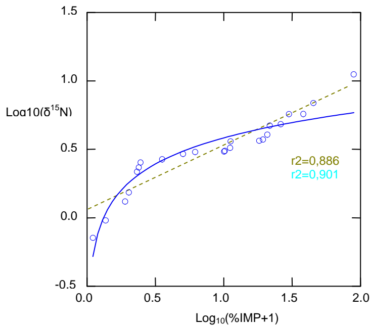
Figura 19. Comparação entre a regressão linear e a logarítmica dos valores de \text{Log}_{10}(\delta^{15}\text{N}) do perifiton em relação a \text{Log}_{10}(\% \text{IMP}+1) . A relação logarítmica de modelo y=a*x^b está representada pela curva azul e apresenta um r^2 mais alto que a relação linear y=a*x+c representada pela linha tracejada amarela.
