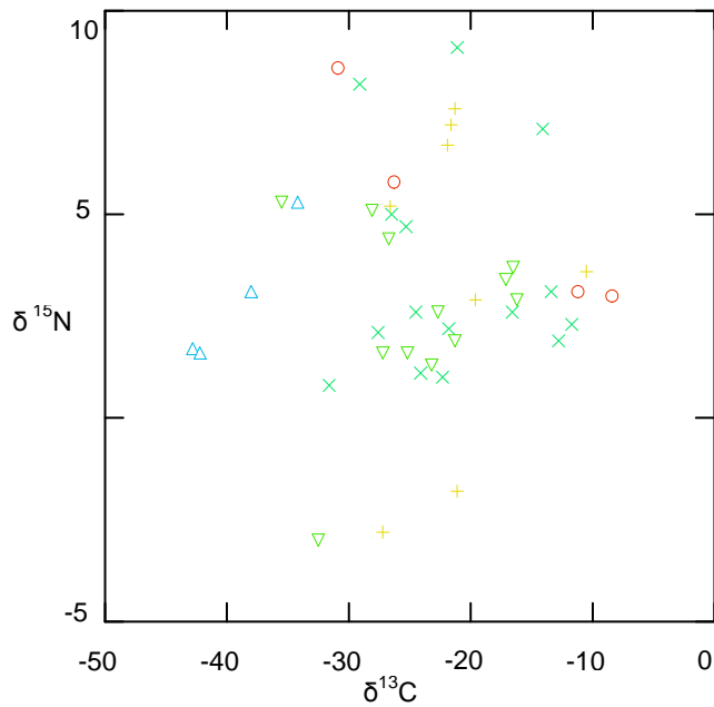
Figura 13. Valores de \delta^{13}\text{C} e \delta^{15}\text{N} em per mil (‰) de das Superclasses de 43 algas filamentosas em 19 riachos da bacia hidrográfica do rio Guapi-Macacús. Legenda: Chlorophyceae (○), Cyanophyceae (×), Oedogoniophyceae (+), Rhodophyceae (Δ) e Zignemaphyceae (▽).
