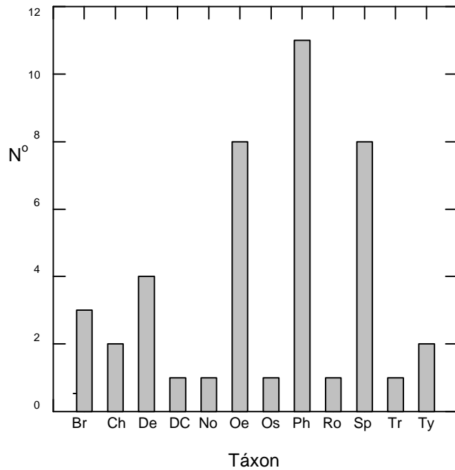
Figura 11. Contagem dos táxons das algas presentes em 19 dos 25 riachos amostrados da Bacia Hidrográfica Guapi-Macacu. Legenda: Br – Batrachospermum , Ch – Chlorophyta, De – Desmidium , DC – Diatomaceae, Chlorophyta e Detritos, No – Nostoc , Oe – Oedogonium , Os – Oscillatoria , Ph – Phormidium , Ro – Rhodophyceae, Sp – Spyrogira , Tr – Trentepohlia , Ty - Tyconema
