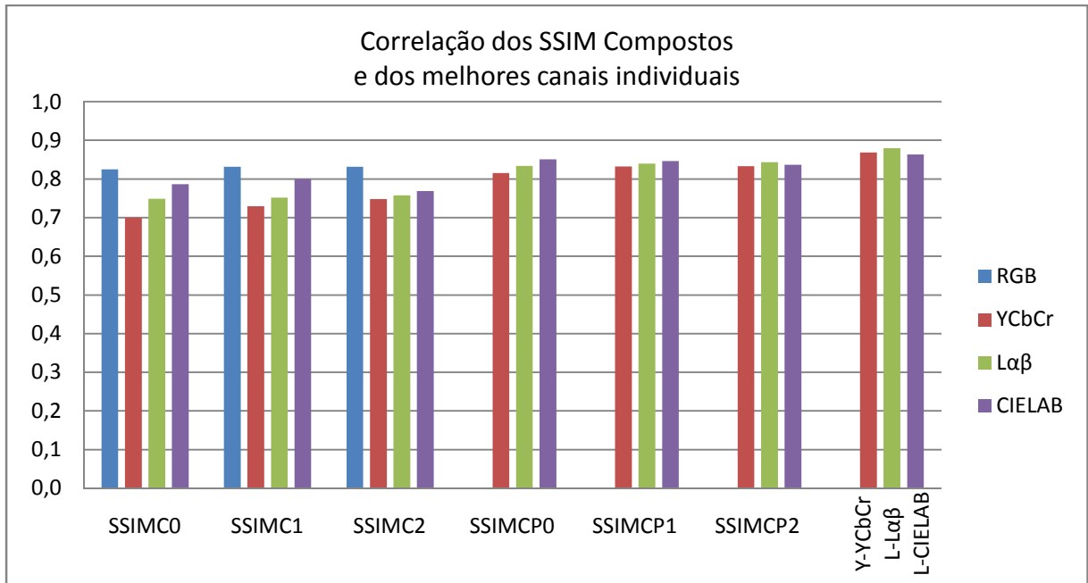
Figura 37 – Correlações entre DMOS e SSIM com ajuste no banco de dados LIVE para os cálculos dos SSIM Compostos e SSIM dos canais individuais com maior correlação.
