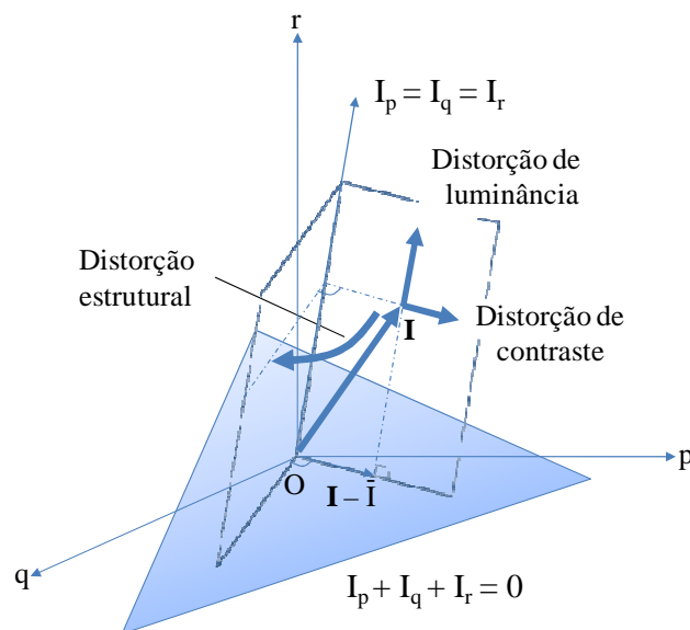
Figura 13 – Separação das distorções de luminância, de contraste e estrutural da imagem de referência I . Inspirado em (26).
