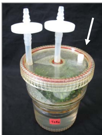
Figura 2 – Recipiente do biorreator de imersão temporária RITA ® , com a saída de ar adicional incorporada à tampa do frasco.
