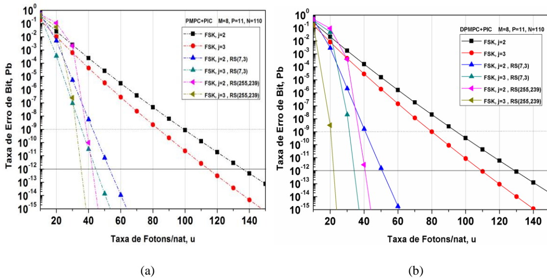
Figura 5.16. BER versus taxa de fótons/nat, u , considerando N = 110 usuários simultâneos para M=8 no sistema FSK+ PIC, com e sem FEC. , (a) PMPC, b) DPMPC.
