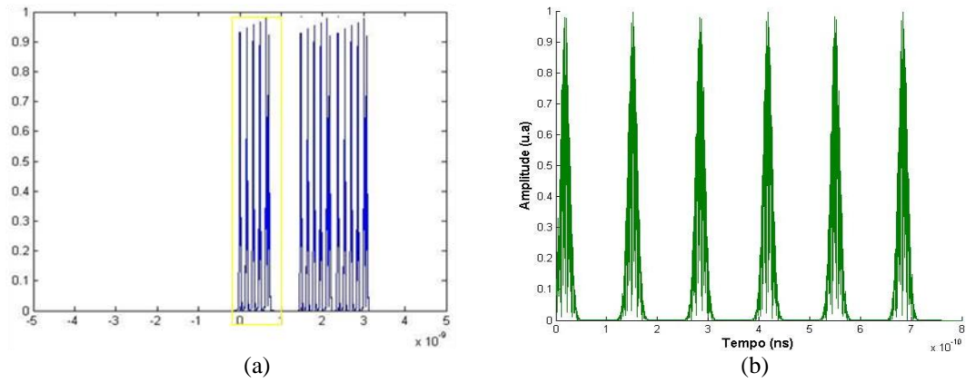
Figura 3.8: a) Seqüência de bits (1,0,1,1) obtida pela codificação (C00) PMPC.
