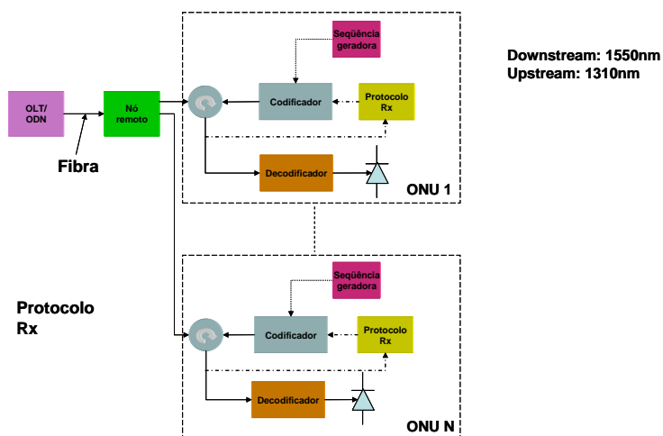
Figura 2.9: ONU para OCDMA- PON.
