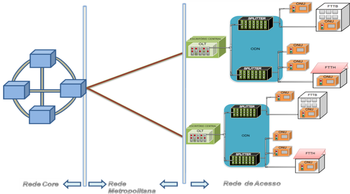
Figura 2.1: Hierarquia das Redes.
