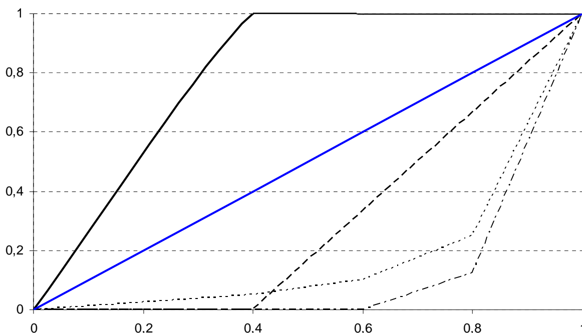
Figura 1 – curva de Lorenz e as curvas de concentração do exemplo
