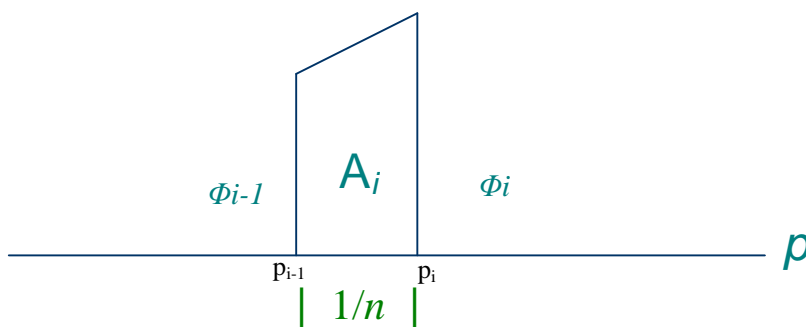
Figura 6 – Um dos trapézios que formam a área \beta .
