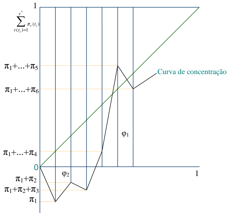
Figura 7 – Curva de concentração
