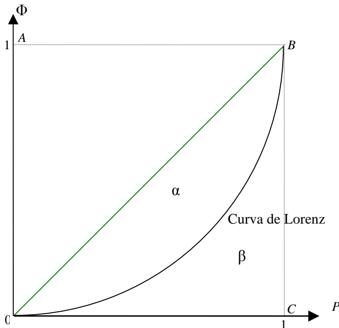
Figura 5 – curva de Lorenz
