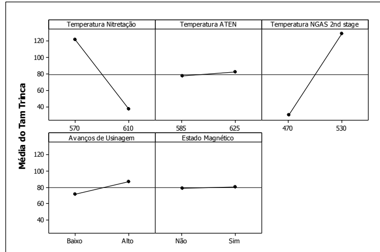
Figura 4.6: Gráfico de efeito das variáveis nas médias de ocorrência de trincas.
