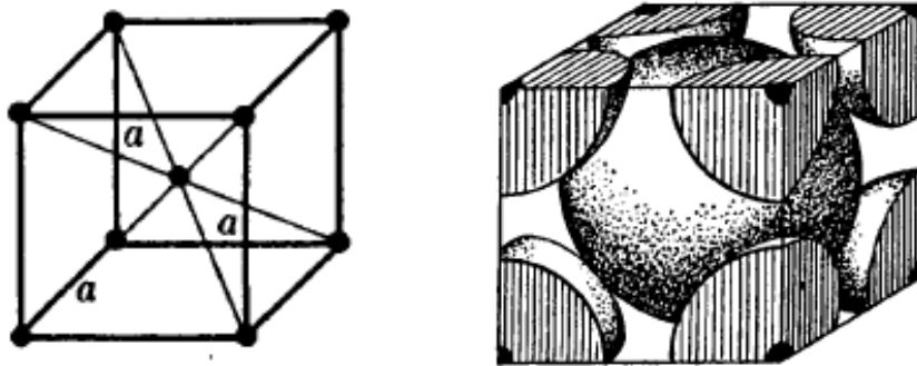
Fig. 2.2: Reticulado cristalino Cúbico de Corpo Centrado. Fonte: Padilha (1997).
