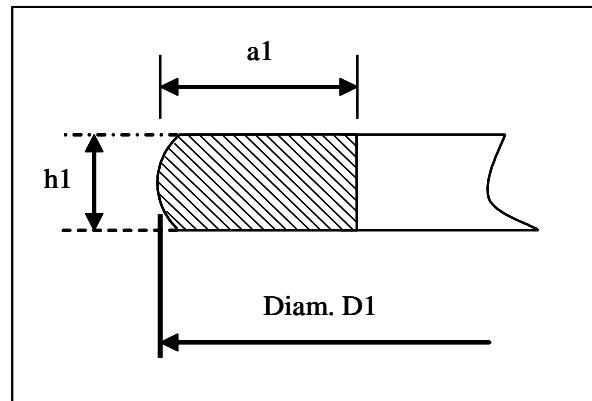
Fig. 1.6: Croqui de anel de pistão de aço inoxidável martensítico nitretado. Fonte ISO 6621, (2003).
