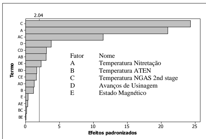
Figura 4.4: Gráfico de Pareto para os termos do modelo de regressão.
