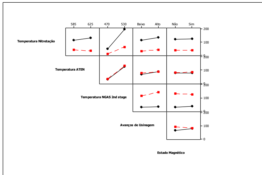
Figura 4.7: Gráfico de interações das variáveis nas médias de ocorrência de trincas.
