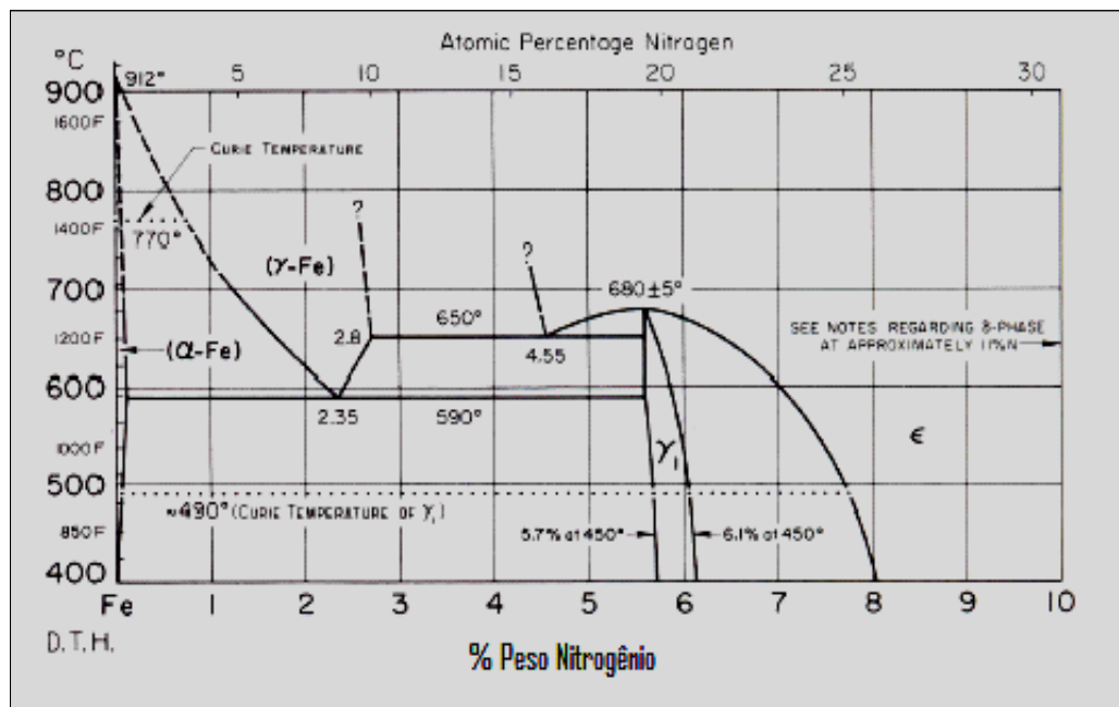
Figura 2.6: Diagrama de equilíbrio Fe-N. Fonte: Ghiglione et al. (1994).
