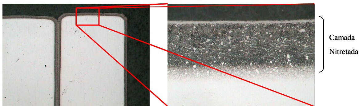
Fig. 1.4 – Micrografia de anéis de aço nitretados, na esquerda 25 X e na direita detalhe com 300X. Ataque Nital 2%. Fonte: Mahle (2008).
