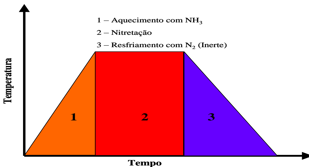
Figura 2.9: Esquema simplificado de um processo típico de nitretação.
