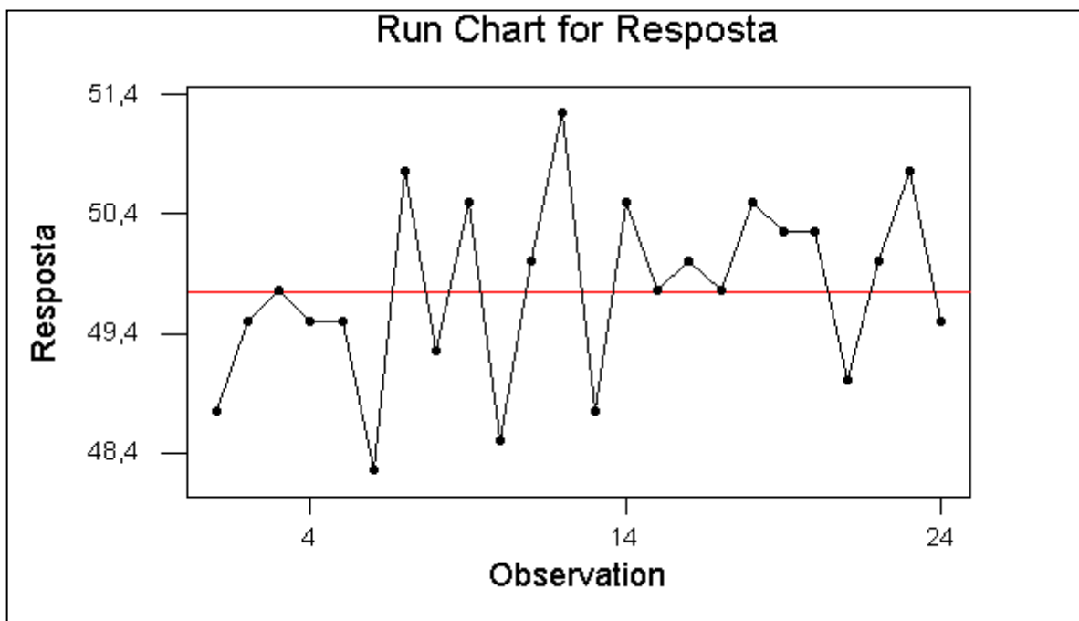
Figura 3.6: Exemplo de gráfico de dados brutos ( run-chart ). Fonte: Minitab®.
