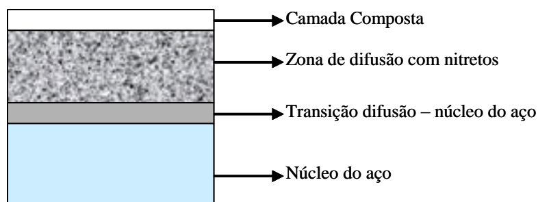
Fig. 2.16: Esquema típico da micro-estrutura de um aço nitretado.
