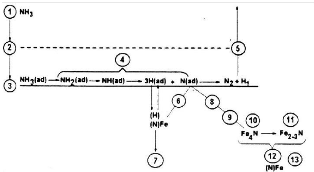
Fig. 2.3: Fenômenos na interface gás/aço durante a nitretação. Fonte Czelusniak (1994).
