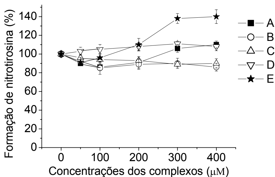
Gráfico 13. Efeito dos complexos como inibidores da nitração do aminoácido tirosina induzida pelo \text{ONOO}^- . Resultados expressos em porcentagem de acordo com os valores da média \pm desvio padrão, em triplicata, de três experimentos diferentes comparados através da máxima formação de NT obtida em relação ao controle positivo.
