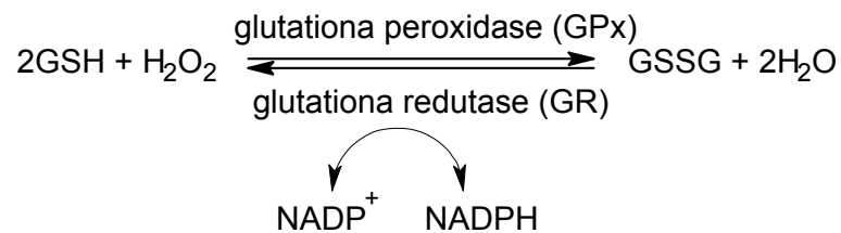
Figura 8. Processo de ciclo redox na atuação indireta das enzimas como antioxidantes.
