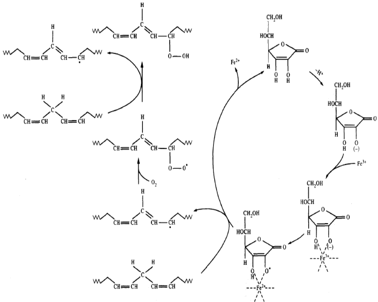
Figura 14. Mecanismo hipotético de iniciação da peroxidação lipídica promovida pela presença de ascorbato e ferro microssomal (adaptado de CASALINO et al., 1996).
