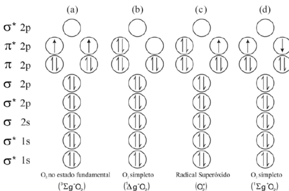
Figura 9. Estados químicos da molécula de dióxigênio ( \text{O}_2 ) (adaptado de HALLIWELL; GUTTERIDGE, 1999; RIBEIRO et al. 2005).
