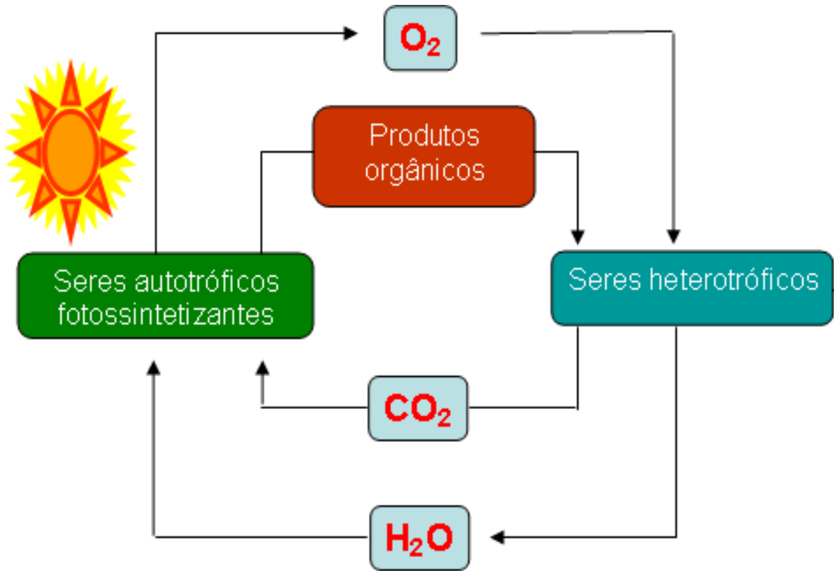
Figura 4. Formas de obtenção de energia e reciclagem do O_2 e CO_2 (adaptado de LEHNINGER, 1986).
