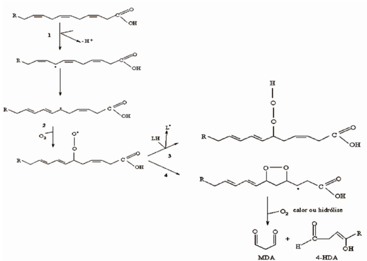
Figura 18. Processo de LPO. Em que: 1: abstração do hidrogênio; 2: reação com oxigênio molecular e formação de radical peroxila; 3: formação de uma espécie radicalar centrada no carbono; e 4: formação de endoperóxido e produtos: MDA: malonildialdeído e 4-HDA: 4-hidróxi-alcenais (adaptado de HALLIWELL; GUTTERIDGE, 1999).
