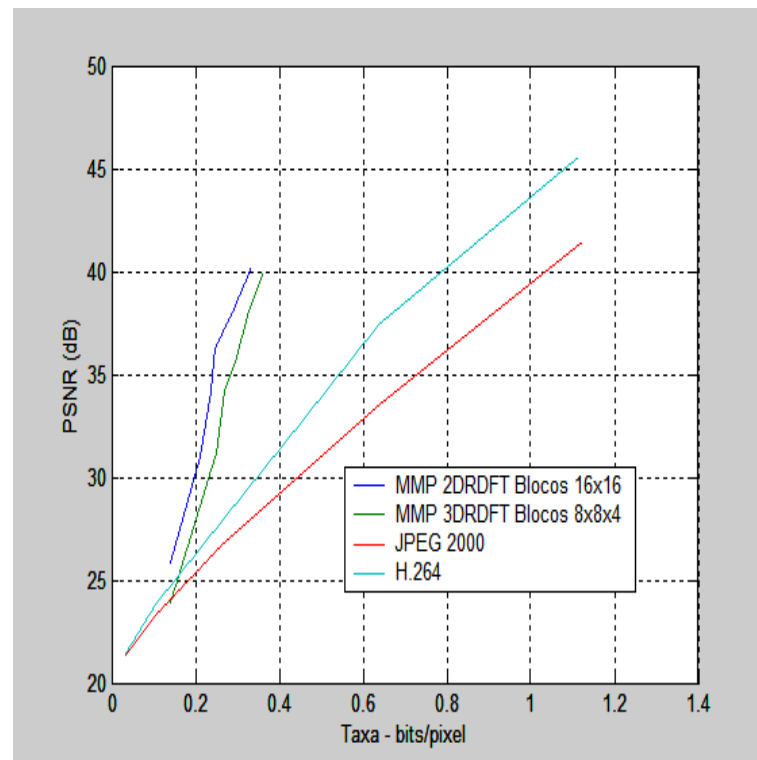
Figura 6.27: Taxa-Distorção para a Comparação do MMP, H.264 e JPEG 2000 para PPI1
