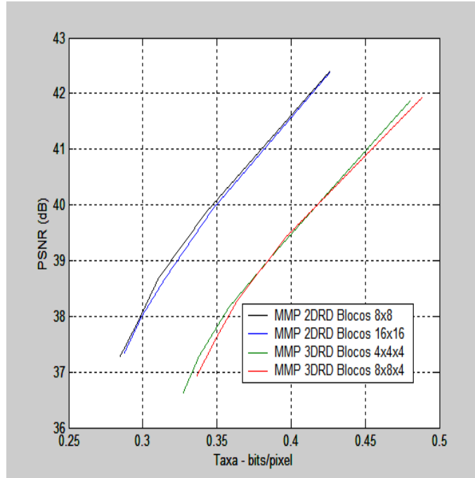
Figura 5.8: Comparação do MMP 3DRD com MMP2DRD para PPI1
