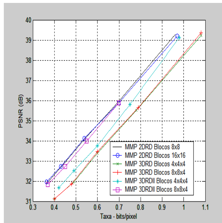
Figura 5.12: Comparação Global para PPI2
