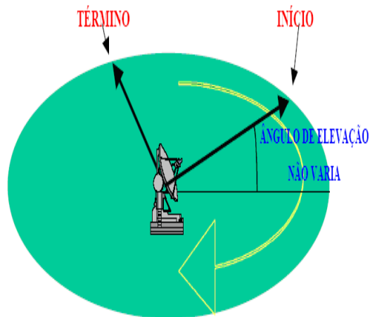
Figura 3.10: Varredura em Azimute
