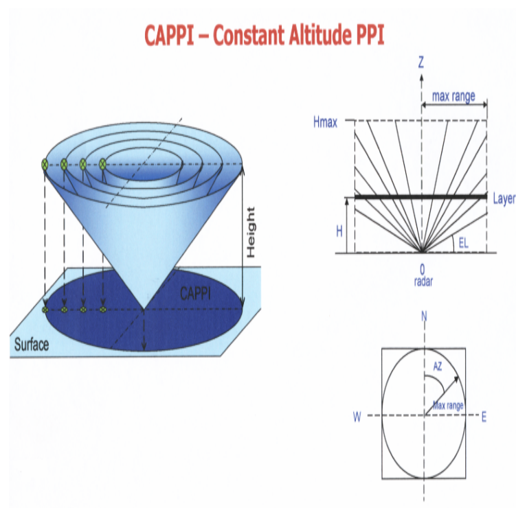
Figura 3.14: Imagem CAPPI
