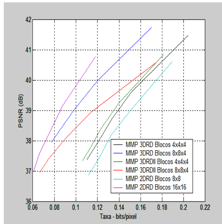
Figura 5.11: Comparação Global para Toy Vehicles
