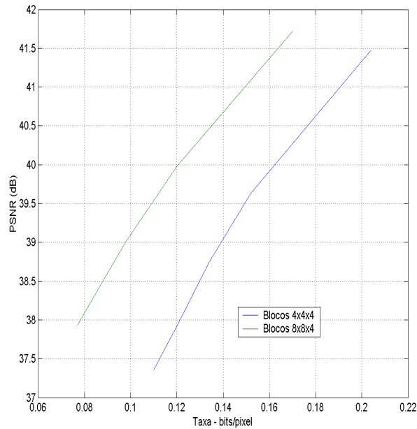
Figura 5.5: Comparação do MMP 3DRD Toy Vehicles com Blocos 8x8x4 e 4x4x4
