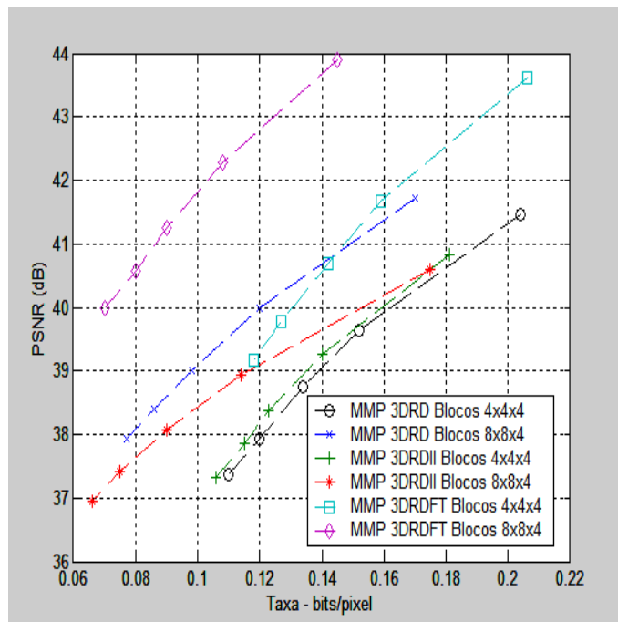
Figura 6.21: Taxa-Distorção para o MMP 3DRD, MMP 3DRDII e MMP 3DRDFT com Toy Vehicles
