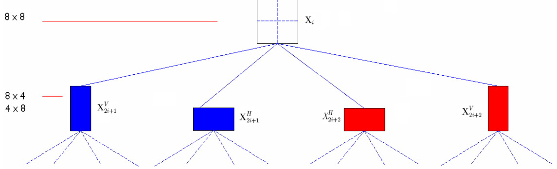
Figura 6.1: Árvore de Segmentação para o MMP 2DRDFT
