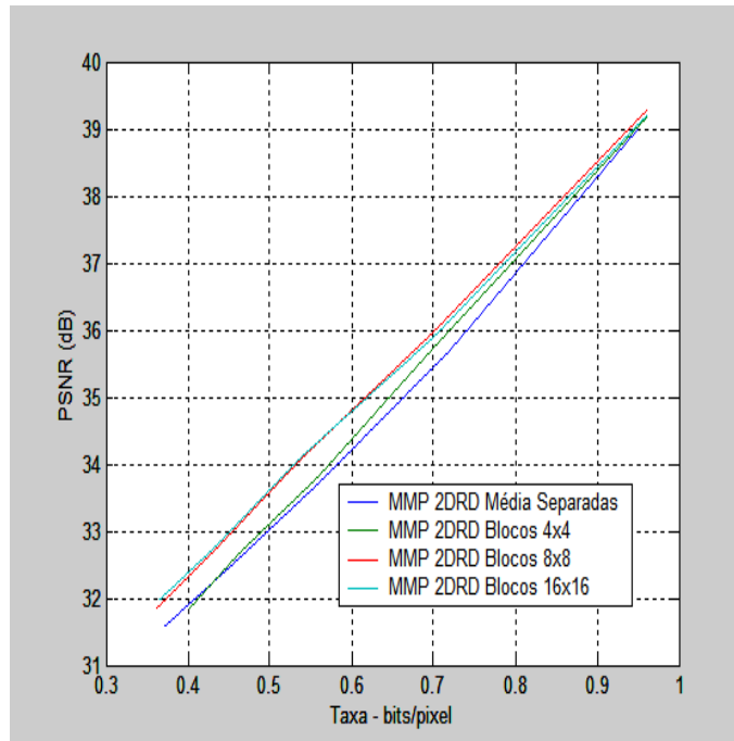
Figura 4.15: Resultados para a Sequência PPI2
