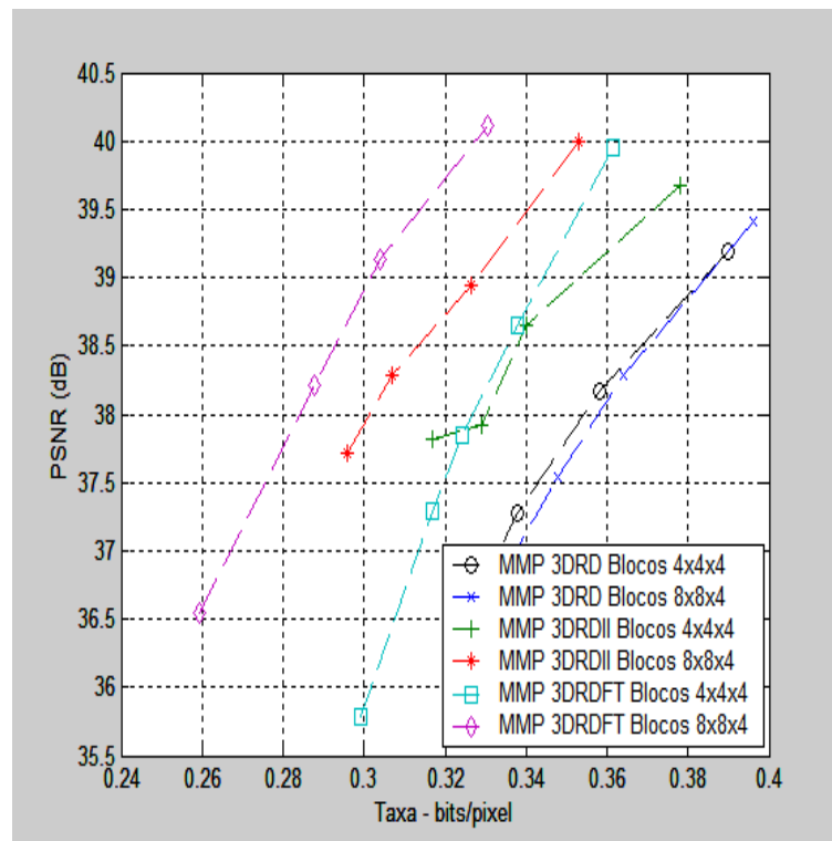
Figura 6.18: Taxa-Distorção para o MMP 3DRD, MMP 3DRDII e MMP 3DRDFT com PPI1
