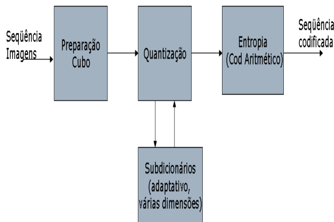
Figura 5.1: Diagrama em Bloco do MMP 3D
