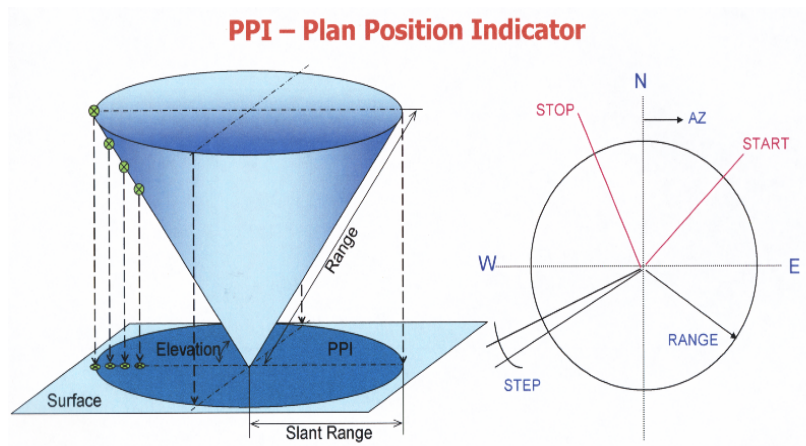
Figura 3.11: Visualização PPI
