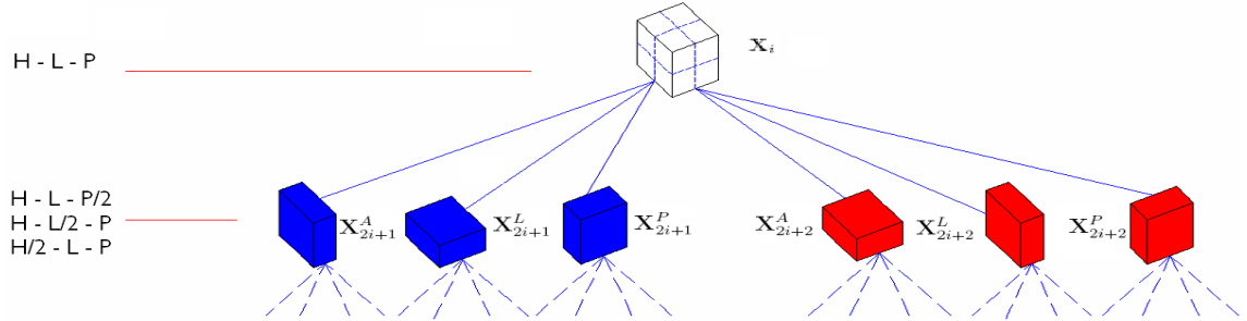
Figura 6.2: Árvore de Segmentação para o MMP 3DRDFT
