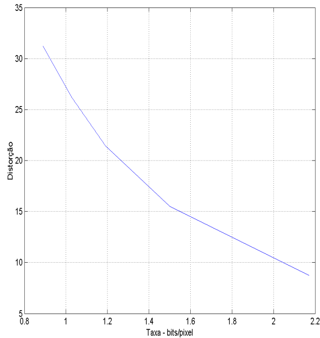
Figura 4.7: D \times R(\text{bit}/s) para a Lena MMP sem Multiescala
