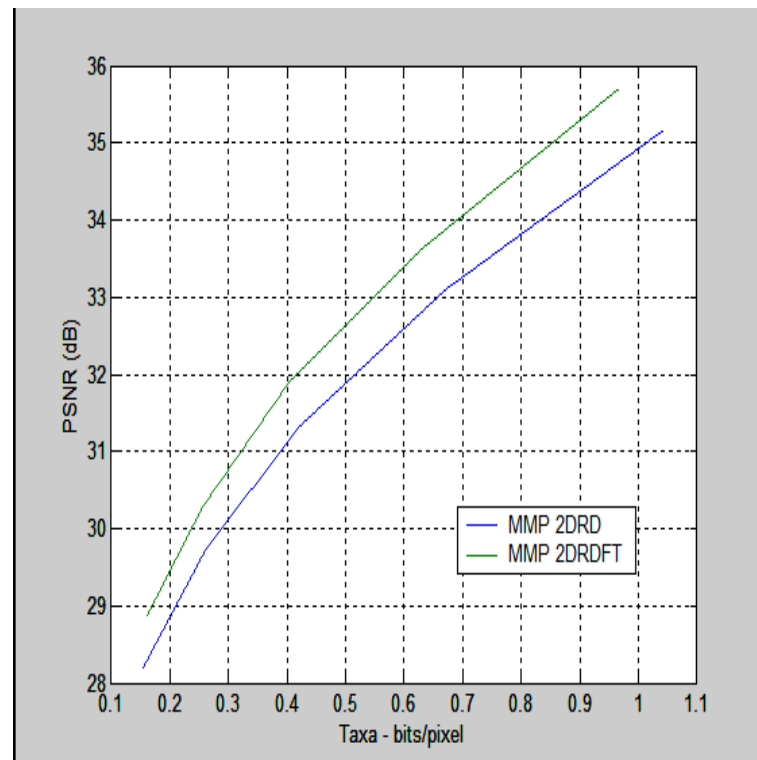
Figura 6.10: Taxa-Distorção para o MMP 2DRD e MMP 2DRDFT com Gold
