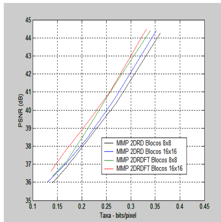
Figura 6.17: Taxa-Distorção para o MMP 2DRD e MMP 2DRDFT com PPI3
