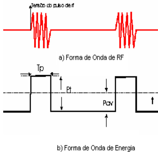
Figura 3.4: Formas de Onda de RF e Energia
