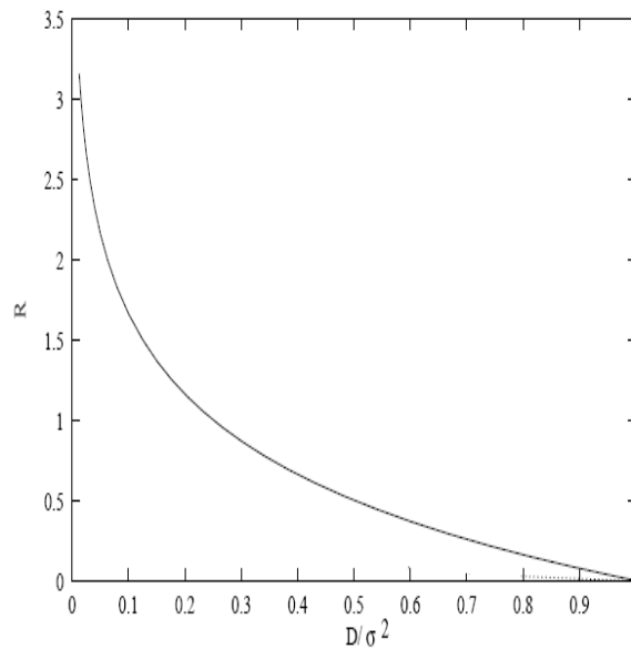
Figura 2.6: Função R(D) da fonte Gaussiana sem memória
