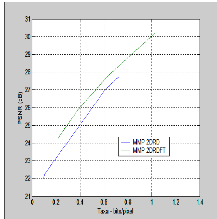
Figura 6.8: Taxa-Distorção para o MMP 2DRD e MMP 2DRDFT com Bridge
