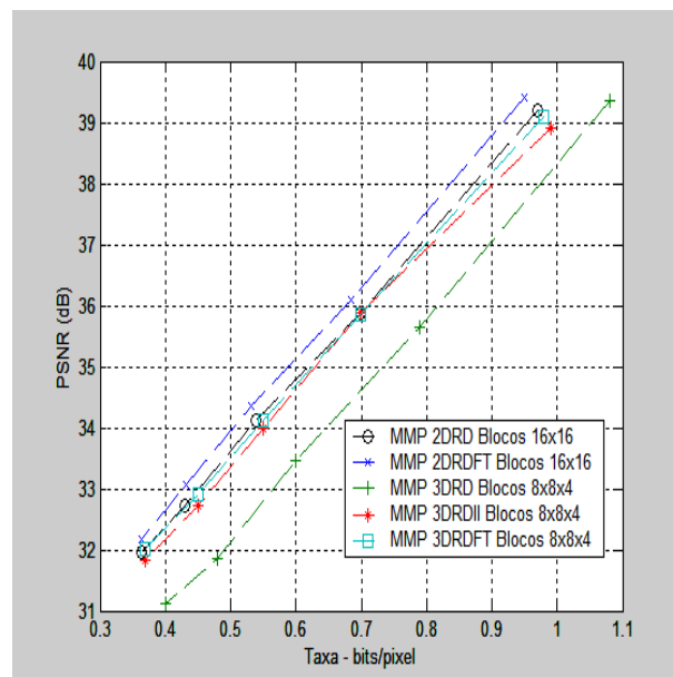
Figura 6.24: Taxa-Distorção para a Comparação dos MMP 2D e MMP 3D para PPI2
