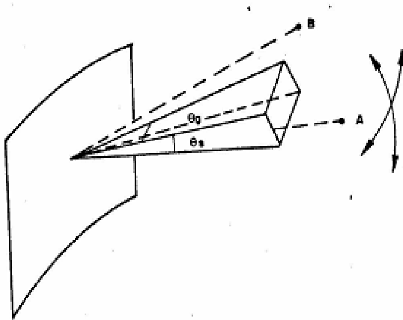
Figura 3.6: Resolução em Azimute
