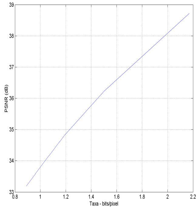
Figura 4.6: PSNR \times Taxa(bit/s) para a Lena MMP sem Multiescala
