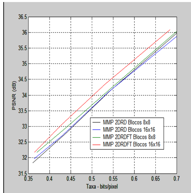
Figura 6.16: Taxa-Distorção para o MMP 2DRD e MMP 2DRDFT com PPI2
