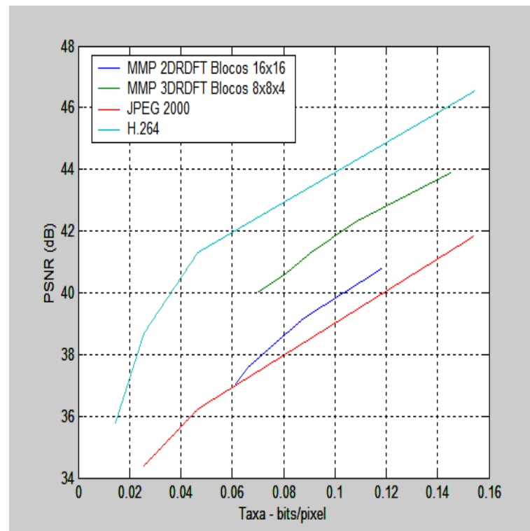
Figura 6.26: Taxa-Distorção para a Comparação do MMP. H.264 e JPEG 2000 para Toy Vehicles
