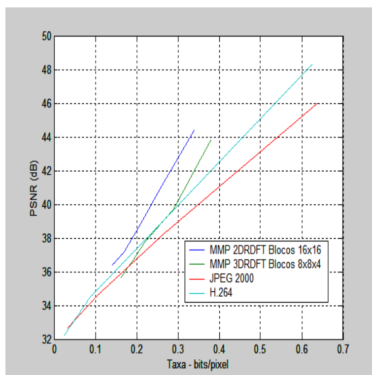
Figura 6.29: Taxa-Distorção para a Comparação do MMP, H.264 e JPEG 2000 para PPI3
