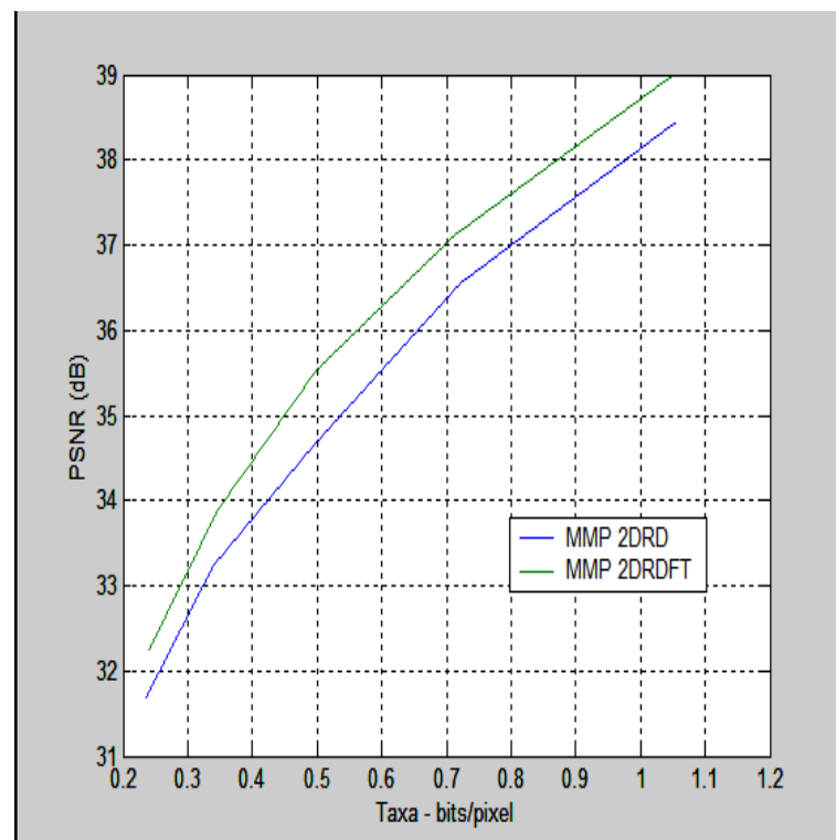
Figura 6.11: Taxa-Distorção para o MMP 2DRD e MMP 2DRDFT com Lena
