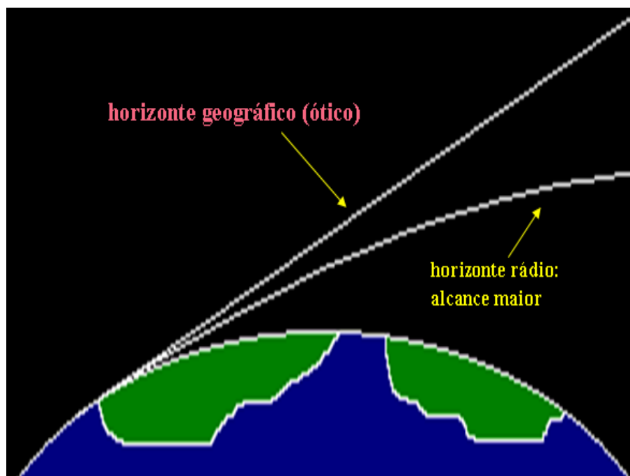
Figura 3.8: Horizonte Radar
