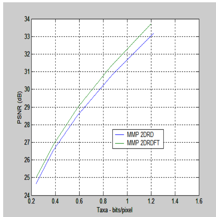
Figura 6.5: Taxa-Distorção para o MMP 2DRD e MMP 2DRDFT com Aerial
