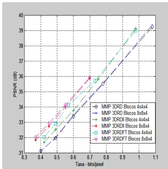
Figura 6.19: Taxa-Distorção para o MMP 3DRD, MMP 3DRDII e MMP 3DRDFT com PPI2
