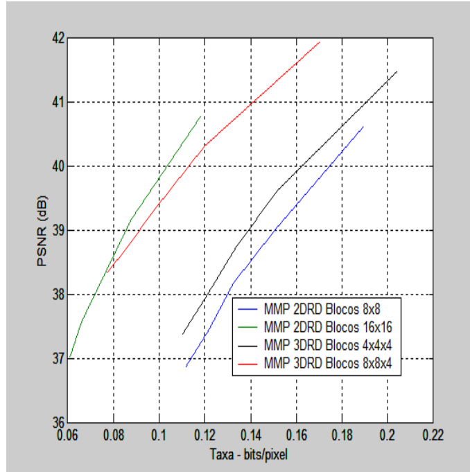
Figura 5.7: Comparação do MMP 3DRD com o MMP2DRD para Toy Vehicles
