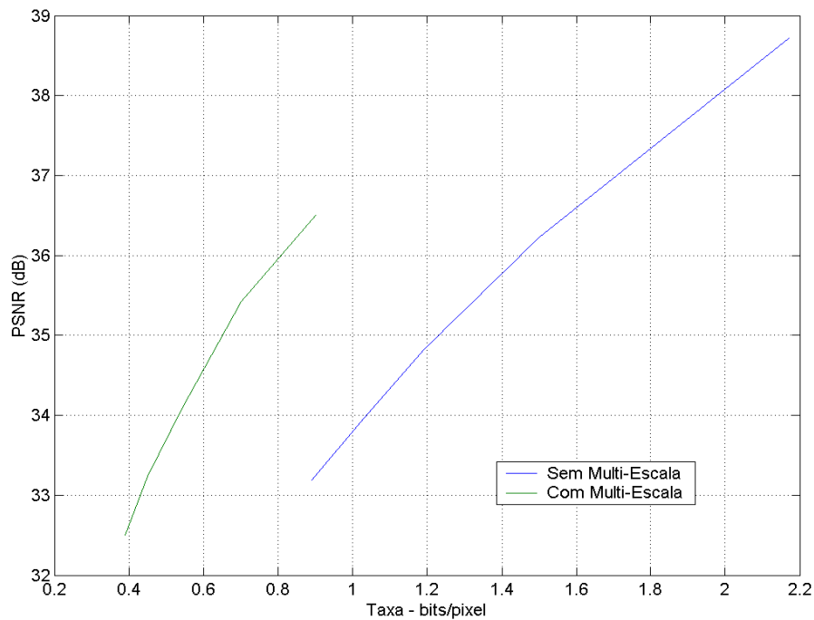
Figura 4.11: Comparação entre Códigos Com e Sem Multiescalas para a Lena
