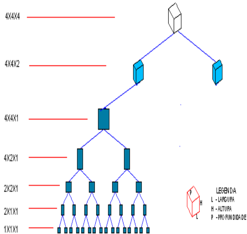
Figura 5.10: Critério de Partição dos Blocos no MMP 3DRDII
