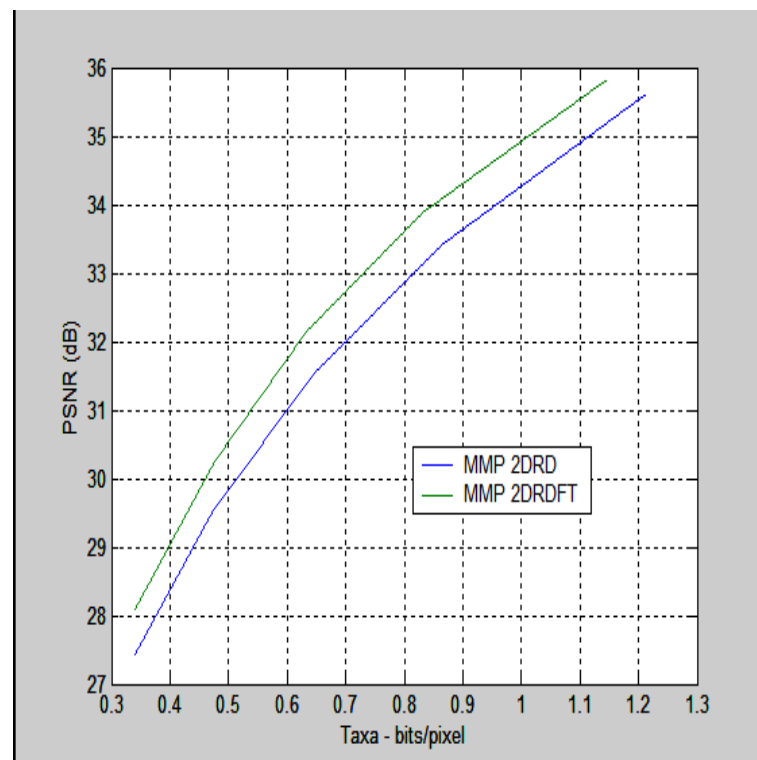
Figura 6.13: Taxa-Distorção para o MMP 2DRD e MMP 2DRDFT com PP1209
