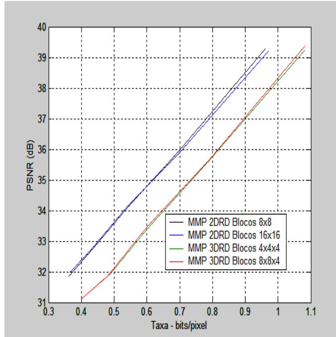
Figura 5.9: Comparação do MMP 3DRD com o MMP2DRD para PPI2
