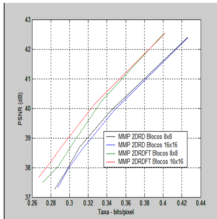
Figura 6.15: Taxa-Distorção para o MMP 2DRD e MMP 2DRDFT com PPI1
