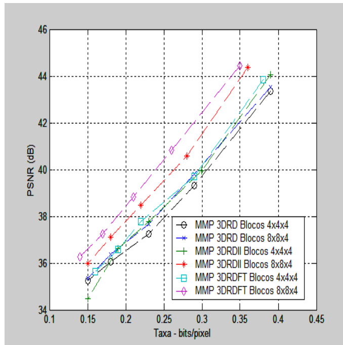
Figura 6.20: Taxa-Distorção para o MMP 3DRD, MMP 3DRDII e MMP 3DRDFT com PPI3
