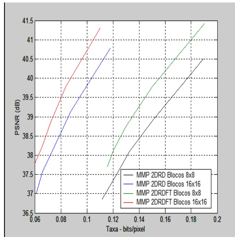
Figura 6.14: Taxa-Distorção para o MMP 2DRD e MMP 2DRDFT com Toy Vehicles
