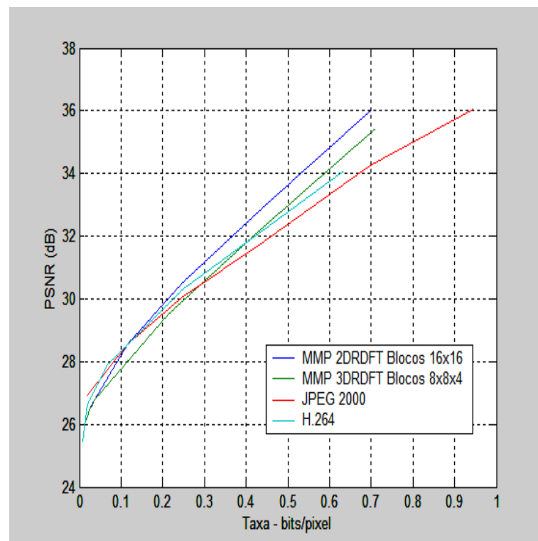
Figura 6.28: Taxa-Distorção para a Comparação do MMP, H.264 e JPEG 2000 para PPI2
