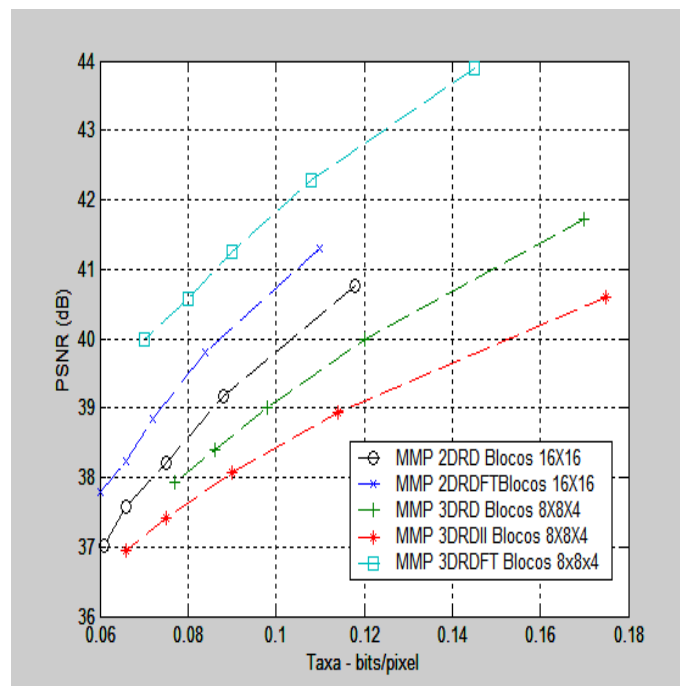
Figura 6.22: Taxa-Distorção para a Comparação dos MMP 2D e MMP 3D para Toy Vehicles
