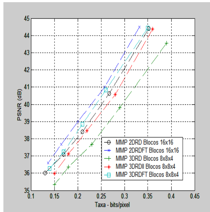
Figura 6.25: Taxa-Distorção para a Comparação dos MMP 2D e MMP 3D para PPI3
