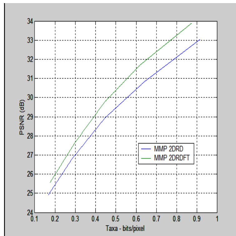
Figura 6.7: Taxa-Distorção para o MMP 2DRD e MMP 2DRDFT com Barbara
