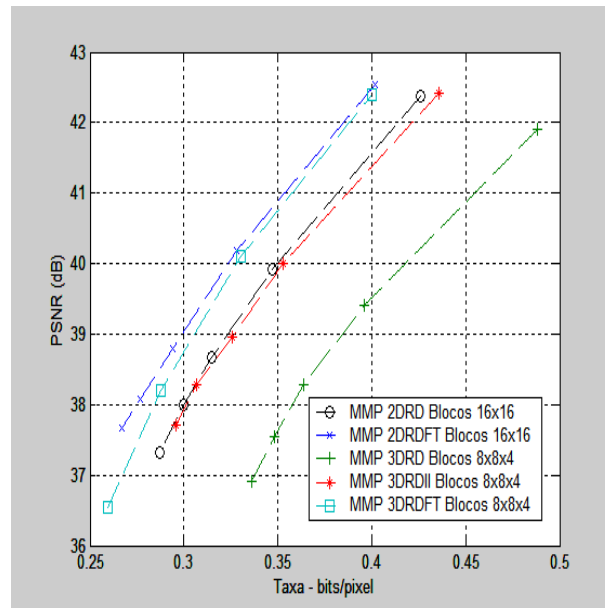
Figura 6.23: Taxa-Distorção para a Comparação dos MMP 2D e MMP 3D para PPI1
