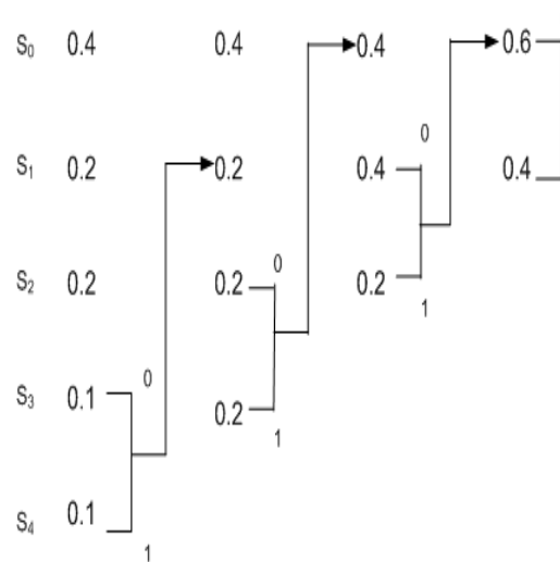
Figura 2.3: Exemplo de Codificação com Huffman
