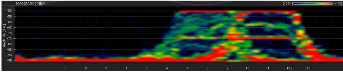
Ilustração 34: Espectro eletromagnético de duas redes utilizando os canais 11 e 8
