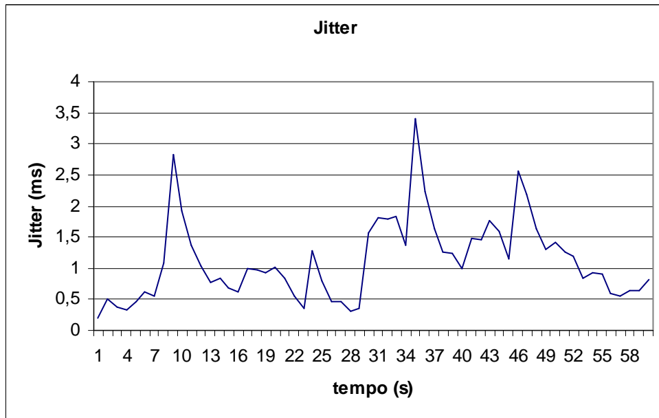
Ilustração 25: Jitter do tráfego UDP com tráfego TCP concorrente e controle de tráfego
