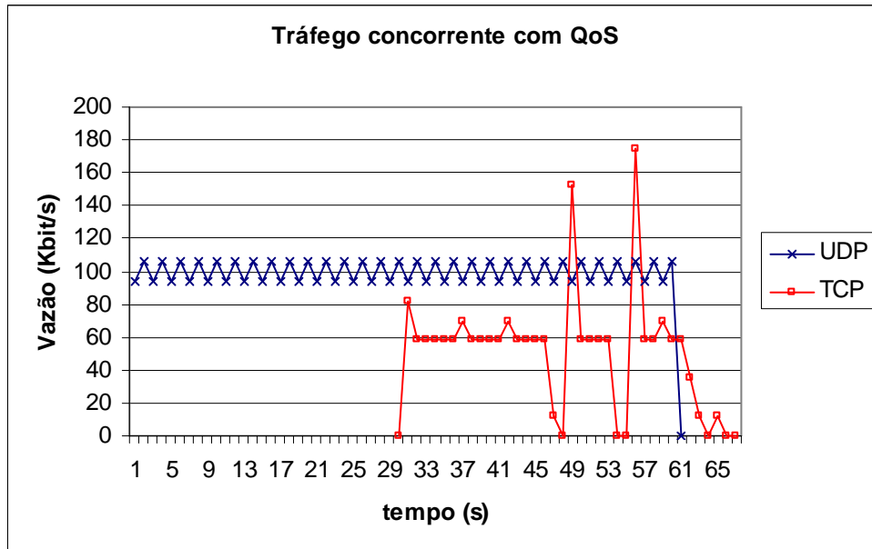
Ilustração 24: Tráfegos UDP e TCP concorrentes com controle de tráfego
