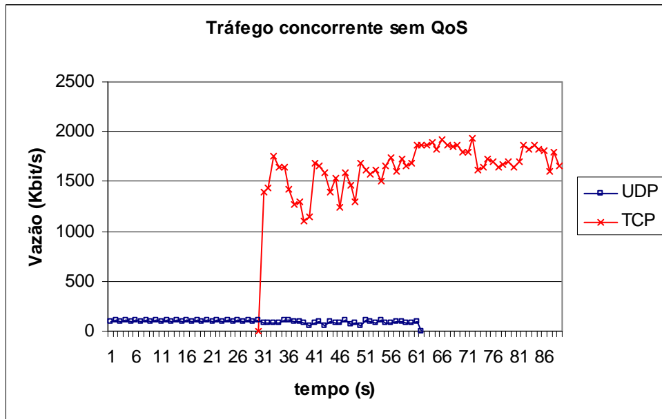
Ilustração 20: Tráfego UDP com tráfego TCP concorrente
