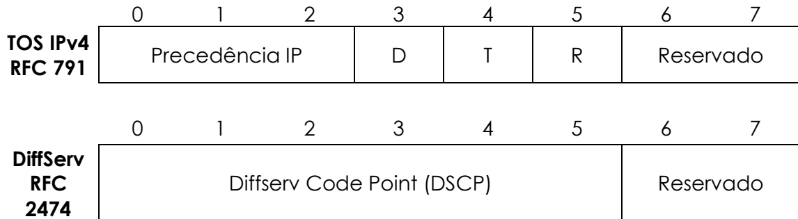
Ilustração 13: Campos TOS e DSCP no IPv4
