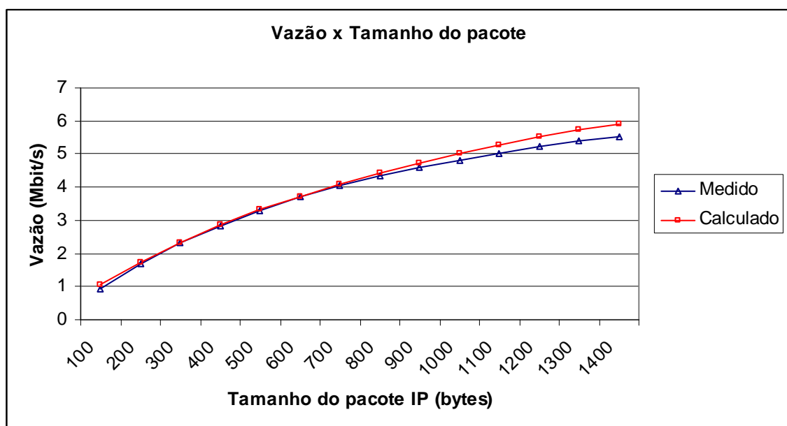
Ilustração 17: Vazão máxima em função do payload
