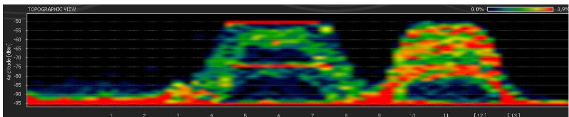
Ilustração 32: Espectro eletromagnético de duas redes utilizando os canais 11 e 6
