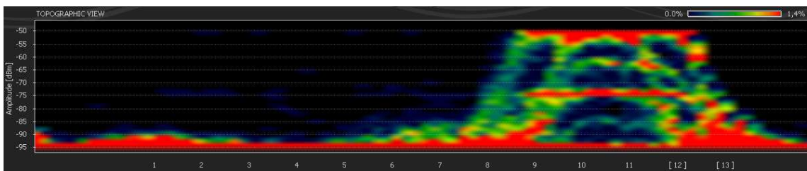
Ilustração 36: Espectro eletromagnético de duas redes utilizando o canal 11
