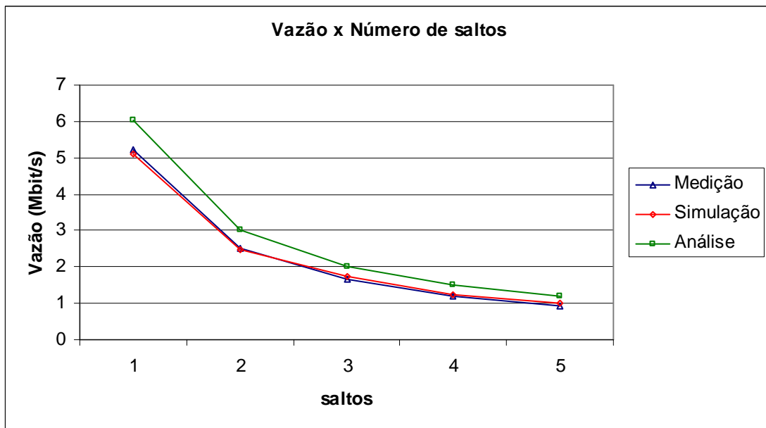
Ilustração 18: Capacidade máxima de banda por saltos – pacotes de 1470 Bytes
