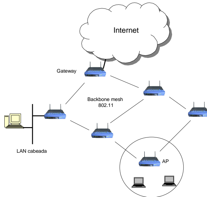
Ilustração 3: Diagrama de uma rede em malha
