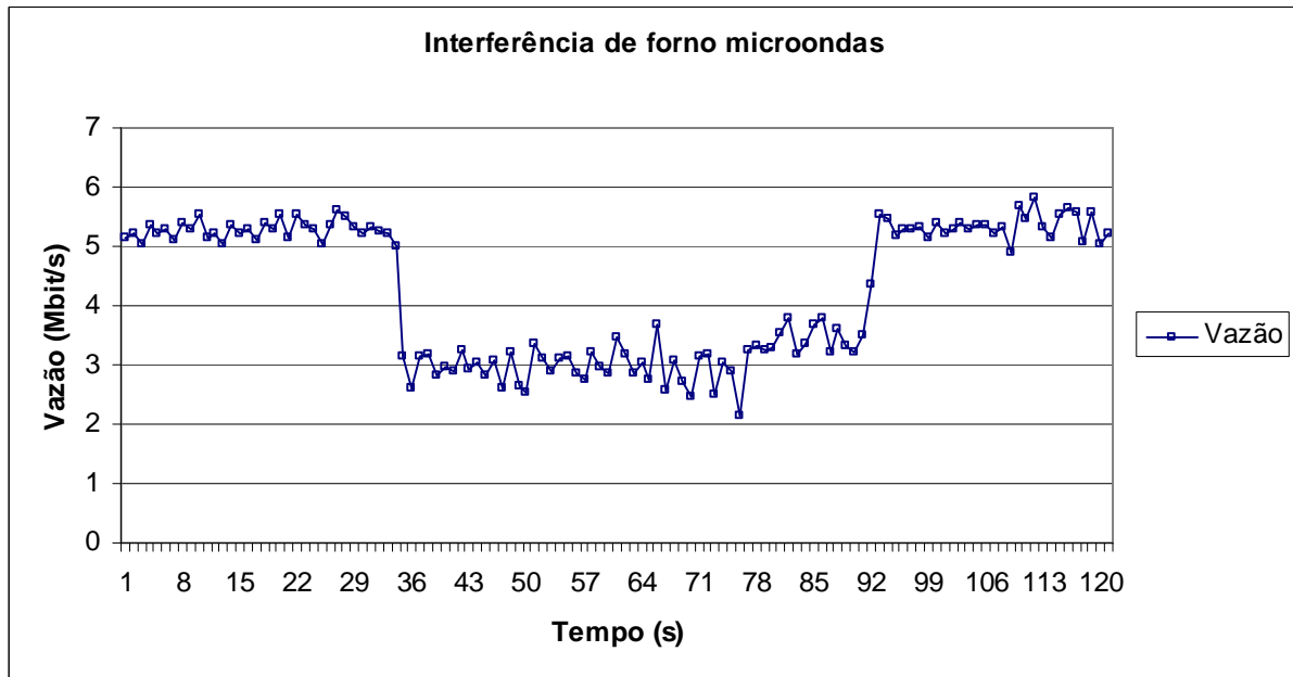
Ilustração 7: Interferência gerada por forno microondas em transmissão de dados
