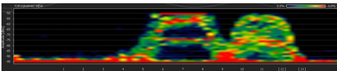
Ilustração 33: Espectro eletromagnético de duas redes utilizando os canais 11 e 7
