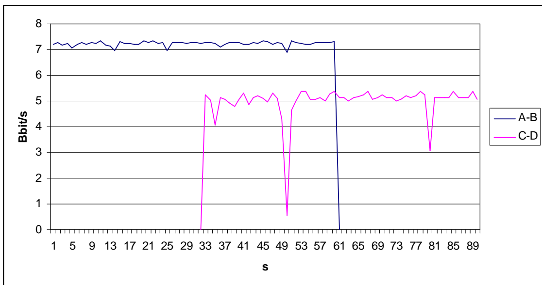
Ilustração 26: Transmissão de duas redes nos canais 11 e 6
