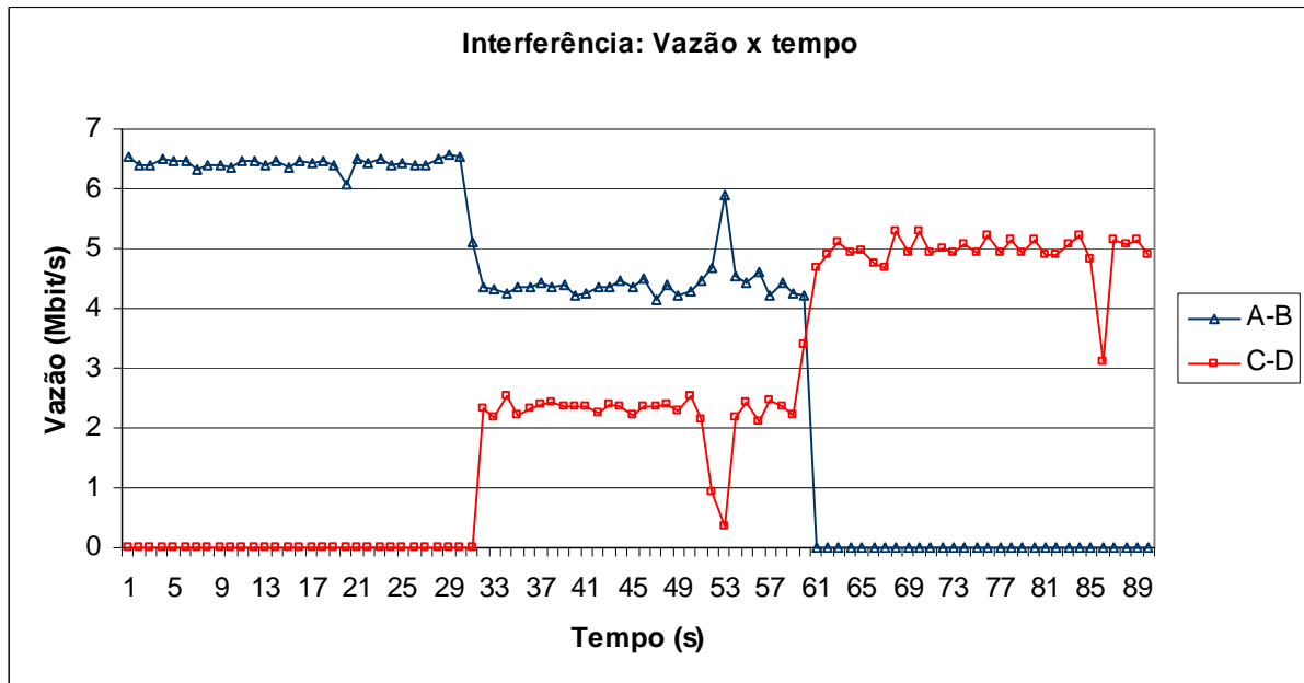
Ilustração 6: Exemplo de interferência de outro sistema
