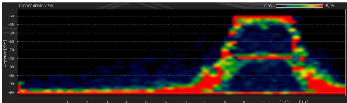
Ilustração 10: Transmissão de dados sofrendo interferência de um forno microondas
