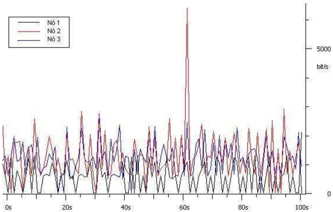
Ilustração 23: Perfil de tráfego do OLSR
