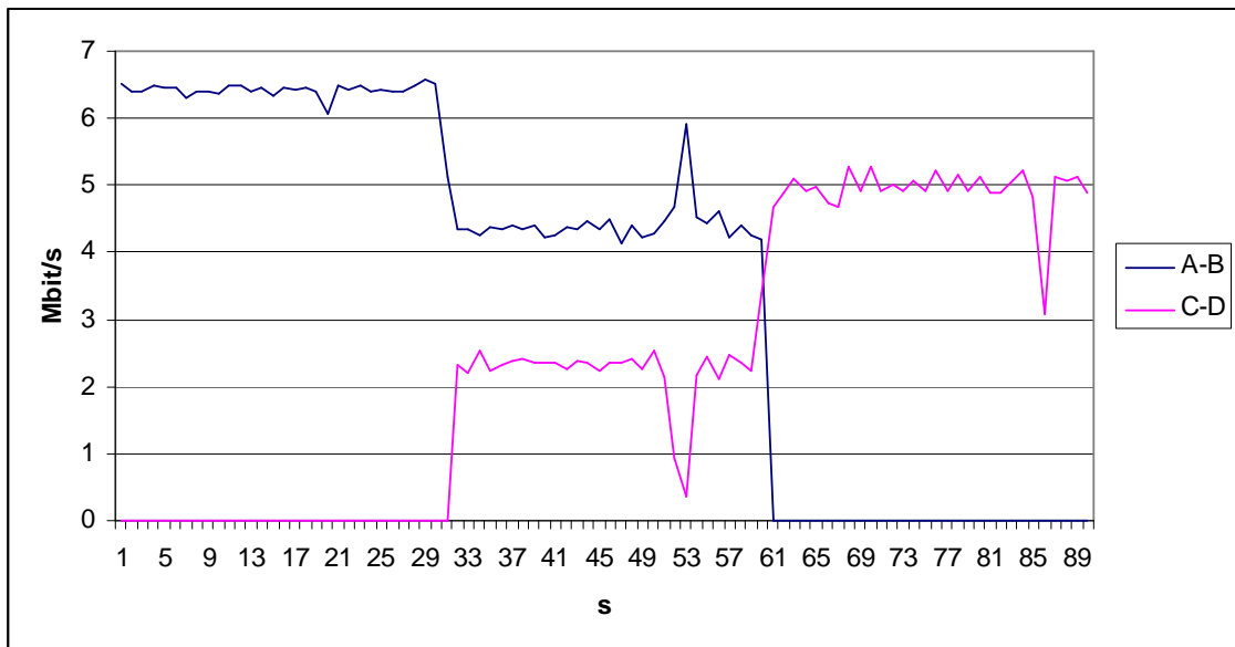
Ilustração 31: Transmissão de duas redes no canal 11
