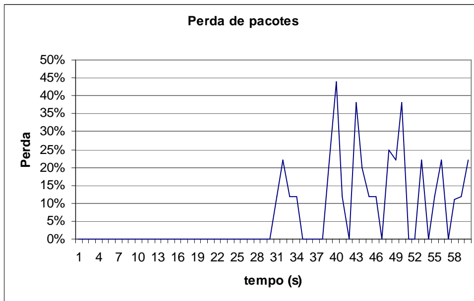
Ilustração 22: Valores de perda de pacotes UDP com tráfego TCP concorrente
