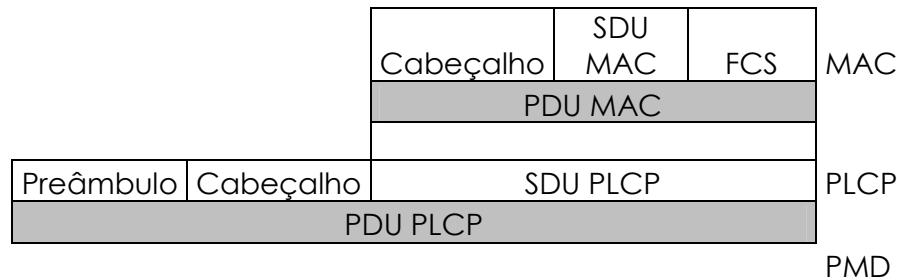
Ilustração 1: Cabeçalhos das diferentes camadas do 802.11
