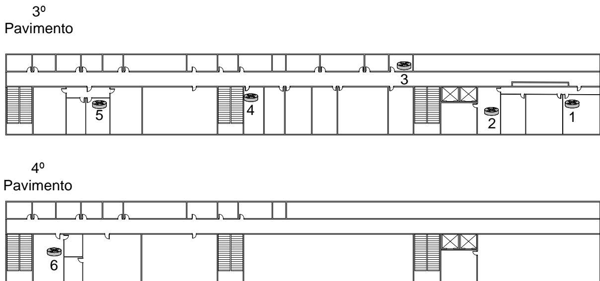
Ilustração 15: Planta baixa dos pavimentos do prédio de Engenharia da UFF
