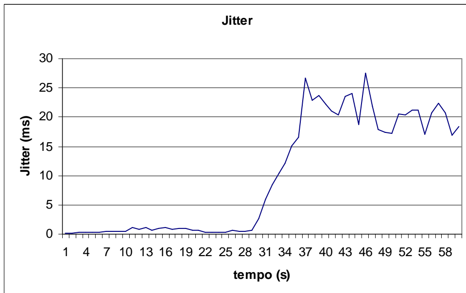
Ilustração 21: Valores de jitter do tráfego UDP com tráfego TCP concorrente
