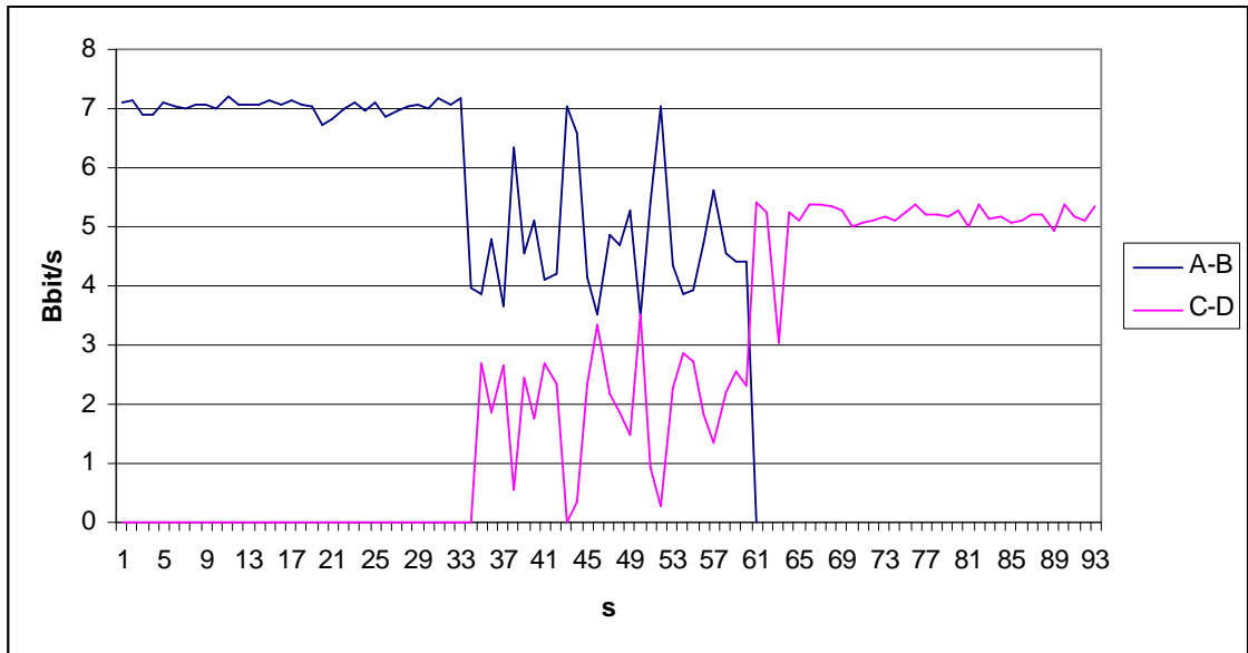
Ilustração 29: Transmissão de duas redes nos canais 11 e 9
