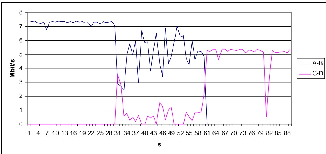
Ilustração 30: Transmissão de duas redes nos canais 11 e 10
