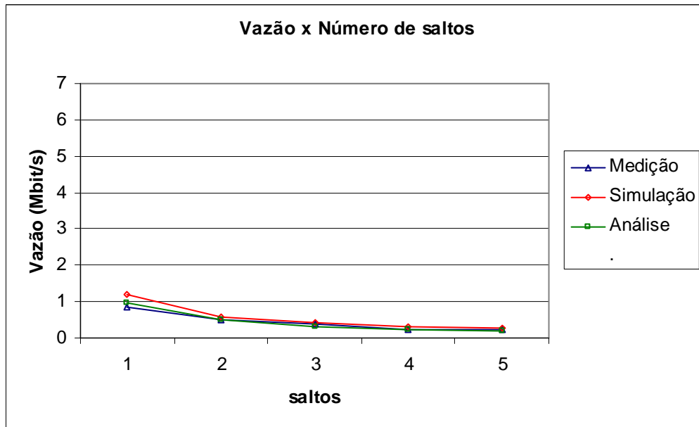
Ilustração 19: Capacidade máxima de banda por saltos – pacotes de 100 Bytes
