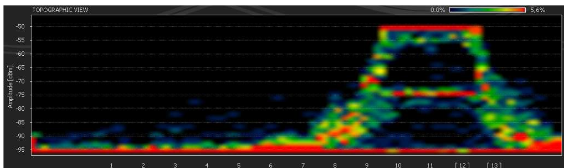
Ilustração 8: Espectro eletromagnético durante uma transmissão sem interferência
