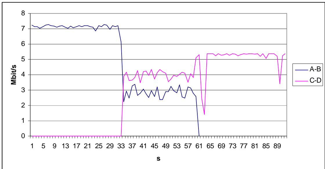
Ilustração 28: Transmissão de duas redes nos canais 11 e 8
