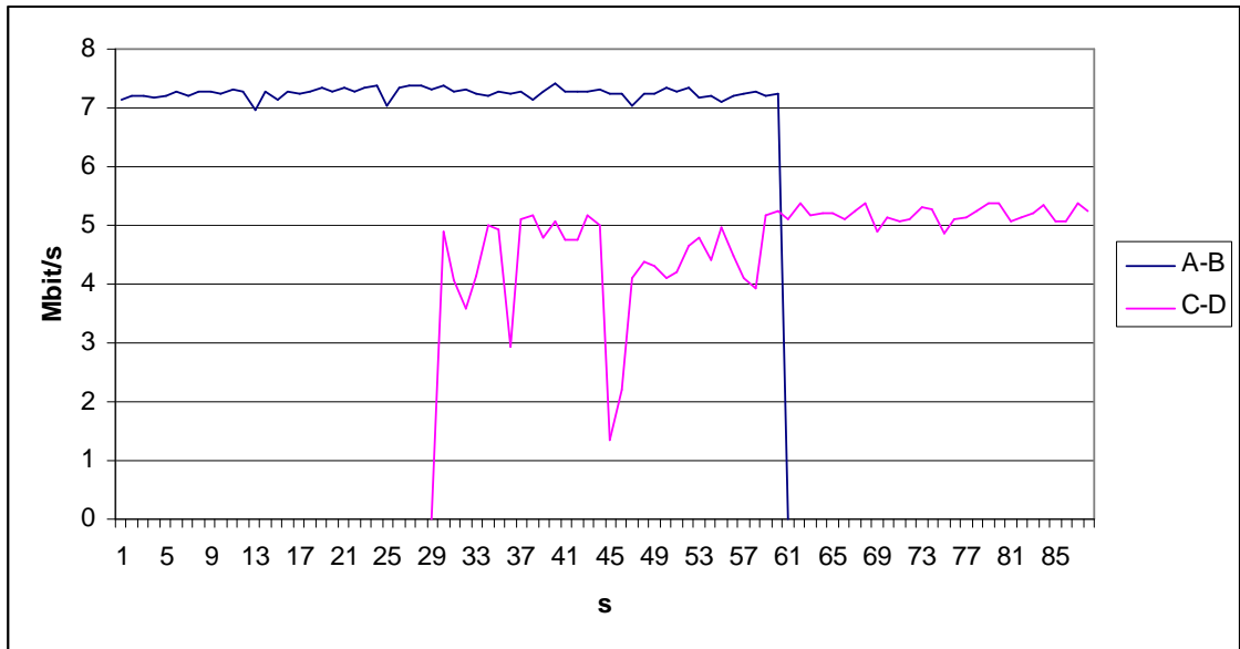
Ilustração 27: Transmissão de duas redes nos canais 11 e 7
