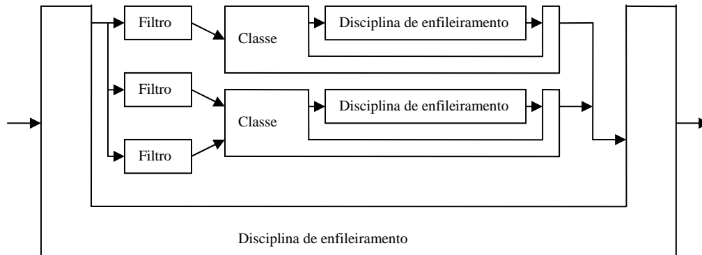
Ilustração 14: Um modelo simples de disciplina de enfileiramento no Linux
