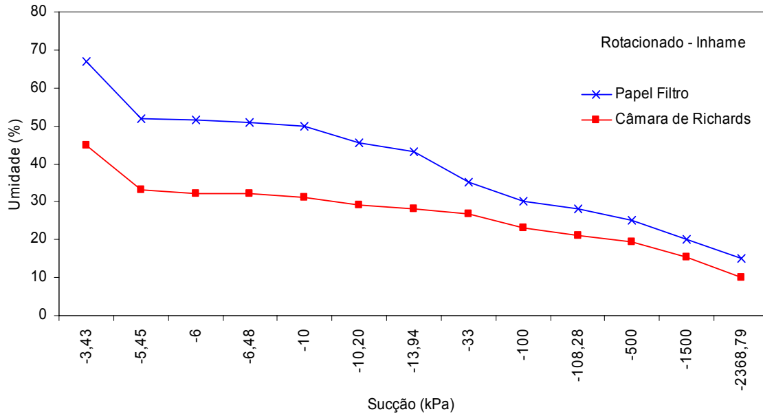
Figura 4.46. Comportamento sucção x umidade na amostra da parcela sob cultivo rotacionado - inhame, obtidos pelos métodos do papel filtro e da câmara de pressão de Richards.
