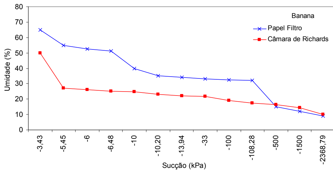
Figura 4.45. Comportamento sucção x umidade na amostra da parcela sob cultivo de banana, obtidos pelos métodos do papel filtro e da câmara de pressão de Richards.
