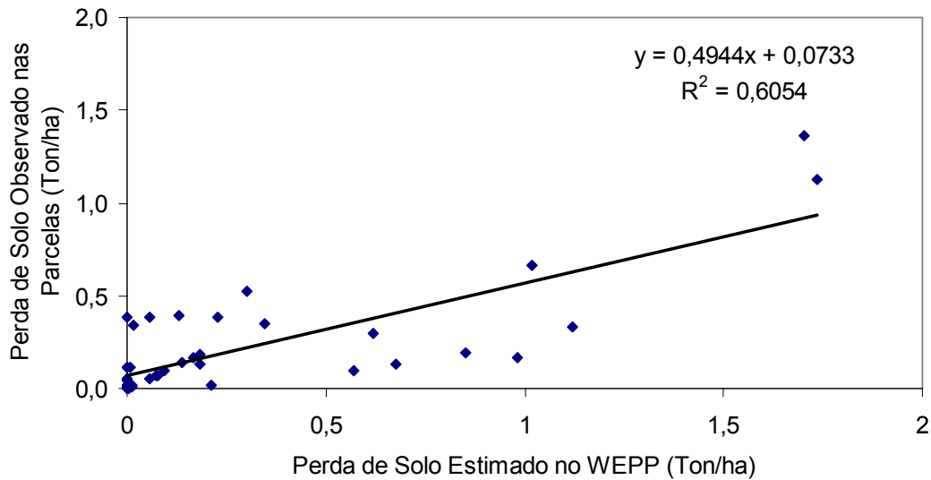
Figura 4.38. Valores de perdas de solo obtidas em campo e simuladas pelo WEPP, decorrentes de eventos isolados de precipitação.
