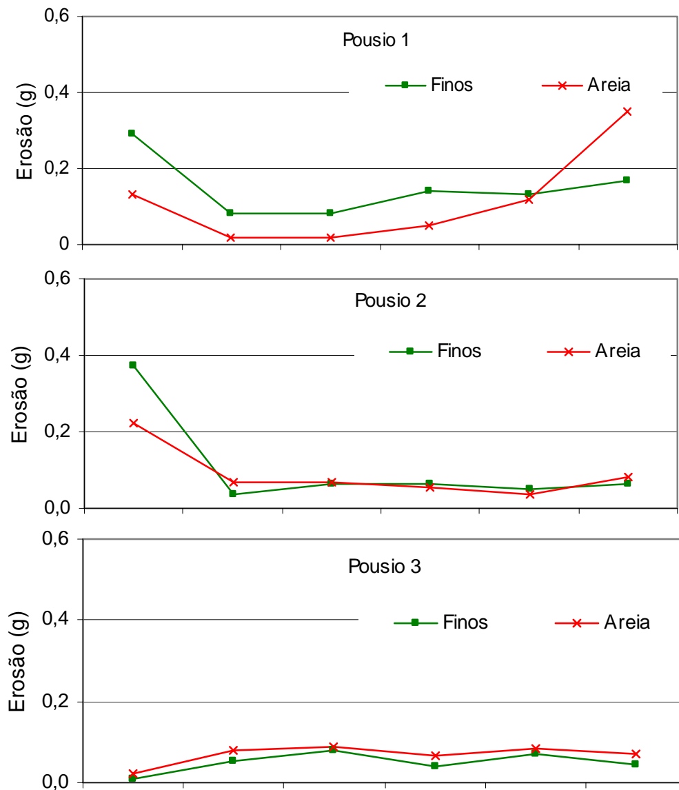
Figura A6. Perdas de solo por meio do ensaio de Inberbitizen com amostras de 70 cm 2 retiradas na parcela em pousio florestal de 2 a 3 anos.
