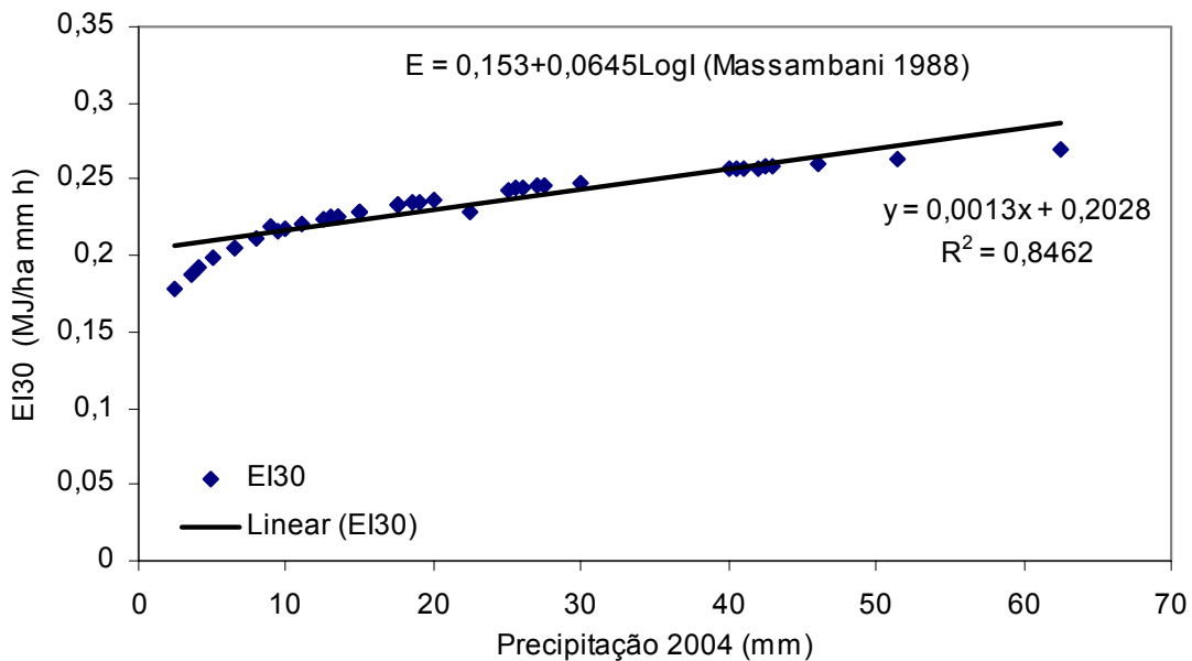
Gráfico 3.2. Cálculo do EI a partir dos dados pluviométricos (modelo de Massambani 1988, para dados de pluviógrafos).
