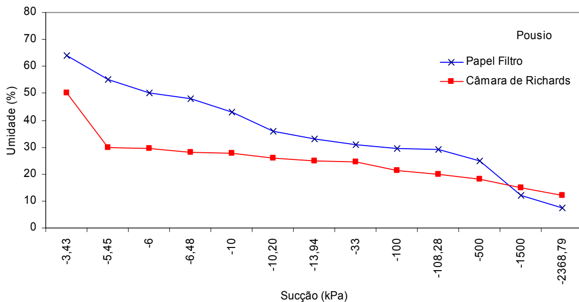
Figura 4.47. Comportamento sucção x umidade na amostra da parcela sob pousio florestal recente, obtidos pelos métodos do papel filtro e da câmara de pressão de Richards.
