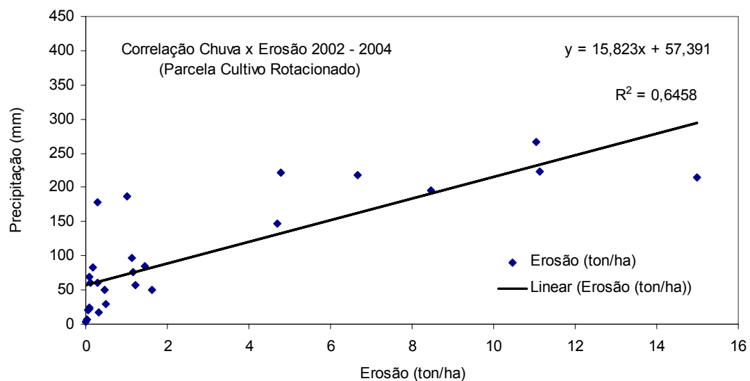
Figura 4.35a. Correlações chuva x erosão no período de 2002 a 2004 para parcela sob cultivo rotacionado.
