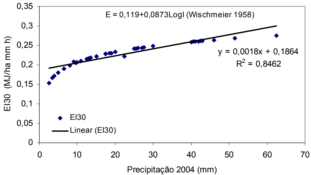
Gráfico 3.1. Cálculo do EI a partir dos dados pluviométricos (modelo de Wischmeier 1958, para dados de pluviógrafos).
