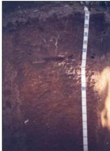
Figura 2.7. Perfil do solo da encosta onde foram montadas as parcelas de perdas de solo.
