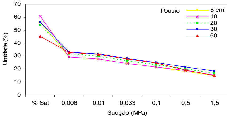
Figura 4.13. Curva característica de retenção de umidade obtida em laboratório – câmara sob pousio, pela panela de pressão de Richards (CNPS – Embrapa).
