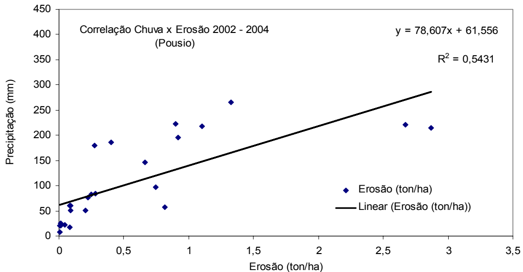
Figura 4.36a. Correlações chuva x erosão no período de 2002 a 2004 para parcela sob pousio florestal recente.
