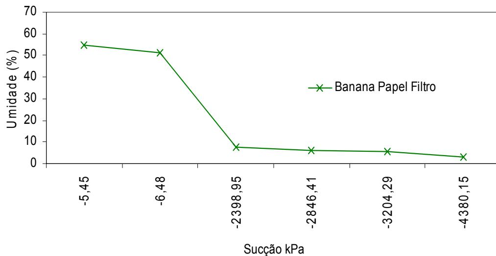
Figura 4.42. Curva característica sucção x umidade para o solo da parcela sob cultivo de banana, obtido pelo método do papel filtro – Bom Jardim, RJ.
