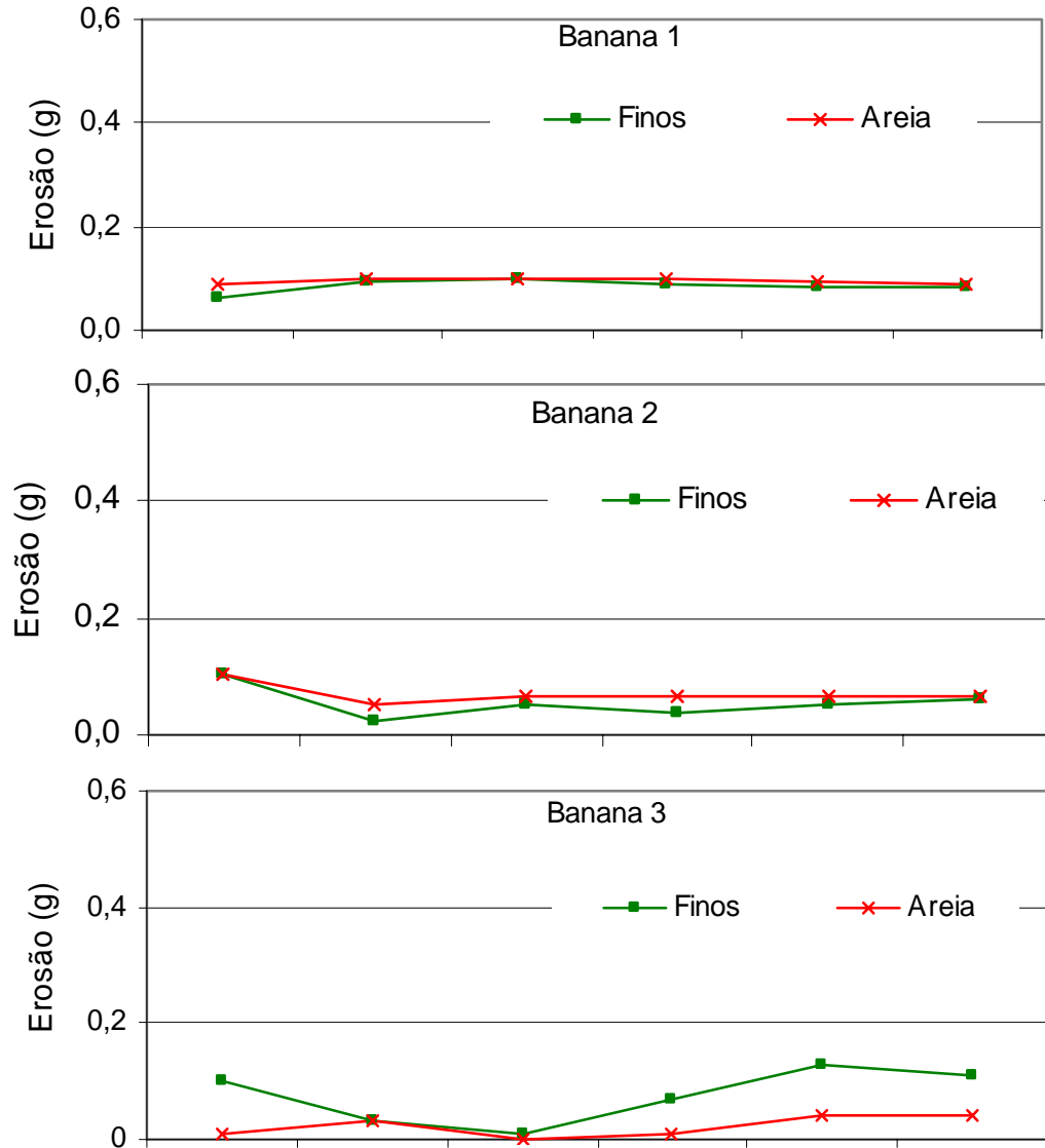
Figura A5. Perdas de solo por meio do ensaio de Inberbitizen com amostras de 70 cm 2 retiradas na parcela sob cultivo de banana.
