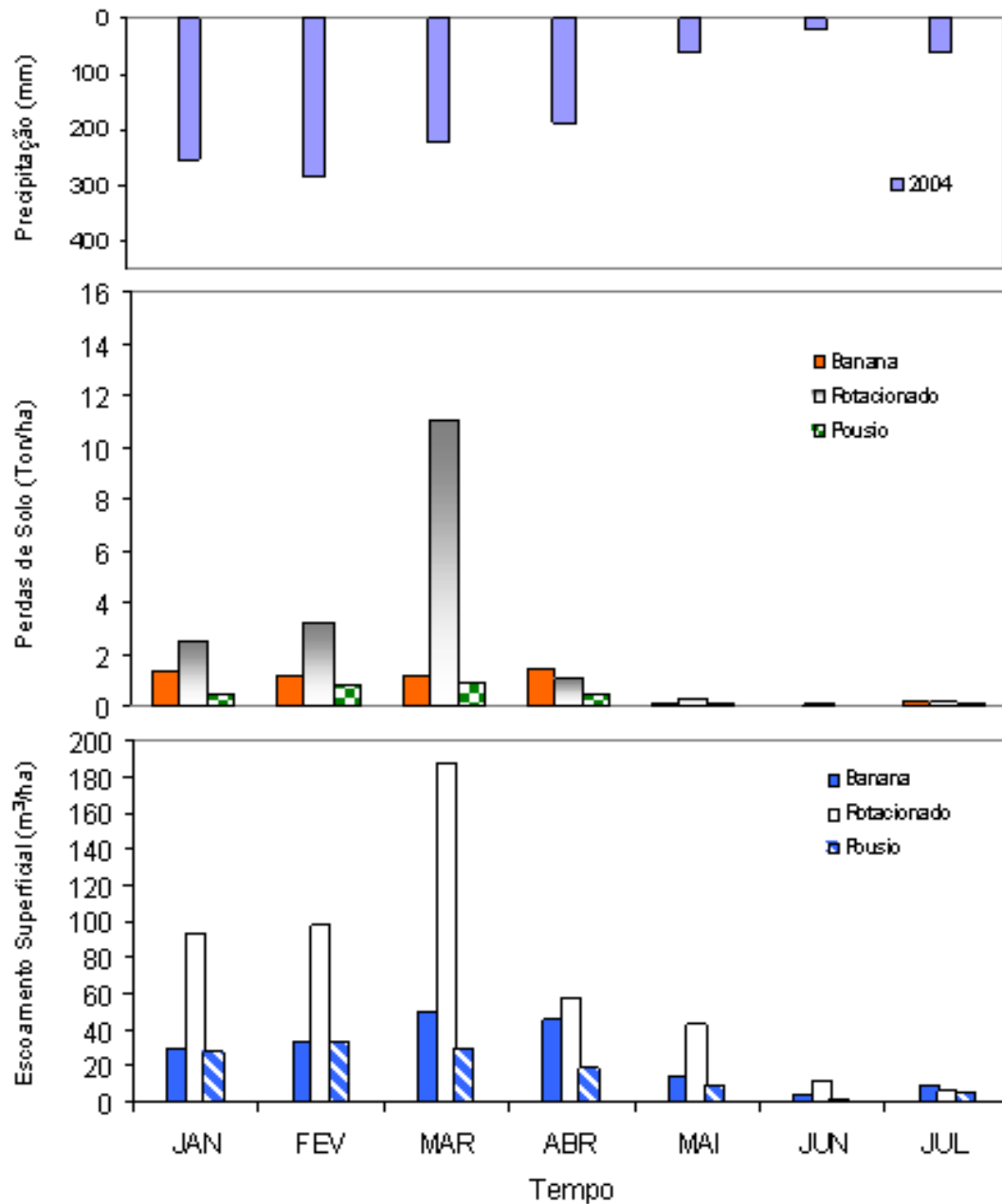
Figura 4.33. Comportamento do escoamento superficial e das perdas de solo sob diferentes coberturas vegetais, em relação à distribuição das chuvas ocorridas no ano de 2004.
