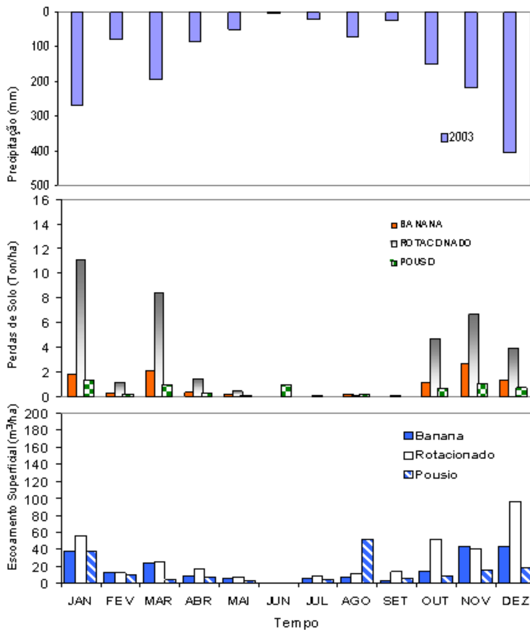
Figura 4.32. Comportamento do escoamento superficial e das perdas de solo sob diferentes coberturas vegetais, em relação à distribuição das chuvas ocorridas no ano de 2003.
