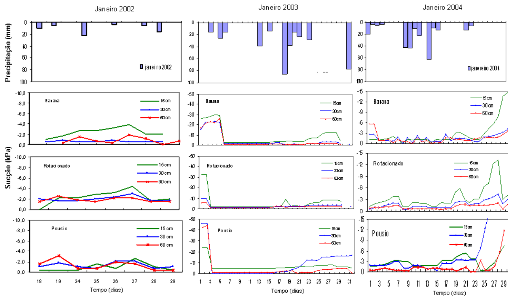
Figura 4.17. Distribuição das succões (Potenciais Matriciais) em kPa nas parcelas sob diferentes coberturas vegetais, em relação aos eventos de precipitação ao longo do tempo (meses de Janeiro de 2002, 2003 e 2004).
