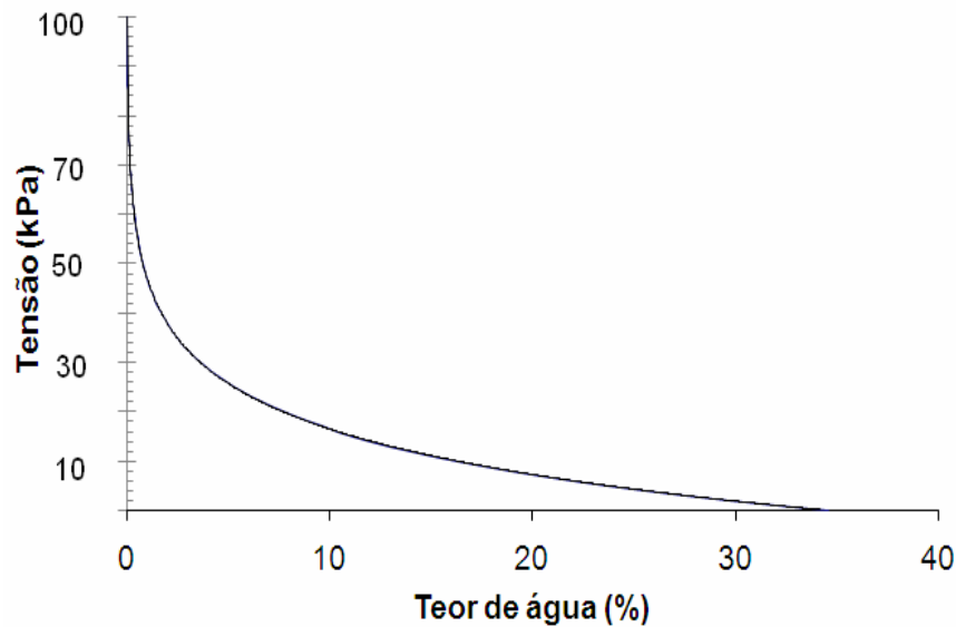
Figura 1: Curva de retenção de água de um solo LVE distrófico textura média e a relação entre a tensão (expressa em bar) e o teor de água no solo (%).
