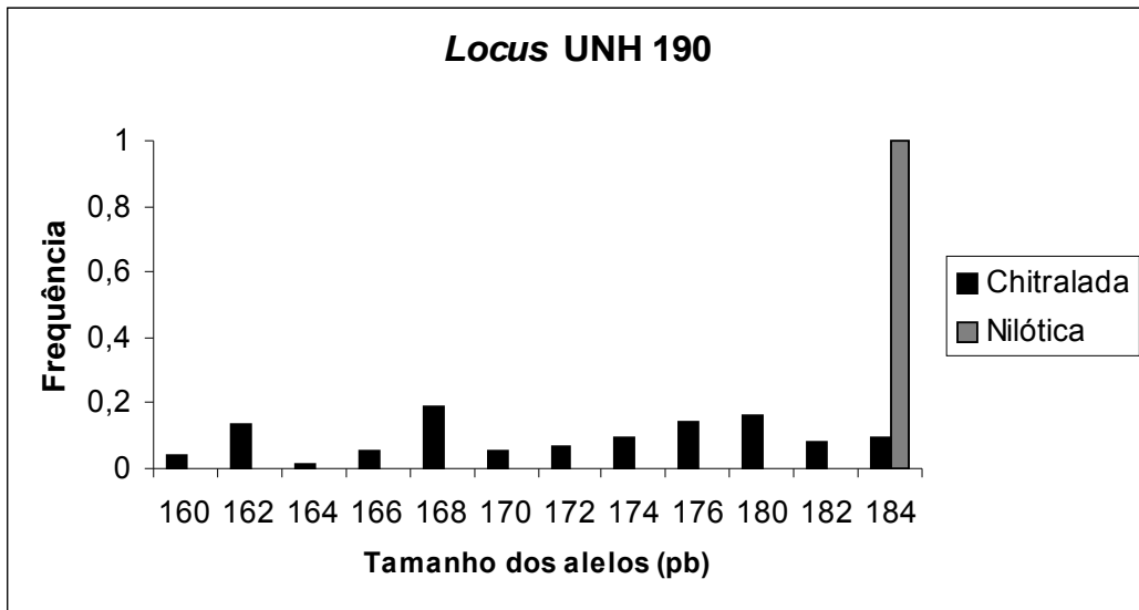
Figura 3. Histograma das frequências dos alelos para o locus UNH 190.
