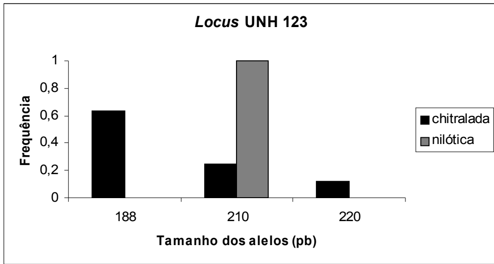
Figura 1. Histograma das frequências dos alelos para o locus UNH 123.
