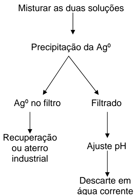
Figura 35-Esquema do tratamento de descontaminação de solução de nitrato de prata.
