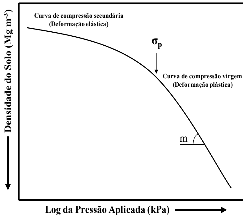
FIGURA 1 Curva de compressão do solo mostrando a curva de compressão secundária, curva de compressão virgem, a pressão de preconsolidação ( \sigma_p ) e o índice de compressão ( m ). Adaptado de Dias Júnior (1994).
