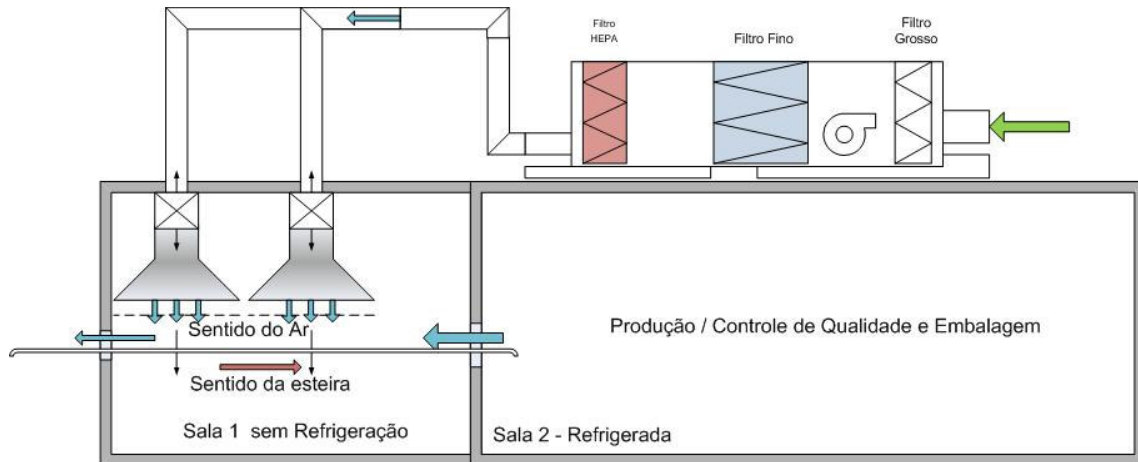
Figura 17: Corte com a apresentação do fluxo de ar para a sala 1 – UTA -2
