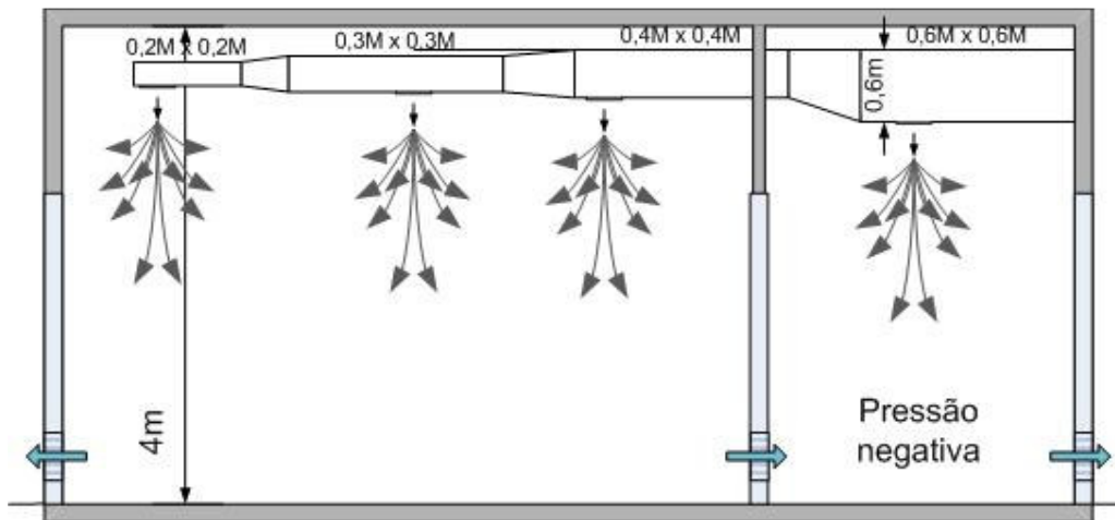
Figura 11: Sala com fluxo de ar turbulento
