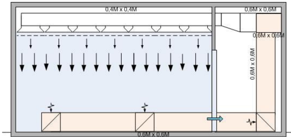
Figura 13: Sala com fluxo unidirecional ou laminar com retorno
