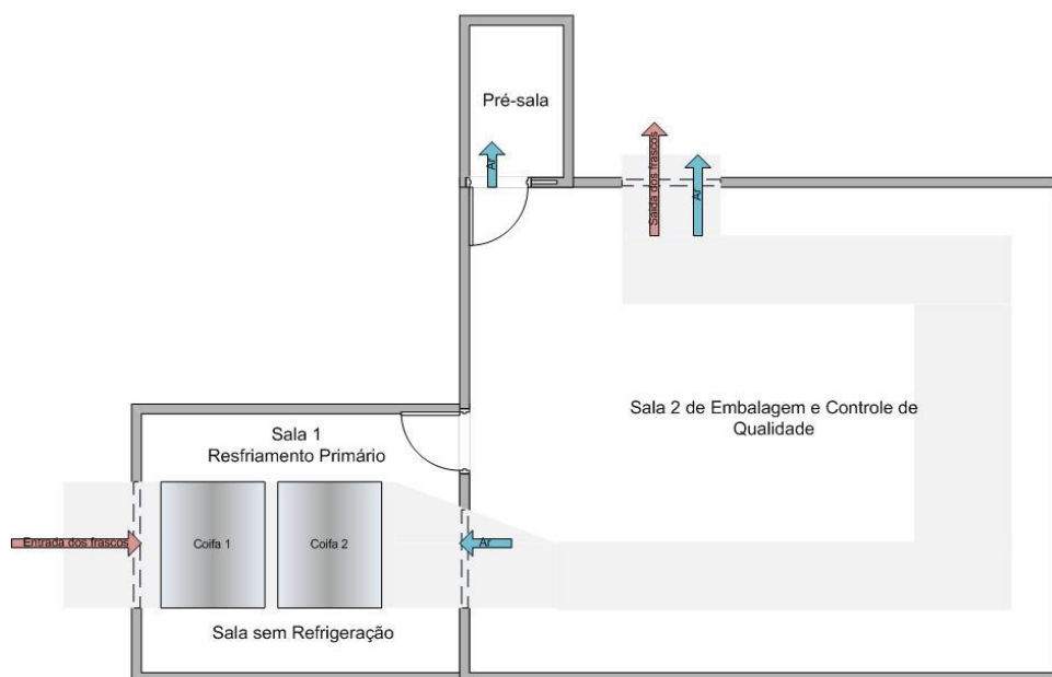
Figura 16: Planta baixa do conjunto linha 2
