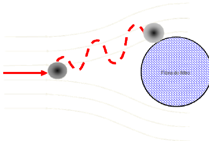
Figura 9: Trajetória pelo mecanismo de difusão browniana.
