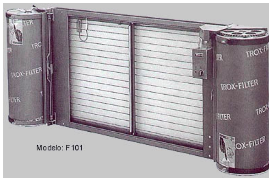
Figura 6: Filtro com renovação automática. (NASCIMENTO, 2002)
