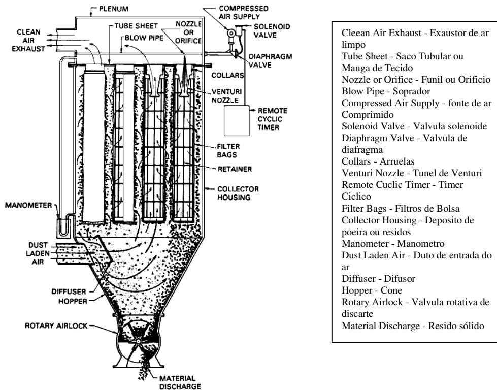
Figura 5: Sistema básico de operação de um Filtro de Manga.
