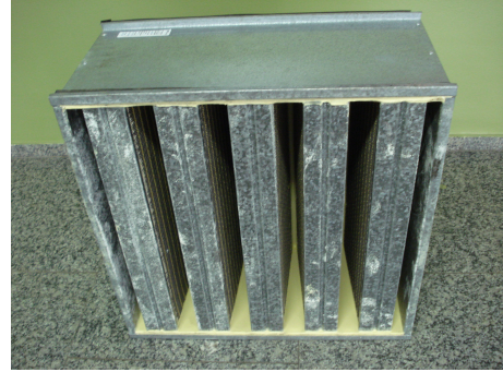
Figura: 27 Filtro absoluto contaminado
