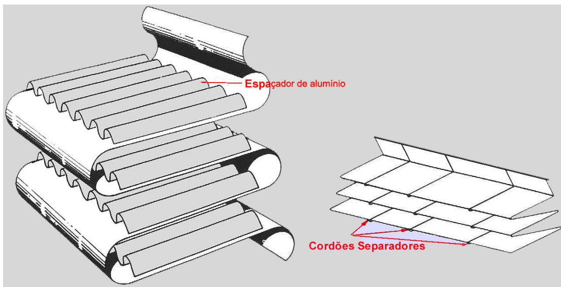
Figura 8: Dois diferentes modos de separar os plissos, utilizando espaçadores de alumínio e cordões separadores.
