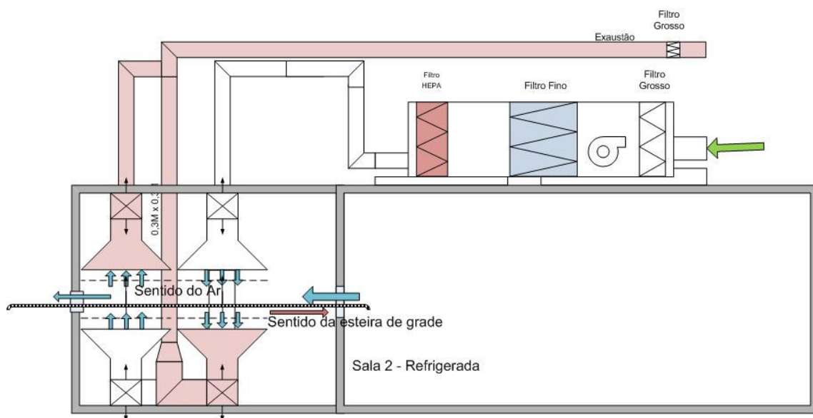
Figura 30: Sala 1 modificada com sistema alternado de ventilação
