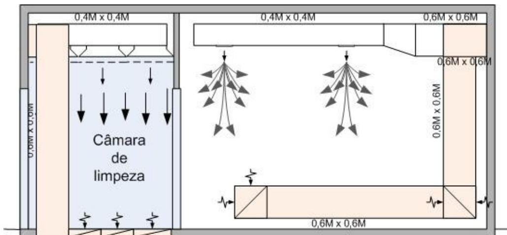
Figura 15: Sala com fluxo ar turbulento, retorno e câmara de limpeza.
