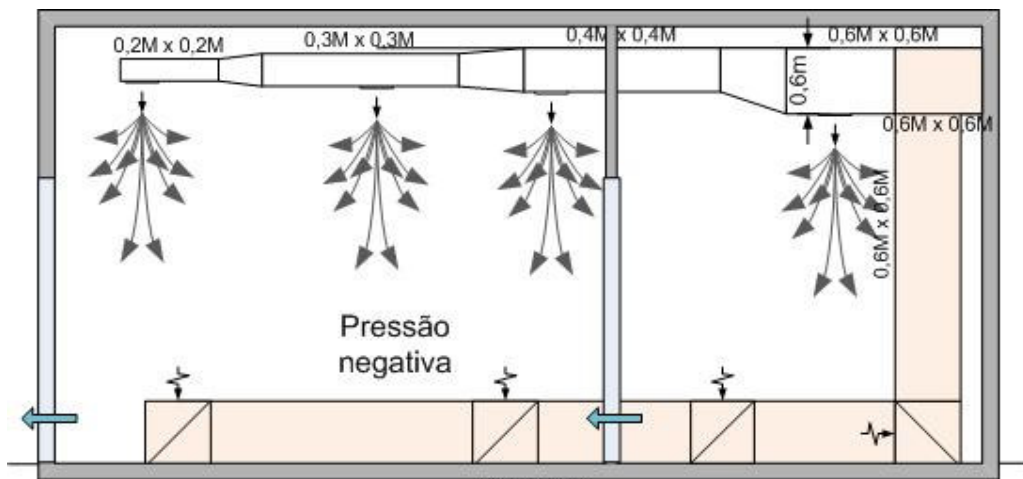
Figura 12: Sala com fluxo de ar turbulento com retorno
