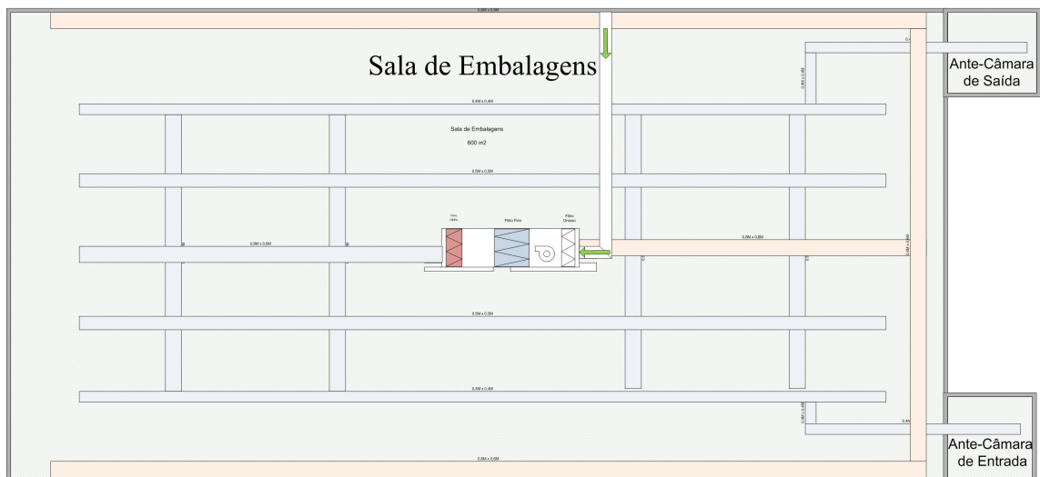
Figura 20: Planta Baixa do conjunto de operação das salas limpas
