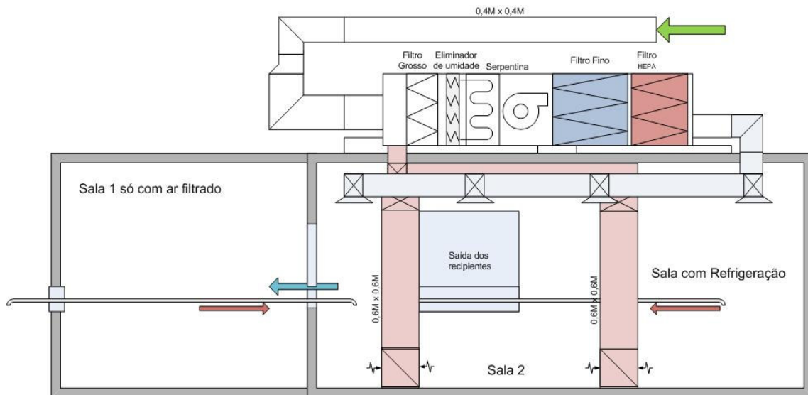
Figura 18: Corte com a apresentação do fluxo de ar para a sala2 – UTA - 1
