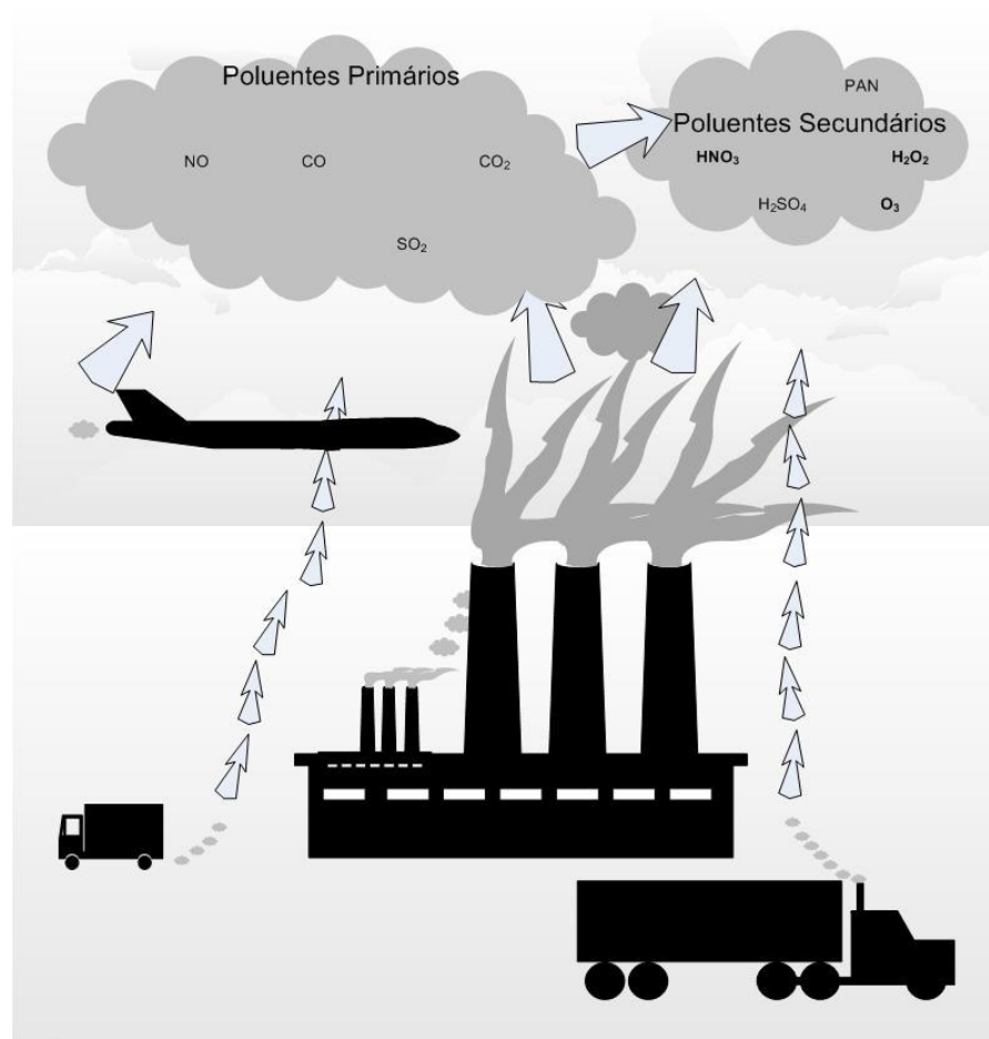
Figura: 2: Processo que ocorre na atmosfera desde a emissão dos poluentes primários até a formação dos poluentes secundários
