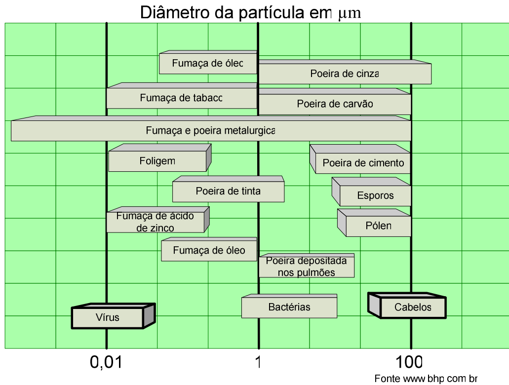
Figura 3: Tamanho de partículas mais comuns encontradas nos ambientes
