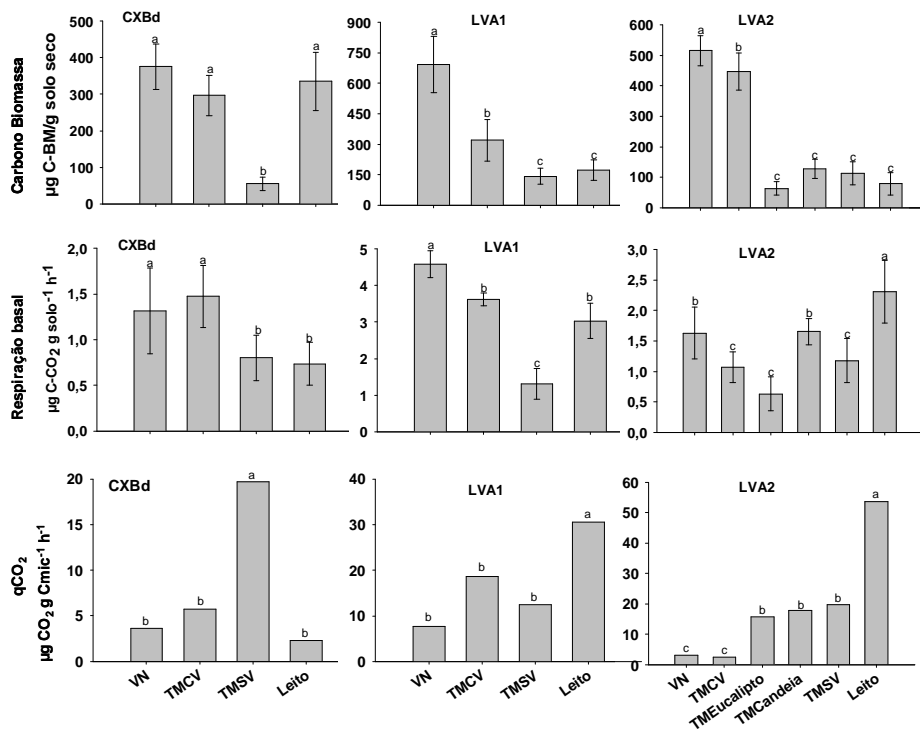
FIGURA 2 Carbono da biomassa microbiana, respiração basal e quociente metabólico ( qCO_2 ) em diferentes ambientes de três voçorocas no município de Lavras, MG. CXBd - Cambissolo háplico, e LVA1 e LVA2-Latossolo Vermelho-Amarelo. Barras verticais representam o erro padrão da média. Médias seguidas pela mesma letra nas barras não diferem, pelo teste de Scott-Knott, a 5%.
