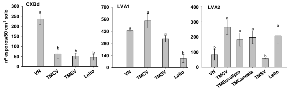
FIGURA 3 Número de esporos ( 50 \text{ cm}^3 solo) de FMAs em diferentes ambientes de três voçorocas no município de Lavras, MG. CXBd - Cambissolo, e LVA1 e LVA2 - Latossolo Vermelho-Amarelo. Barras verticais representam o erro padrão da média. Médias seguidas pela mesma letra nas barras não diferem, pelo teste de Scott-Knott, a 5%.
