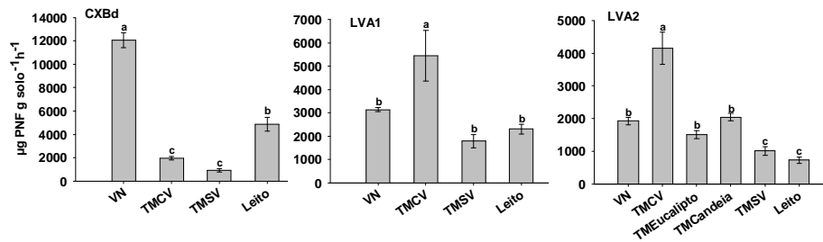
FIGURA 4 Atividade da fosfatase em diferentes ambientes de três voçorocas no município de Lavras, MG. CXBd ó Cambissolo háptico e LVA1 e LVA2 - Latossolo Vermelho-Amarelo. Barras verticais representam o erro padrão da média. Médias seguidas pela mesma letra, nas barras, não diferem, pelo teste de Scott-Knott, a 5%.
