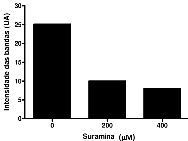
Figura 4.10: Efeito da suramina sobre o conteúdo de colesterol de L. amazonensis . Os lipídios extraídos de promastigotas de L. amazonensis após o tratamento com 200 \mu\text{M} e 400 \mu\text{M} de suramina por 24 horas foram separados por TLC, conforme mostrado na Fig. 4.11 e analisados por densitometria, sendo sua quantidade relativa expressa em unidades arbitrárias (UA). A imagem da TLC foi digitalizada e analisada pelo programa “ImageMaster TotalLab v1.11”.
