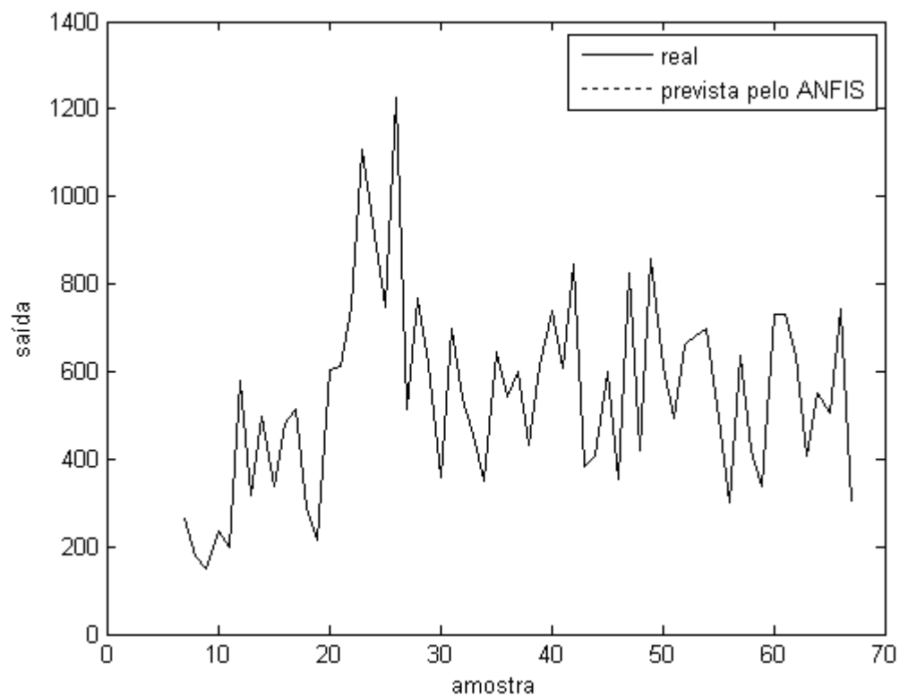
Figura 4.12 – Insumo X versus previsão do modelo ANFIS (Simulação 2)
