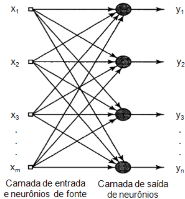
Figura 3.5 – Rede alimentada adiante com uma única camada de neurônios.
