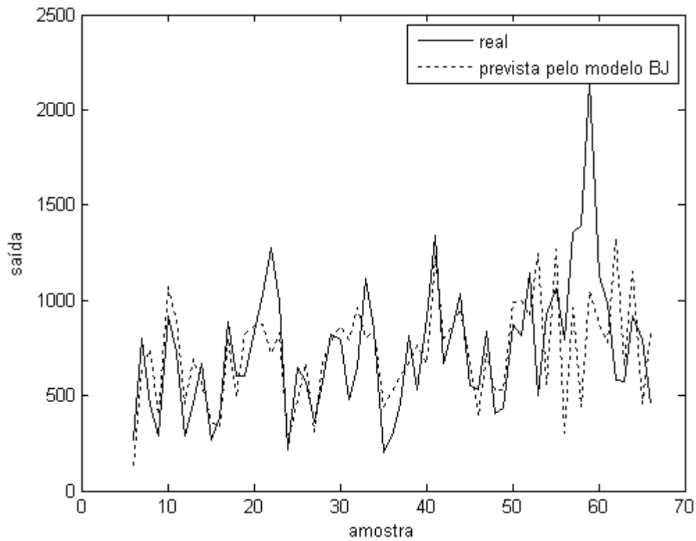
Figura 4.14 – Insumo Y versus previsão do modelo ARIMA (simulação 1)
