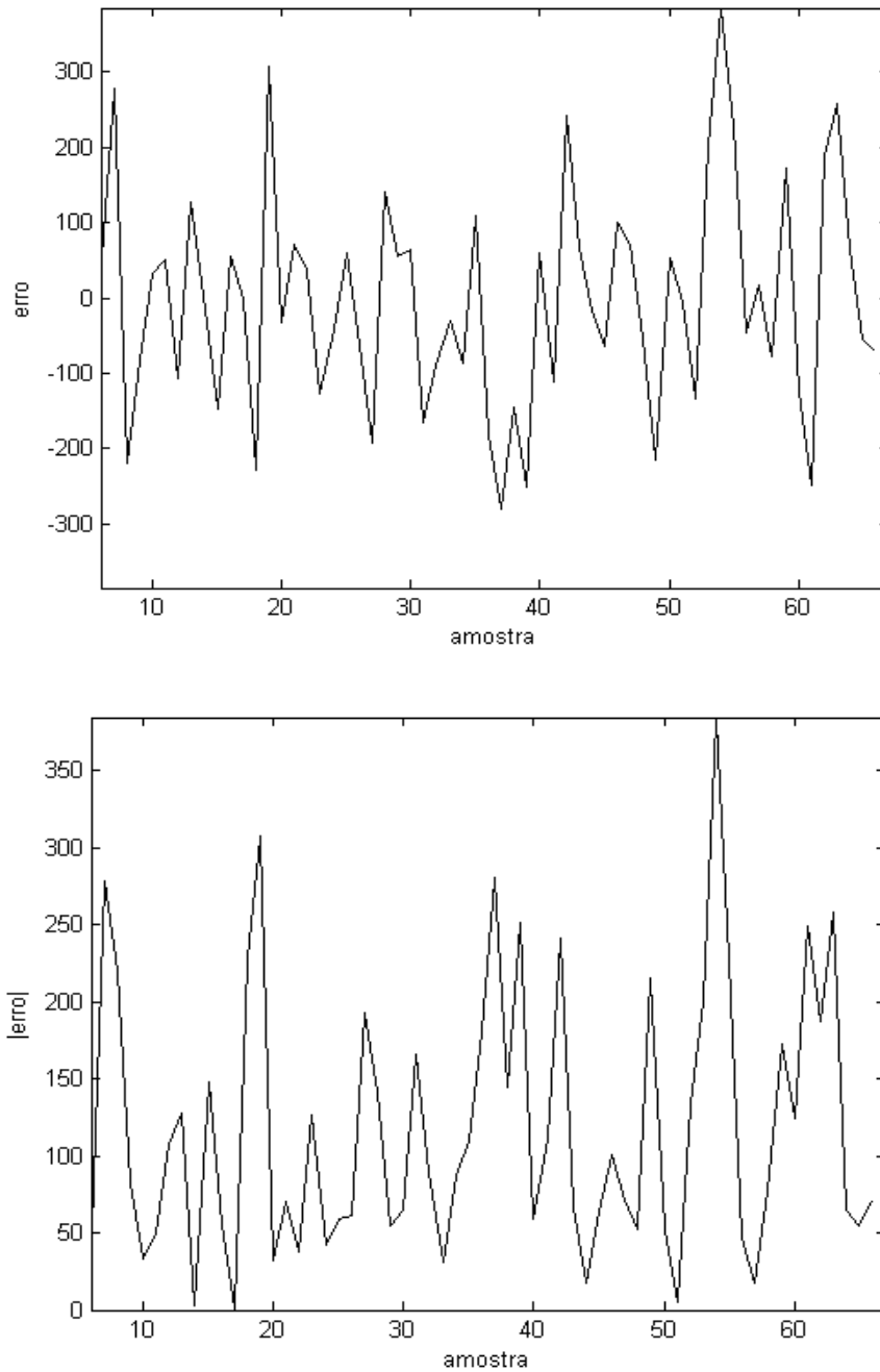
Figura 4.5 – Erros do modelo ARIMA Insumo X (Simulação 1)
