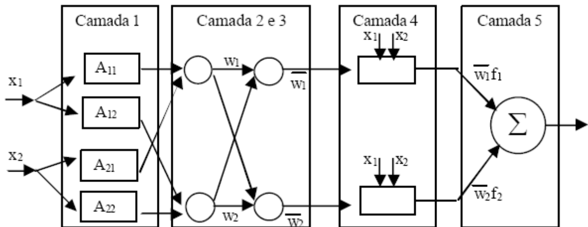
Figura 3.13 – Arquitetura ANFIS do tipo Takagi-Sugeno
