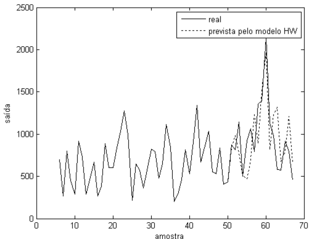
Figura 4.20 – Insumo Y versus previsão do modelo HW (Simulações 3 e 4)
