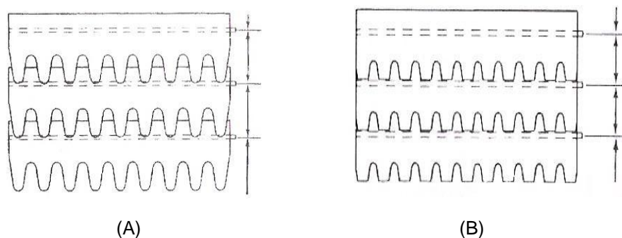
Figura 10 – Tipos de peneiras utilizadas nas colhedoras automáticas de fluxo axial: (A) Peneira superior 1-5/8 (B) Peneira inferior 1-1/8.
