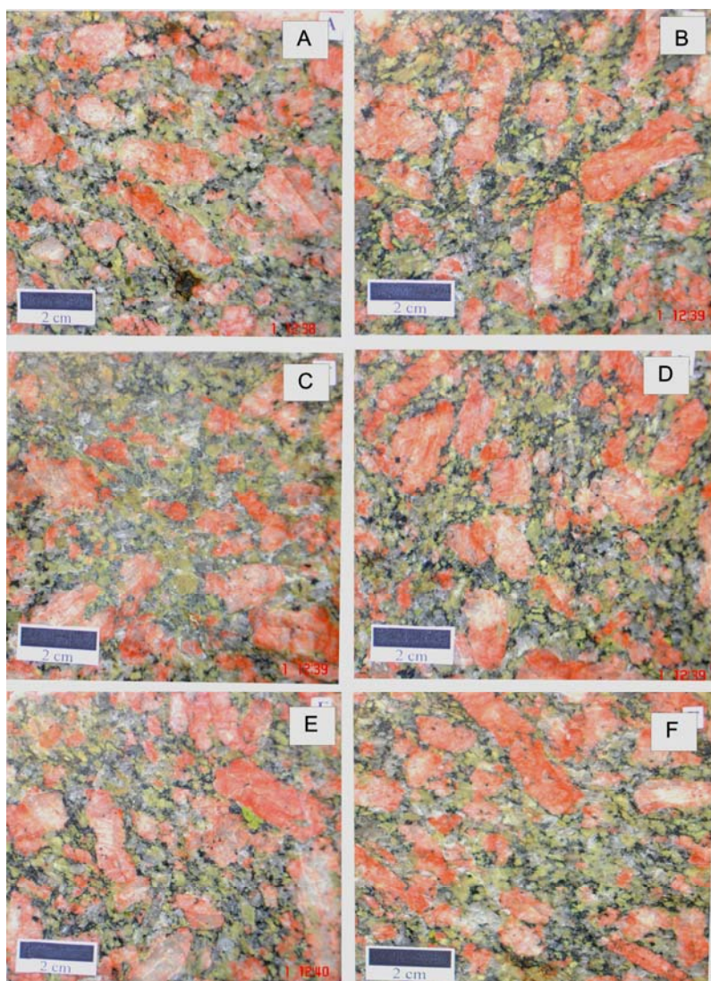
Prancha 24. Ortognaisse Fortuna (03) amostra neutra (A); ácido cítrico (B), ácido clorídrico (C), cloreto de amônia (D), hidróxido de potássio (E), hipoclorito de sódio (F).
