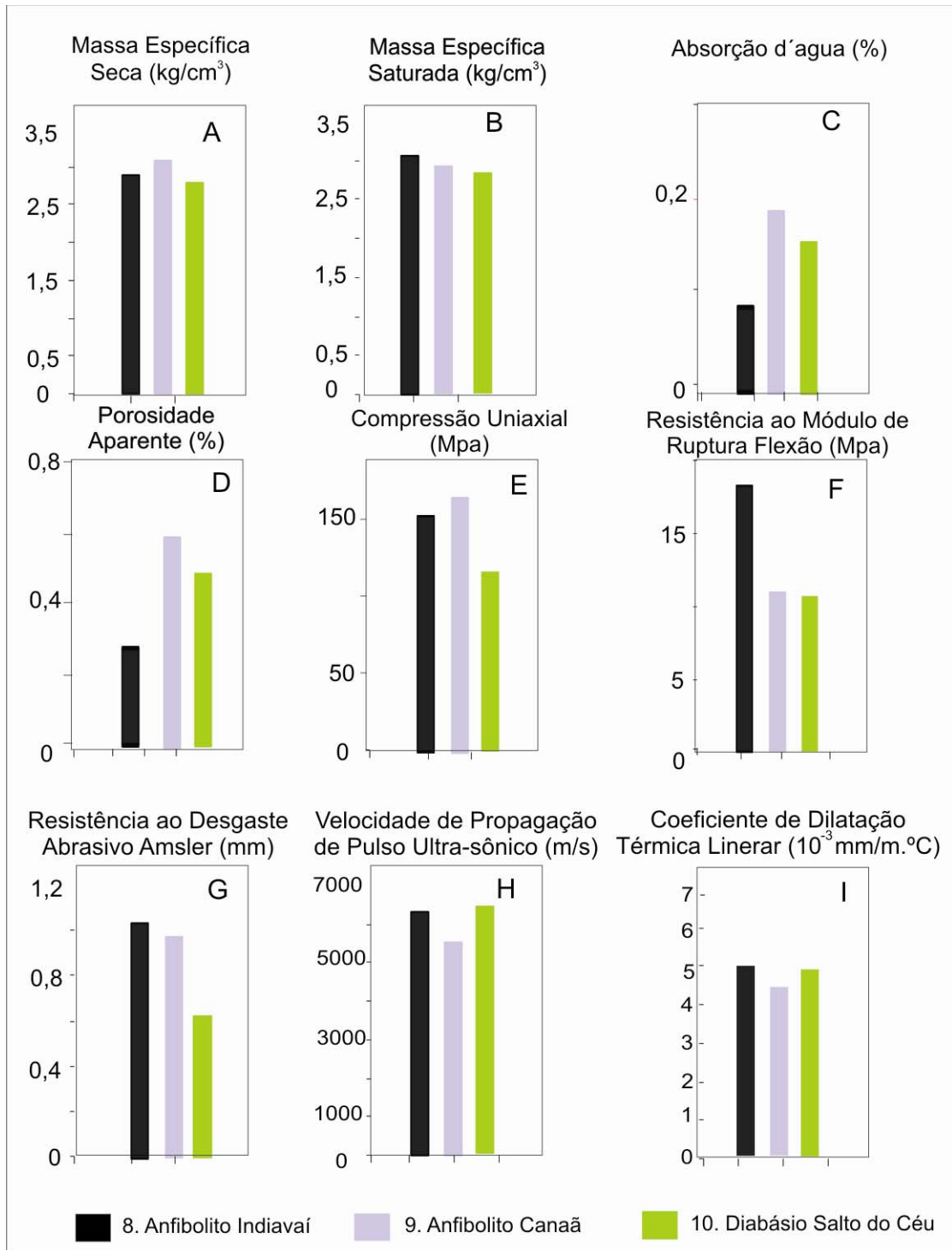
Figura 33. Representação gráfica dos resultados dos ensaios físico-mecânicos das rochas graníticas e movimentados pretos.
