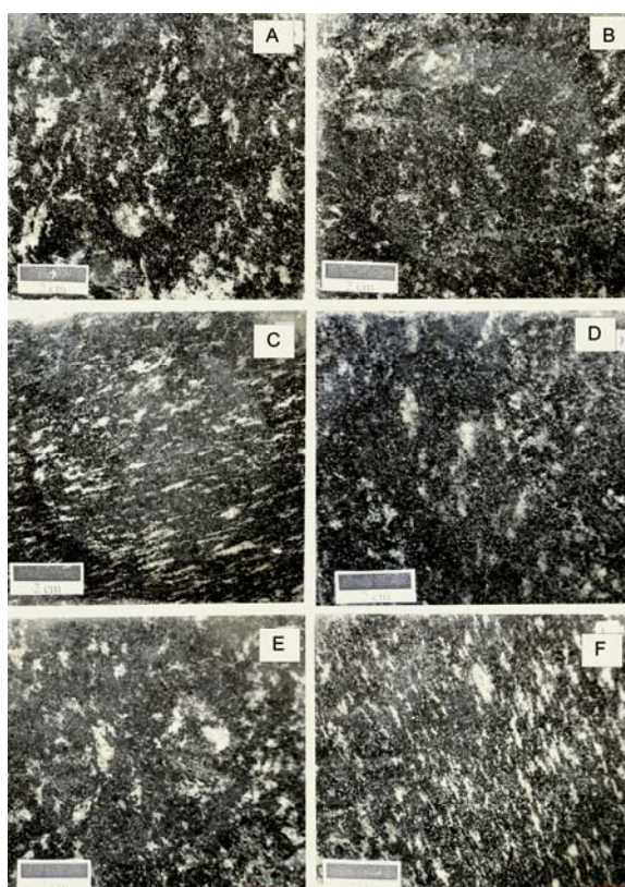
Prancha 29. Anfíbolito Indiavaí (08) amostra neutra (A); ácido cítrico (B), ácido clorídrico (C), cloreto de amônia (D), hidróxido de potássio (E), hipoclorito de sódio (F).
