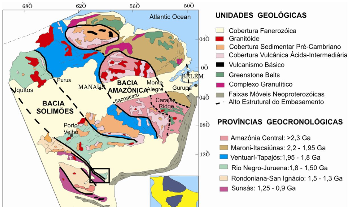
Figura 15. Situação da área dentro das províncias geocronológicas de Tassinari e Macambira (1999).
