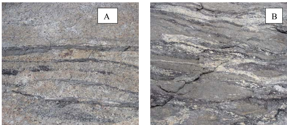
Prancha 11. Aspectos de campo do Ortognaisse Indiavaí Cinza
