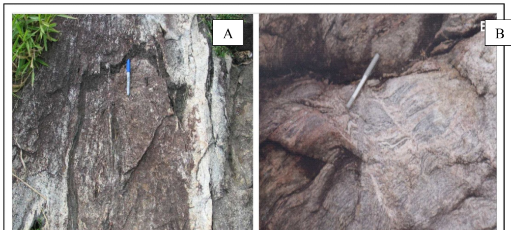
Prancha 13. Aspectos de campo dos Ortognaises do Domínio Cachoeirinha.
