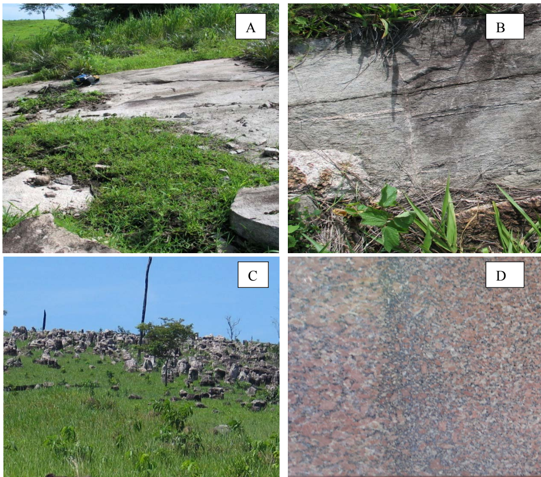
Prancha 7. Aspecto de campo e petrográficos do Ortognaisse Indiavaí Vermelho
