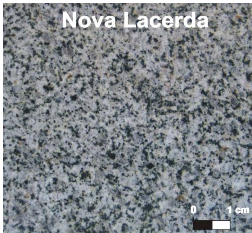
Figura 30. Aspectos de placas polidas do Granito Nova Lacerda
