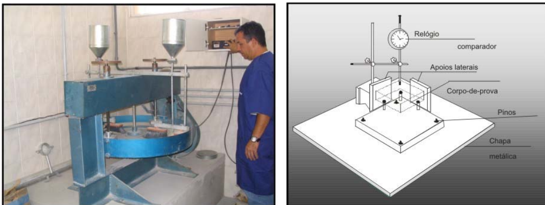
Figura 7. Equipamento utilizado para medir o desgaste por abrasão “Máquina Amsler”. Laboratório de Caracterização Tecnológica de Rochas Ornamentais da UNESP. Esquema do medidor do corpo-de-prova antes e após desgaste.
