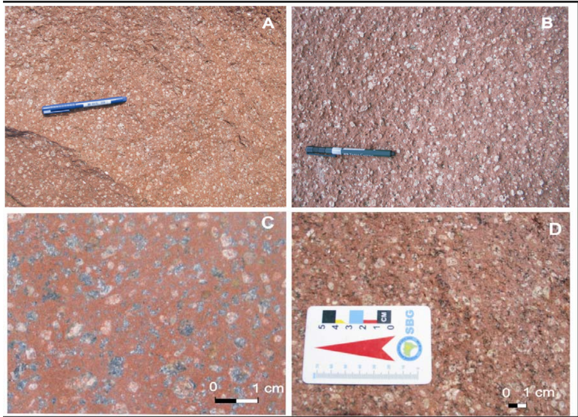
Prancha 3. As fotos A, B C e D mostram detalhes das placas apresentando os aspectos macroscópicos e a típica textura rapakivi do Granito Rio Branco.
