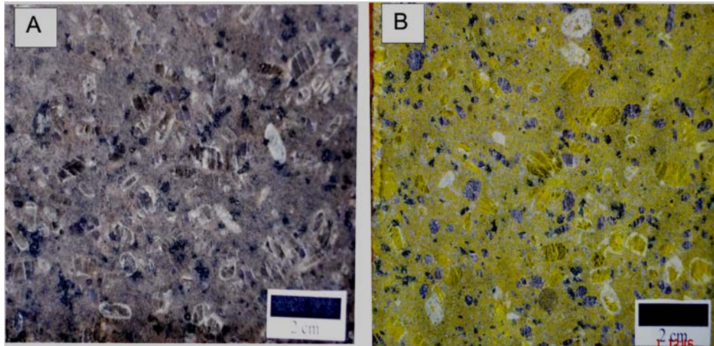
Prancha 12. Foto de placa de rocha (A) e ensaio de Colorimetria (B) do Ortognaisse Indiavaí Cinza.
