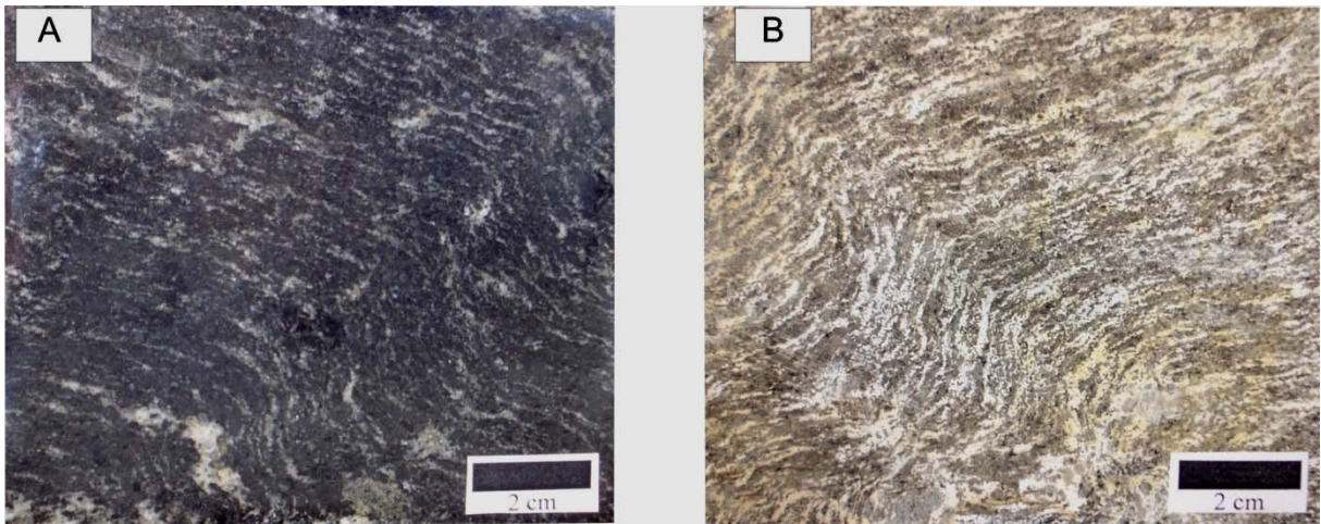
Prancha 16. Foto de placa de rocha (A) e ensaio de Colorimetria (B) do Anfíbolito Indaiavá
