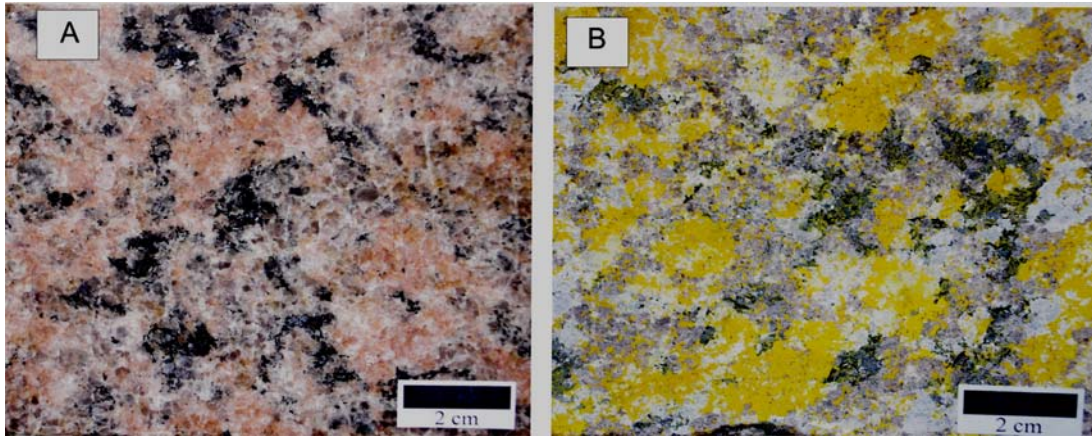
Prancha 8. Foto de placa de rocha (A) e ensaio de Colorimetria (B) do Ortognaise Indiavaí Vermelho.
