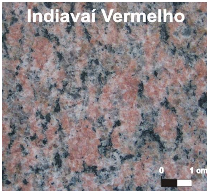
Figura 27. Aspectos de placas polidas do Ortognaisse Indiavaí Vermelho.
