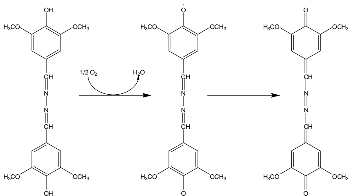
Figura 13: Reação de seringaldazina na presença de lacase (Sanchez-Amat & Solano, 1997; Mayer & Staples, 2002).
