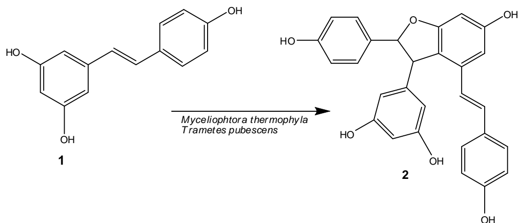
Figura 5: Biotransformação do trans-resveratrol (1) realizada por lacases dos fungos Myceliophthora thermophyla e Trametes pubescens em dímero \epsilon -viniferina (2) (Nicotra et al. , 2004).
