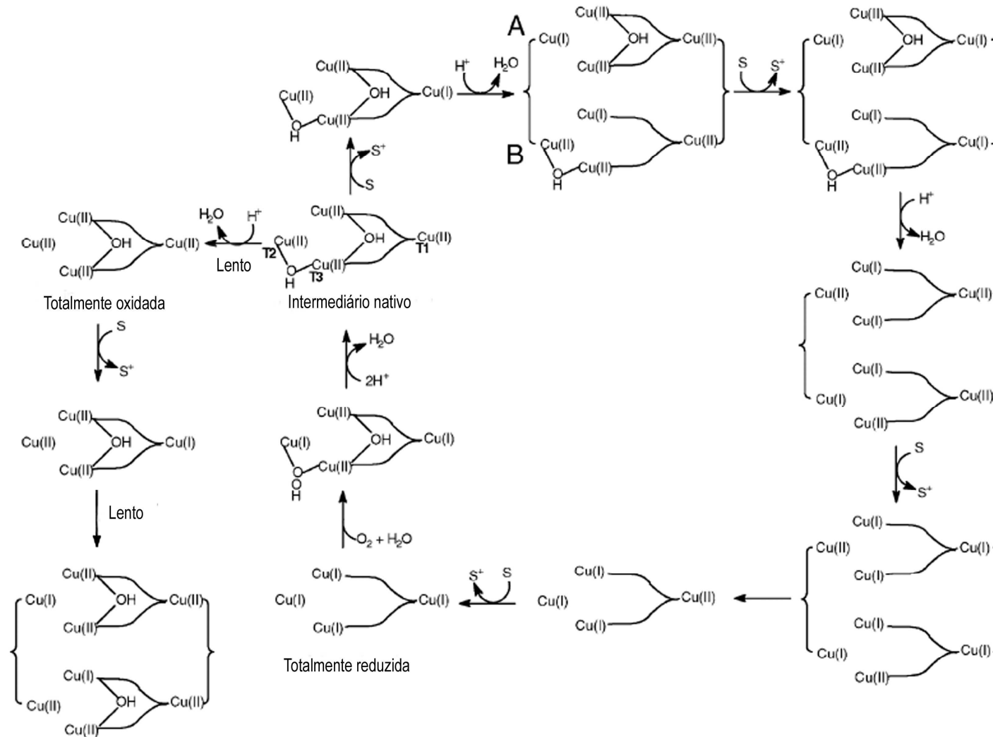
Figura 2: Ciclo catalítico da lacase (Gianfreda et al. , 1999; Durán et al. , 2002).
