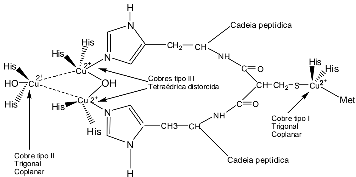
Figura 1: Representação esquemática dos centros de cobre da lacase e indicação das geometrias obtidas por cristalização (Durán et al. , 2002; Piontek et al. , 2002).
