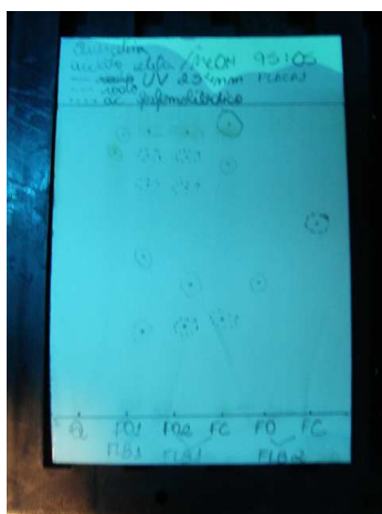
Figura 17: Cromatoplaça das frações acetato de etila e cetônica do experimento A. Condições cromatográficas: fase móvel Acetato de etila/metanol (95:05) e diferentes reveladores. Reveladores: UV (254nm) (365nm), Iodo, Ácido fosfomolibdico.
