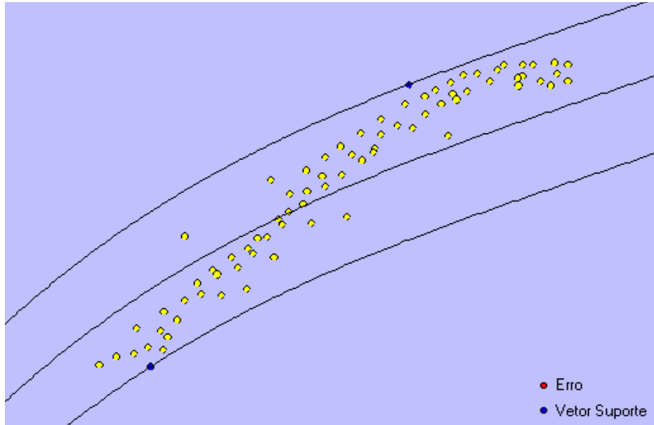
FIGURA 13 - RESULTADO DO SVR COM KERNEL POLINOMIAL NÃO HOMOGÊNIO E PARÂMETROS p=4 E k=2
