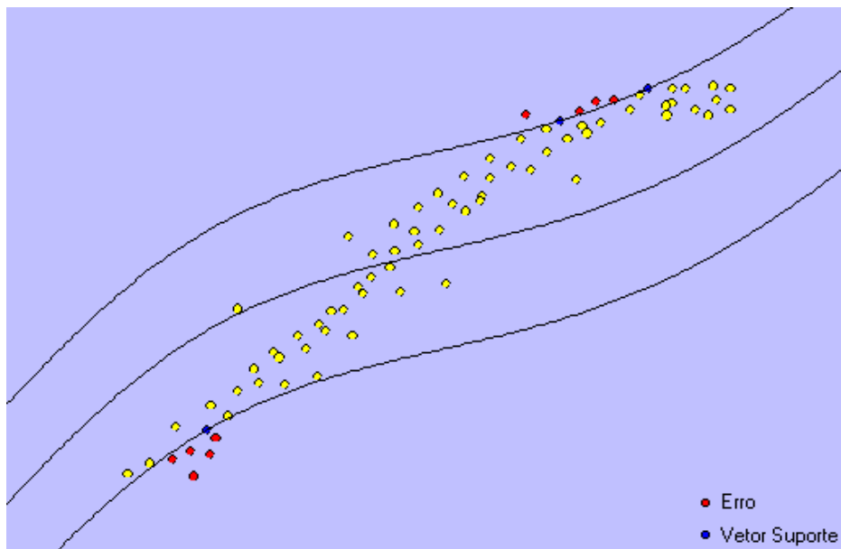
FIGURA 14 - RESULTADO DO SVR COM KERNEL SIGMOIDAL E PARÂMETROS \kappa=2 E k=-1,7
