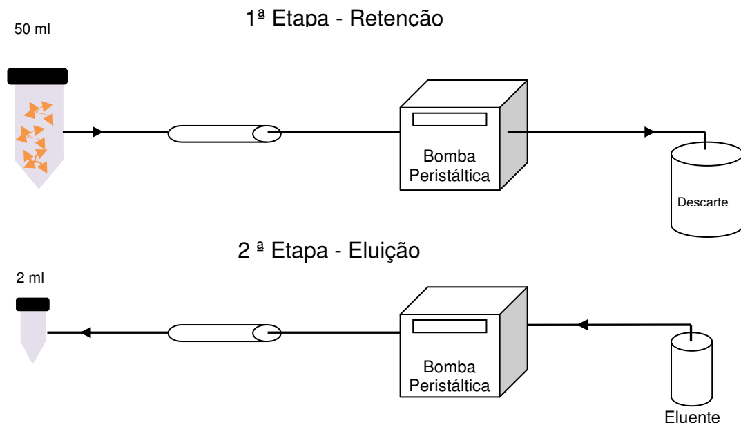
Figura 5: Etapas de extração em fase sólida.
