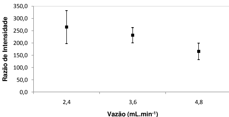
Figura 16: Variação da vazão de 2,4 a 4,8 mL min -1 em padrão de 25 µg L -1 de Cd com 1% de HNO 3 , 0,3% de DDTP e eluição com 4,7 mol L -1 de HNO 3 . ■ (média) e I (desvio padrão).
