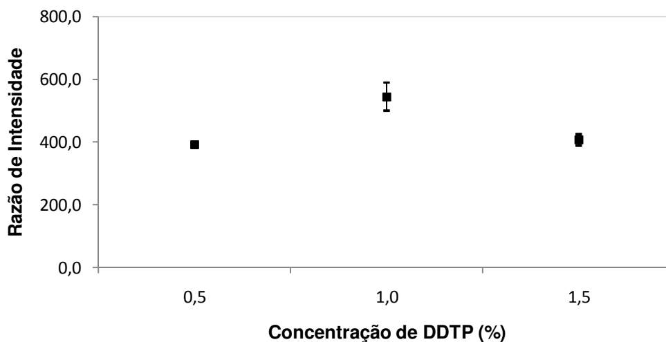
Figura 9: Variação da concentração de DDTP de 0,5 a 1,5 % em padrão de 25 \mu\text{g L}^{-1} de Cd com 0,32 \text{mol L}^{-1} de HCl e 0,05% de Triton X-114. ■ (média) e I (desvio padrão).
