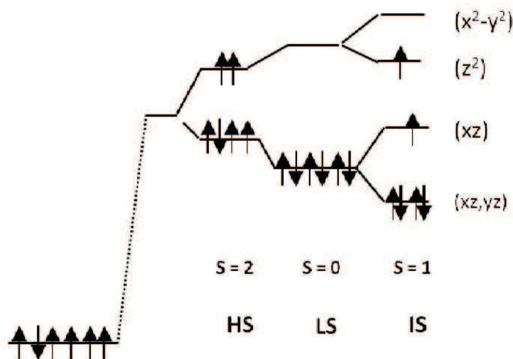
Figura 5.3: Diagrama esquemático da possível configuração dos íons de \text{Co}^{+3} .
