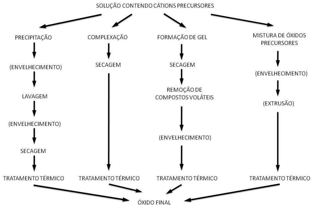
Figura 3.1: Representação esquemática das reações envolvidas no método.
