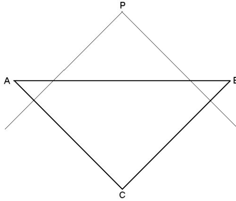
Figura 2.2: Contorno de integração usado na derivação de (2.26).
