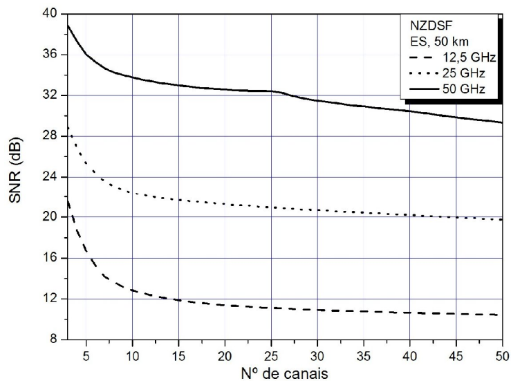
Figura 3.21 – SNR em função do número de canais.
