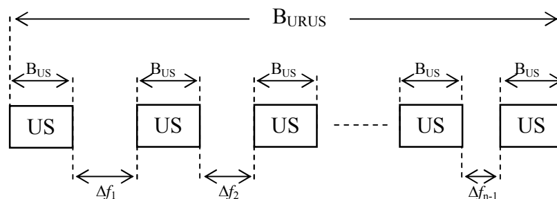
Figura 4.7 – Sistema WDM de N canais com alocação RDE-DE de base M com espaçamento variável entre unidades de base.
