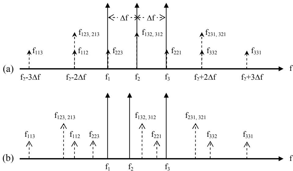
Figura 2.2 Esboço de três ondas injetadas com frequências f_1 , f_2 e f_3 e as nove ondas geradas pelo processo de FWM para (a) separação ( \Delta f ) uniforme entre as frequências dos canais e (b) separação não uniforme entre as frequências dos canais. Reproduzido de acordo com SHIBATA et al (1987), ZEILER (1995) e NUMAI (2000).
