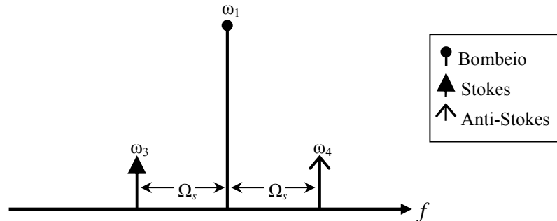
Figura 2.1 – Ondas Stokes e anti-Stokes geradas a partir de um bombeio de alta potência.
