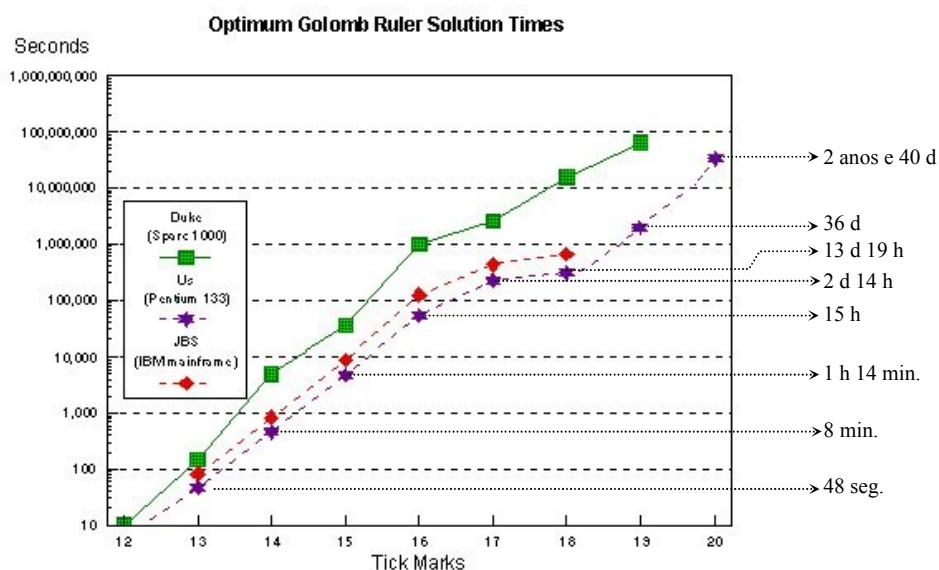
Figura 3.6 – Tempo necessário para determinar OGRs em função do número de marcas. O computador Pentium 133 operou com 100% do tempo de CPU dedicado ao processo OGR utilizando algoritmo otimizado. Fonte: http://members.golomb20.com/about.htm .
