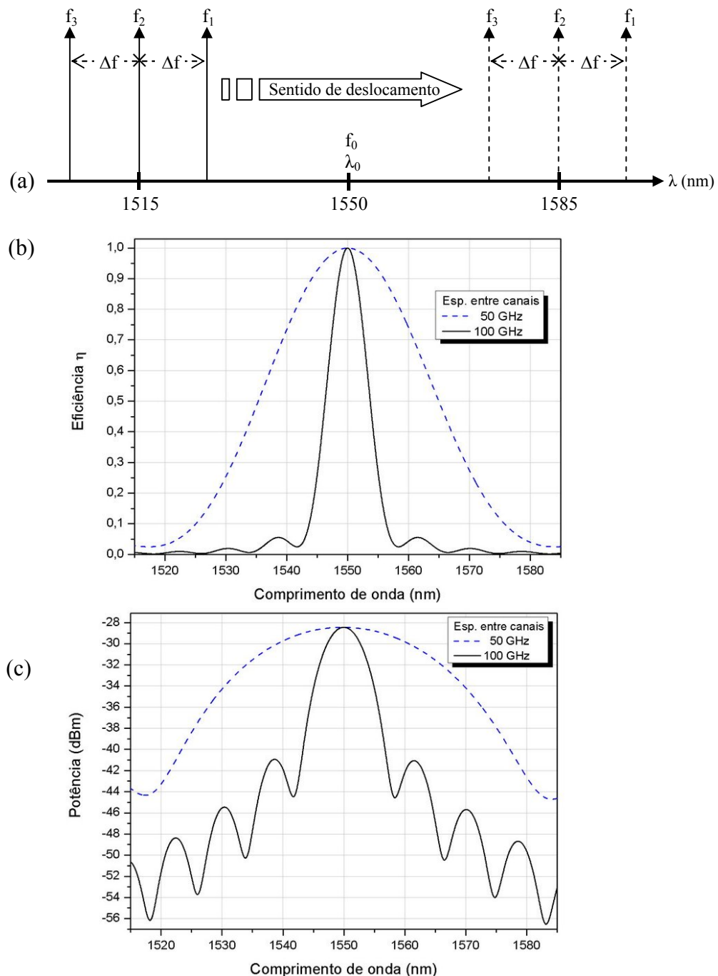
Figura 3.1 – Esboço das três ondas injetadas com frequências f_1 , f_2 e f_3 onde: (a) alocação inicial e final do arranjo de canais, (b) variação da eficiência e (c) variação de potência de FWM nas componentes f_{132} e f_{312} em função do comprimento de onda do canal central em uma fibra DSF.
