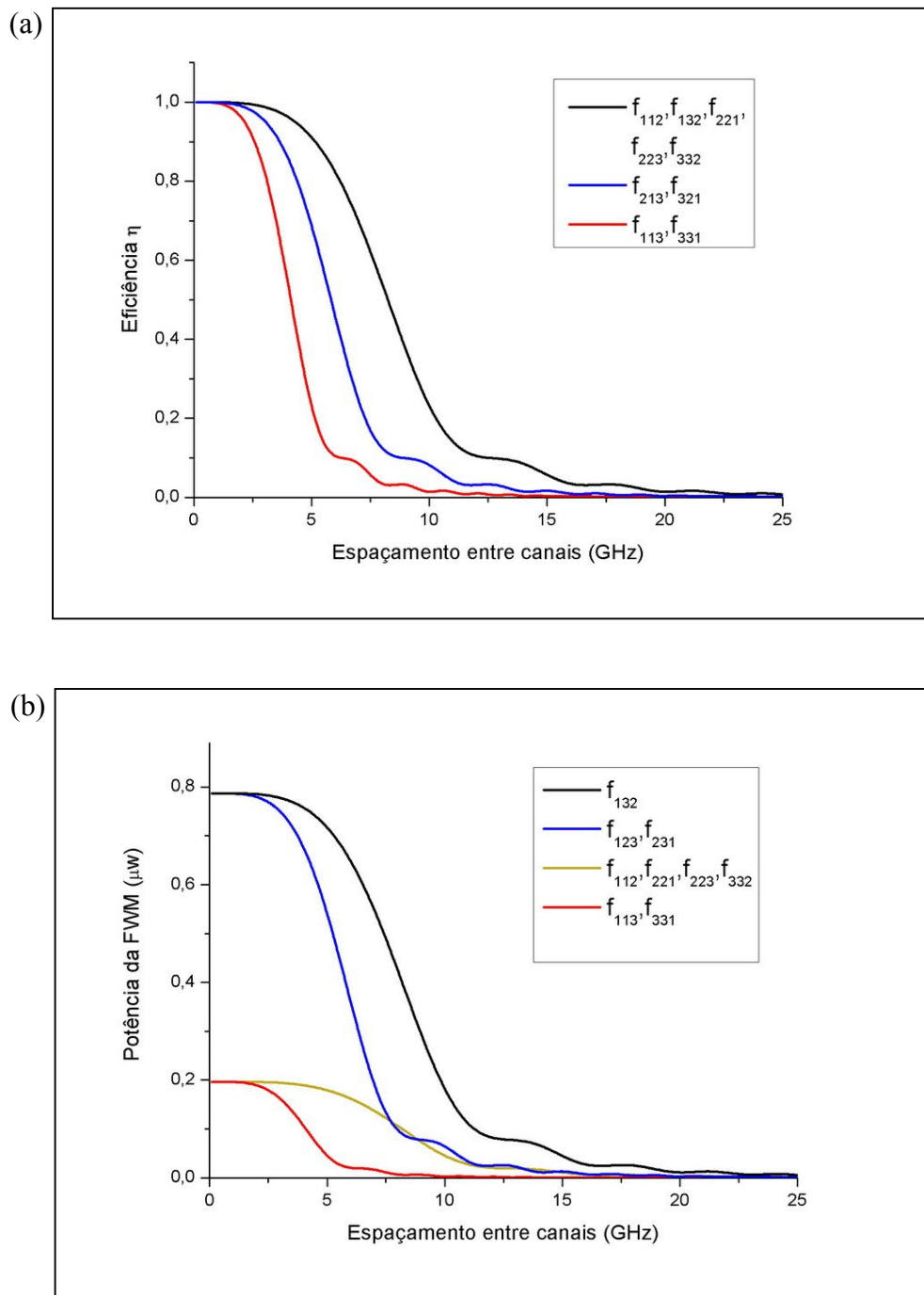
Figura 2.6 – Cálculo de (a) Eficiência \eta e (b) Potência de FWM em função do espaçamento entre canais ( \Delta f ) para os diferentes componentes de FWM em um sistema de três canais utilizando fibra SMF. Reproduzido de acordo com ZEILER (1995).
