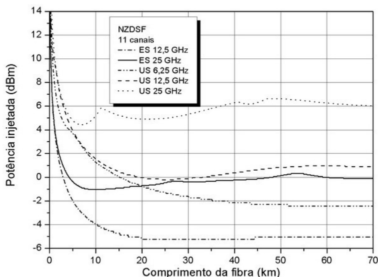
Figura 3.18 – Potência injetada em função do comprimento de fibra NZDSF para sistema de 11 canais, SNR \geq 23 dB.
