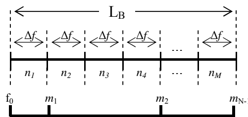
Figura 3.7 – Alocação de canais baseada em Régua de Golomb.
