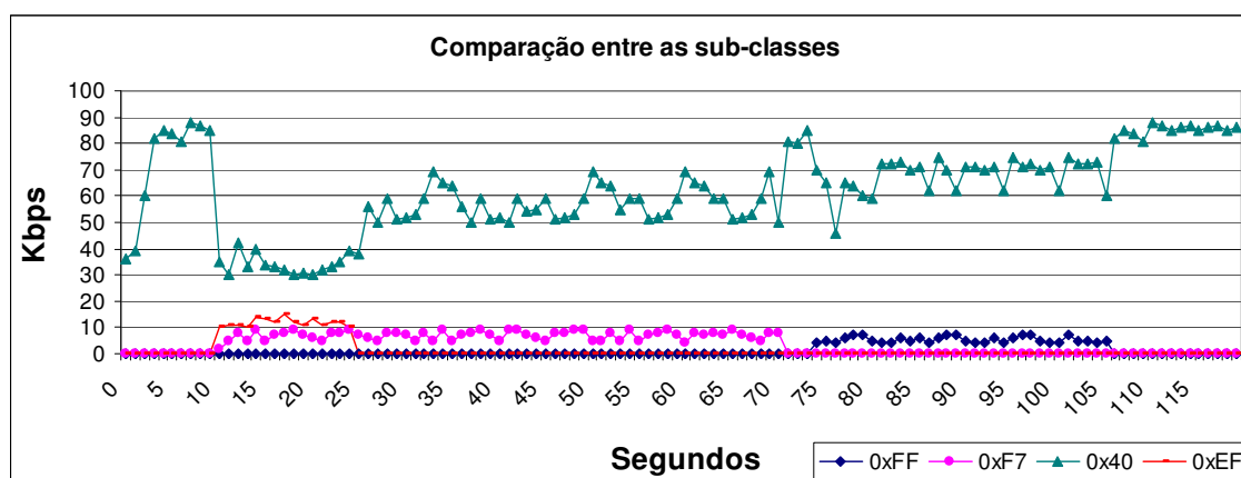
Figura 37: Gráfico com priorização de pacotes.
