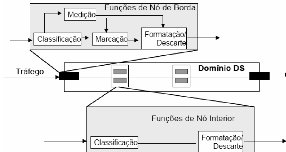
Figura 6 Roteador que implementa arquitetura DiffServ
