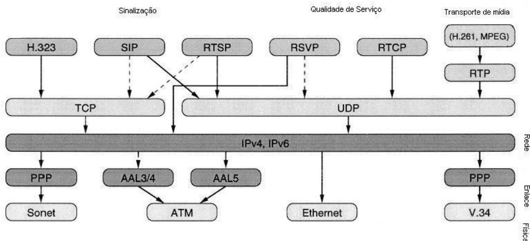
Figura 3: Pilha de Protocolos
