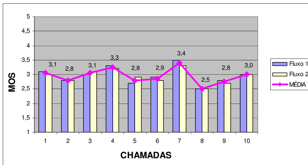
Figura 41: Valores de MOS obtidos com 10 chamadas de teste (rede sem QoS).
