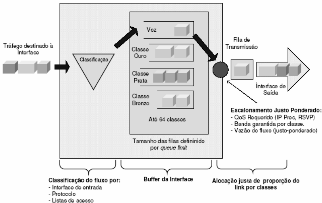
Figura 15: O mecanismo de escalonamento CB-WFQ
