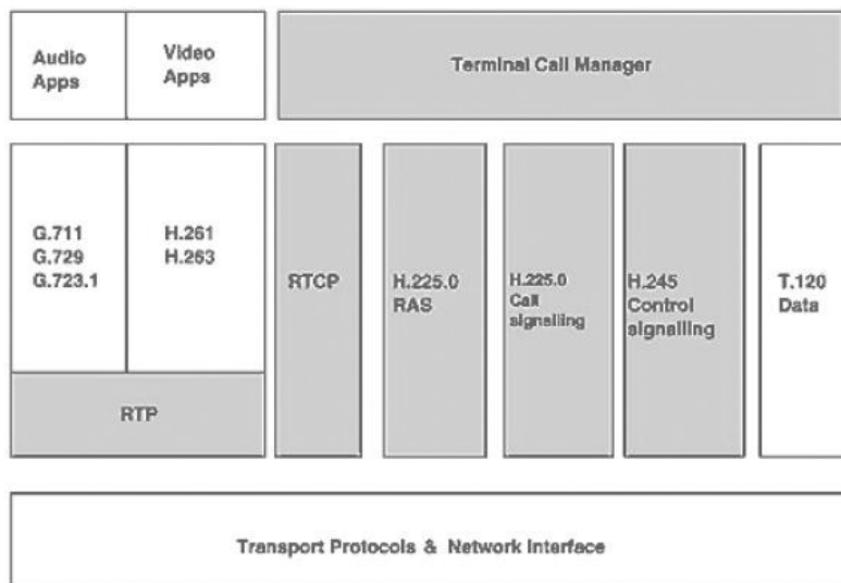
Figura 2: Pilha H.323
