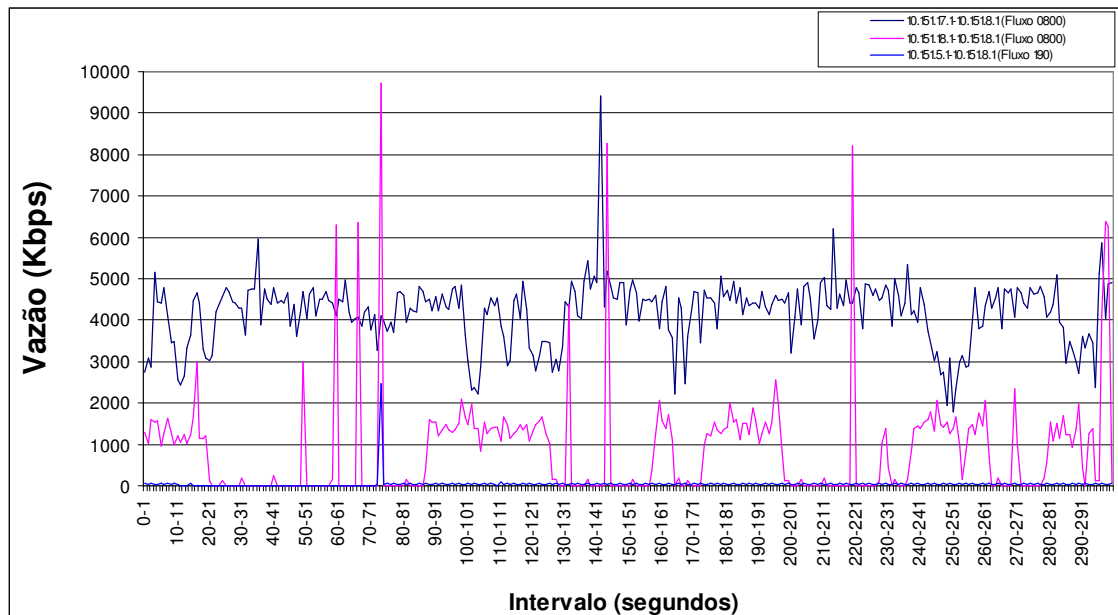
Figura 39: Influência dos fluxos 0800 no fluxo 190 (rede sem QoS).
