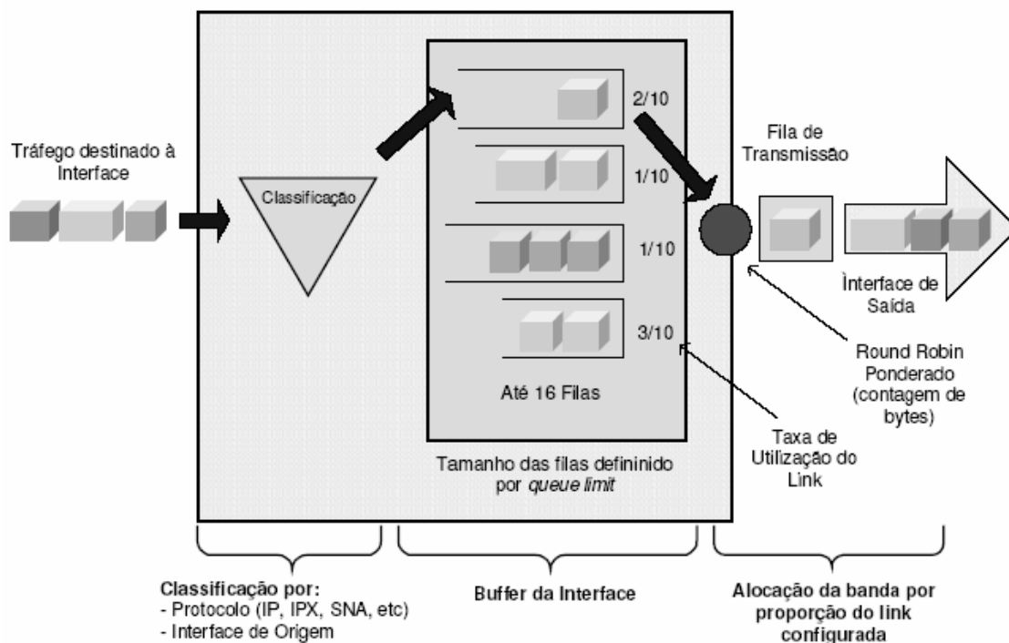
Figura 14: Filas do Custom Queueing
