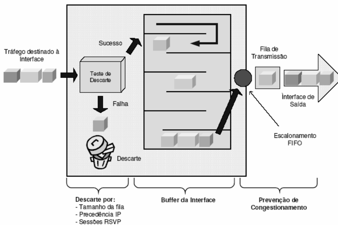
Figura 16: Filas de funcionamento do WRED
