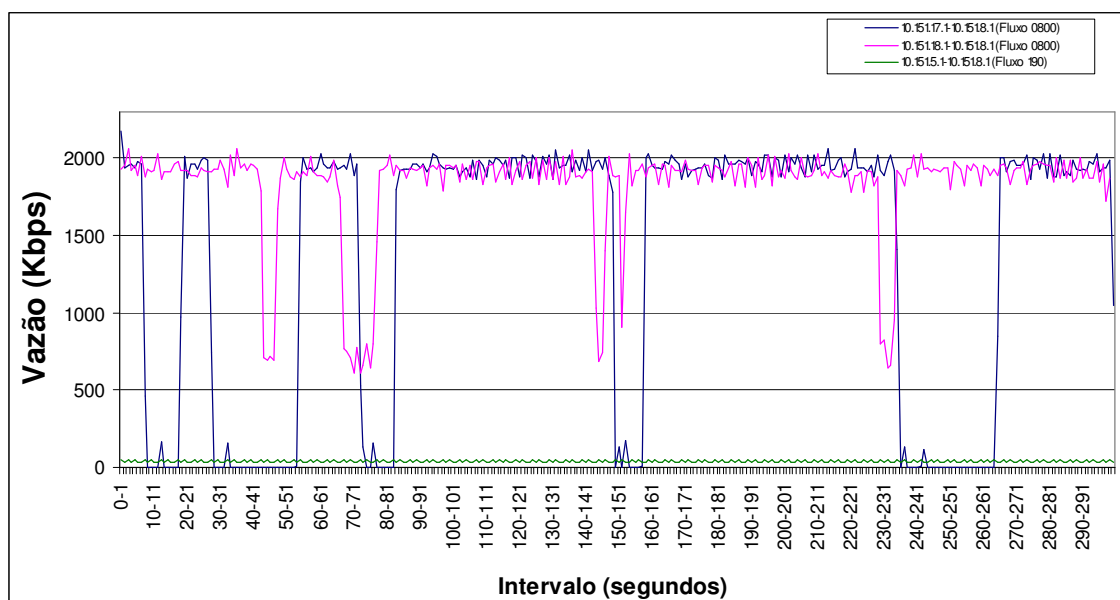
Figura 40: Influência dos fluxos 0800 no fluxo 190 (rede com QoS).
