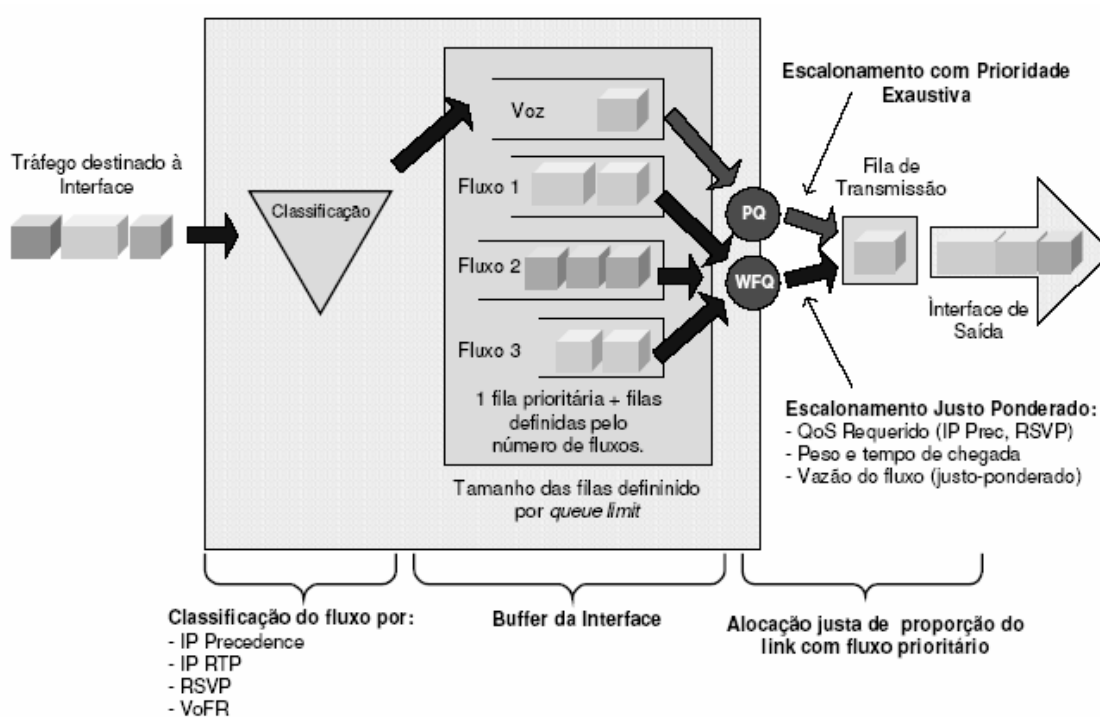
Figura 17: O mecanismo de escalonamento LLQ
