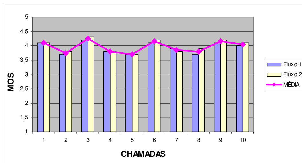
Figura 42: Valores de MOS obtidos com 10 chamadas de teste (rede com QoS).
