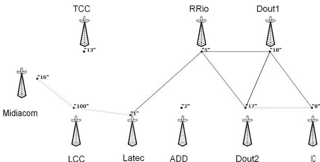
Figura 25: Rede mesh interna UFF.
