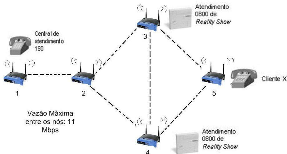
Figura 38: Topologia de testes na rede em malha sem fio.
