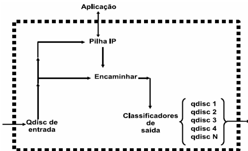
Figura 27: Disciplinas de filas nos dispositivos.
