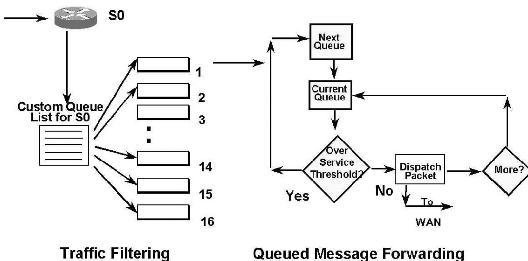
Figura 13: Operação do enfileiramento do Custom Queueing
