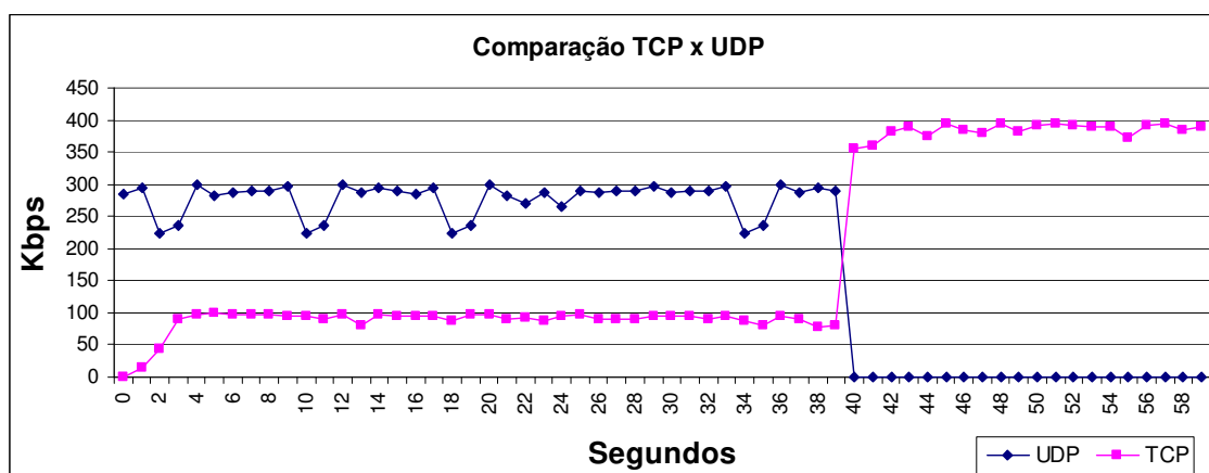
Figura 35: Gráfico comparativo TCP x UDP – prioridades iguais.
