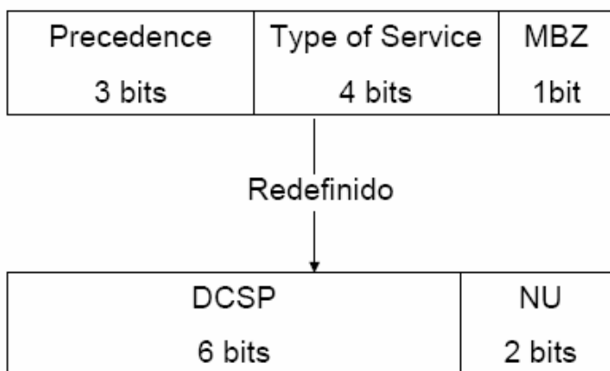
Figura 7: Campo TOS versus Byte DS
