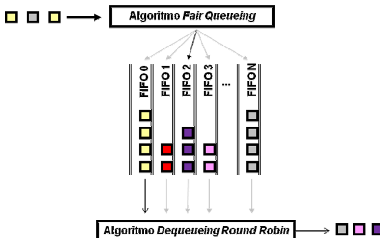
Figura 9: A estrutura do Stochastic Fairness Queueing .
