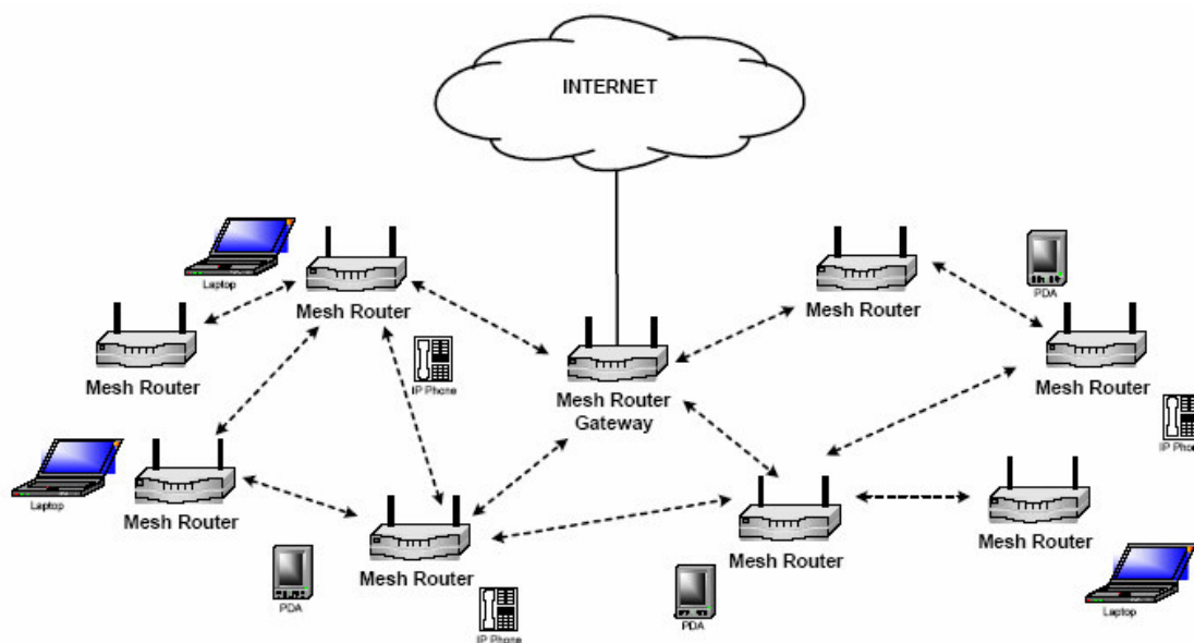
Figura 24: Infra-estrutura / backbone de uma rede mesh.
