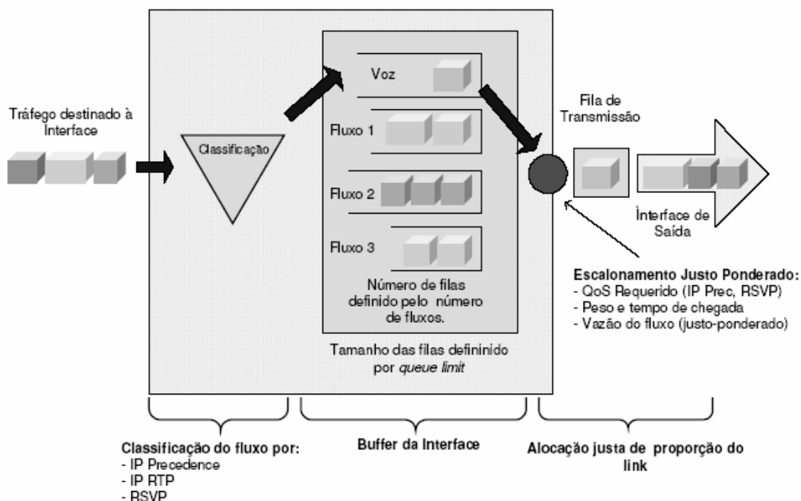
Figura 11: O funcionamento do Weighted Fair Queueing
