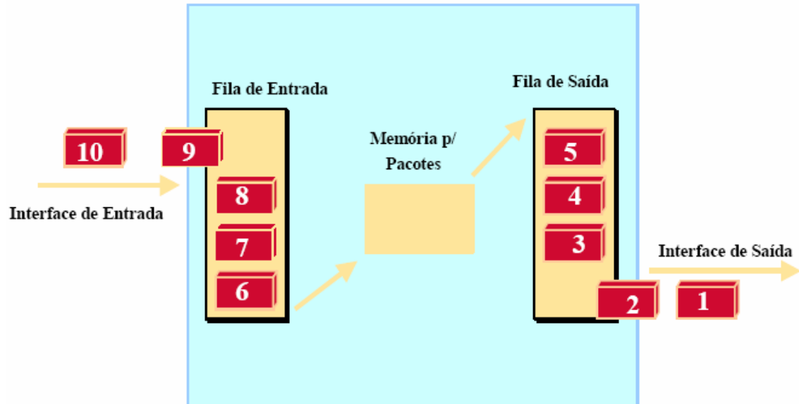
Figura 8: Uma fila FIFO.
