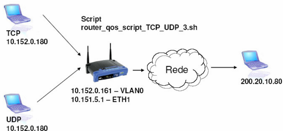
Figura 33: Validação TCP x UDP.
