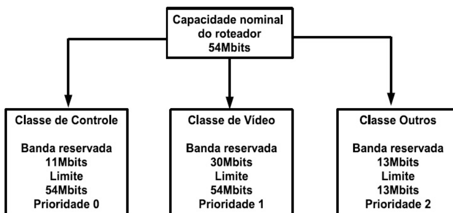
Figura 43: Estrutura de classes do mecanismo de reservas de recursos.
