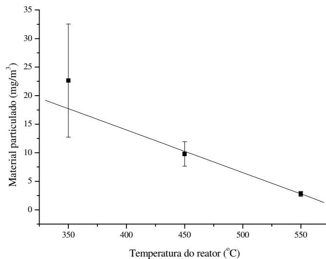
Figura 49. Material particulado em função da temperatura do catalisador ( \gamma -Alumina), com velocidade espacial de 50.000 h -1 , utilizando os gases de exaustão do biodiesel, gerados a partir do motor de baixa taxa de compressão (M1).
