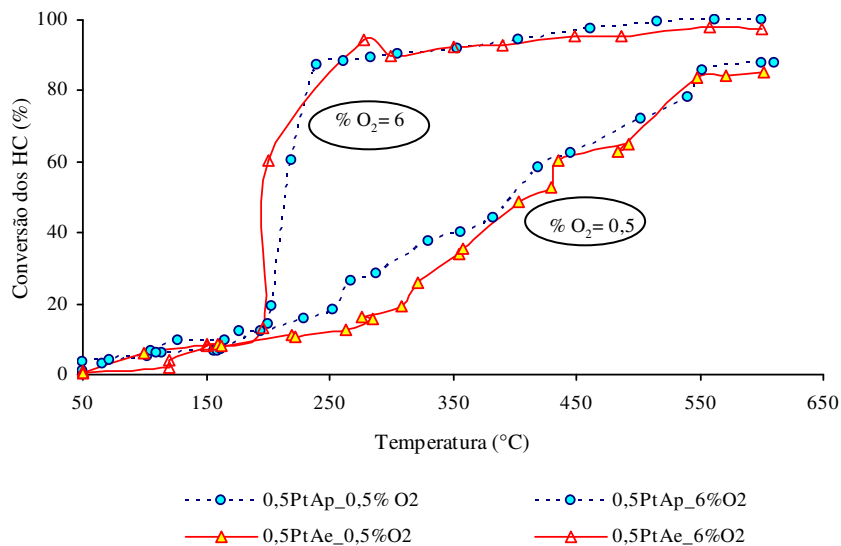
Figura 40. Conversão dos hidrocarbonetos dos gases de exaustão contendo distintas concentrações de oxigênio (6 e 0,5% molar) em função da temperatura, utilizando o catalisador 0,5Pt/A em esferas e em partículas, com velocidade espacial de 10.000 h -1 .
