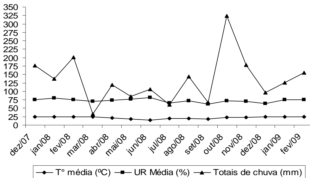
FIGURA 1. Representação das médias mensais de temperatura, umidade relativa e precipitação de dezembro de 2007 a fevereiro de 2009.
