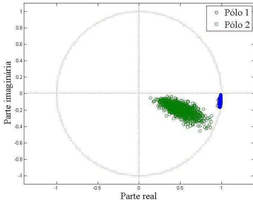
Figura 5.17 - Distribuição do conjunto de pares de pólos (1 e 2) no plano Z para sinais simulados do modelo I.
