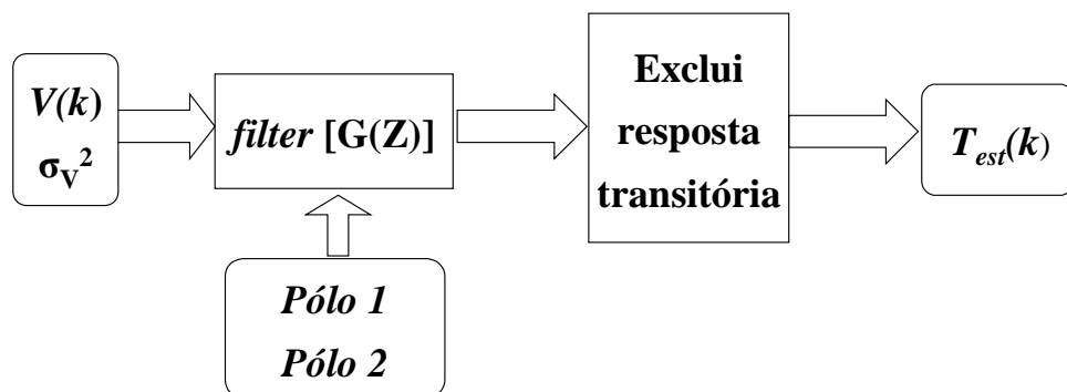
Figura 5.23 - Fluxograma da simulação do modelo AR do canal.
