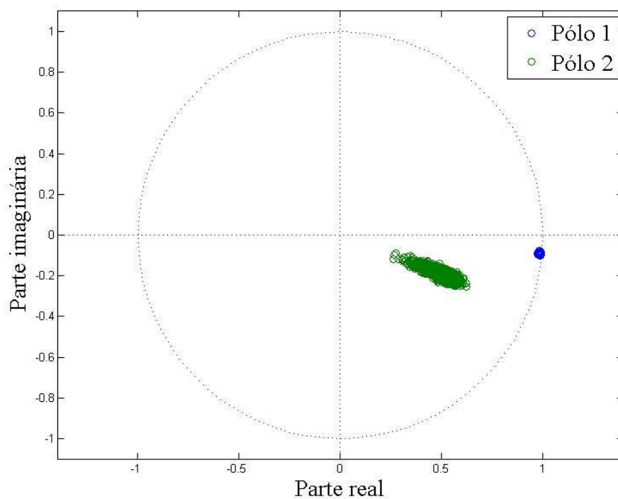
Figura 5.19 - Distribuição do conjunto de pares de pólos (1 e 2) no plano Z para sinais simulados do modelo III.
