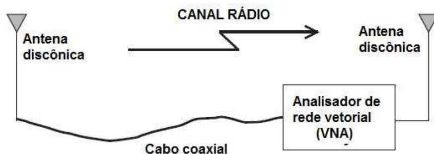
Figura 5.4 - Diagrama de blocos do equipamento utilizado para sondagem do canal no domínio da frequência.
