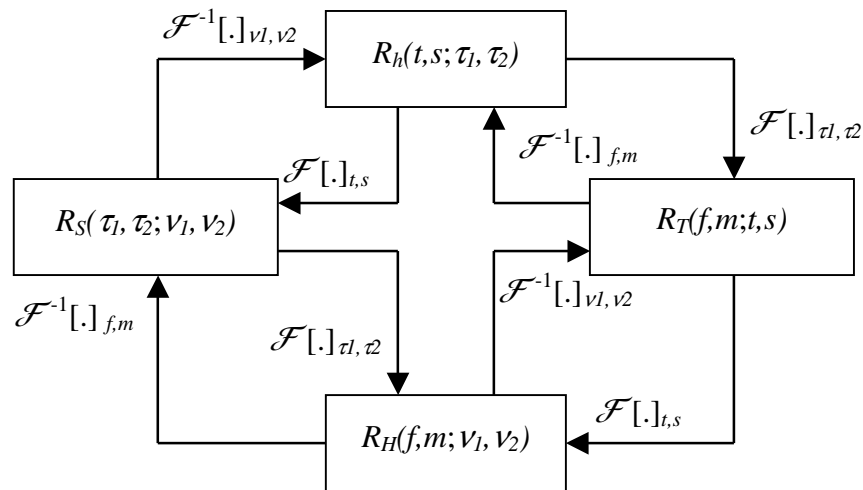
Figura 2.4 - Diagrama das relações das funções autocorrelação que representam o canal.
