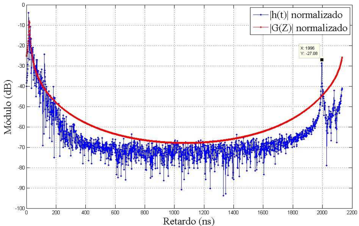
Figura 5.10 - Comparação entre as funções |h(\tau)| normalizadas: uma estimada pelo filtro G(Z) do modelo AR e outra obtida pela transformada inversa de Fourier discreta para uma dada medida T(k) .
