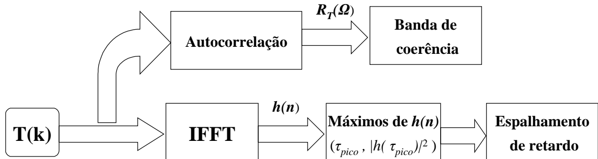
Figura 5.7 - Fluxograma para processamento da medida T(k) a fim de obter banda de coerência e espalhamento de retardo.
