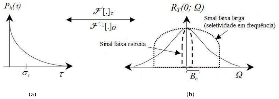
Figura 2.6 - Ilustração da relação entre (a) o perfil de potência de retardos com espalhamento de retardo \sigma_\tau e (b) autocorrelação R_T(0; \Omega) que apresenta a comparação entre a banda de coerência B_c do canal com as bandas de um sinal faixa larga e de um sinal faixa estreita (adaptado de [4]).
