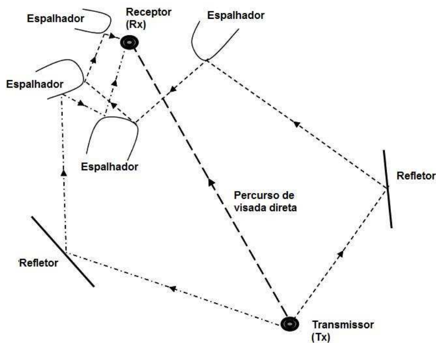
Figura 2.1 - Propagação em multipercursos do sinal transmitido em um canal rádio (adaptado de [4]).
