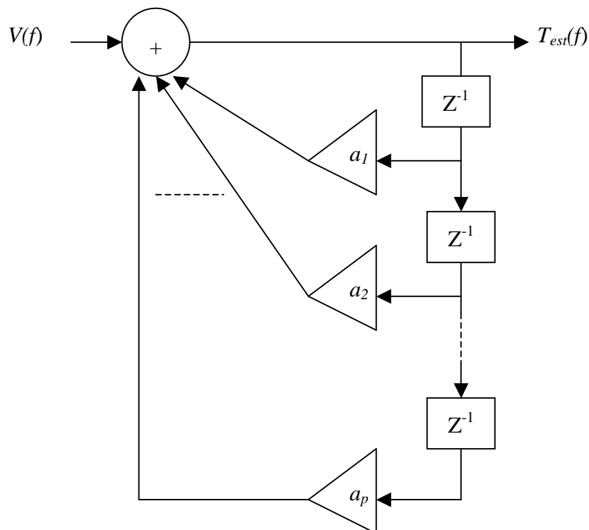
Figura 3.1 - Diagrama de blocos do modelo AR.
