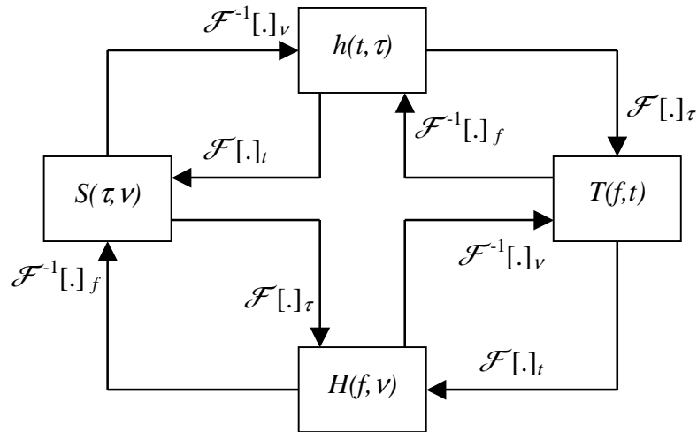
Figura 2.3 - Diagrama da relação entre as funções que representam o canal.
