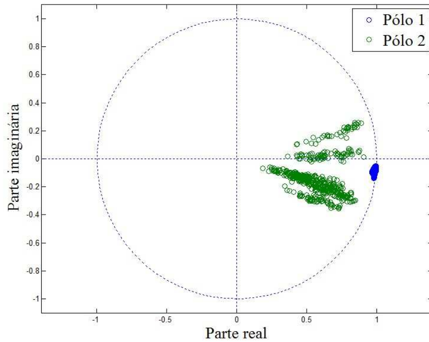
Figura 5.8 - Distribuição dos pares de pólos ( p_1 e p_2 ) referente às medidas de T(k) nos ambientes A, B e C.
