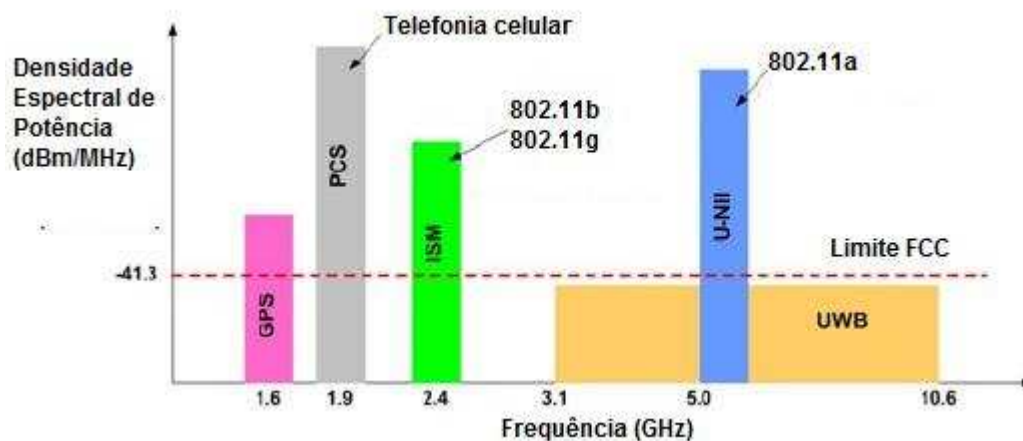
Figura 1.2 - Comparação entre espectro de sistemas disponíveis e da tecnologia UWB regulamentada pelo FCC (adaptado de [1]).
