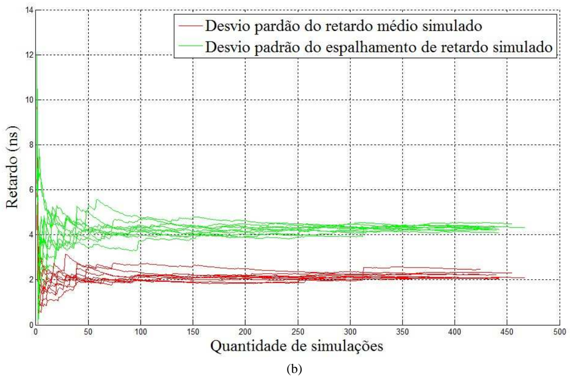
Figura 5.15 - Resultado de dez testes de convergência do modelo II para as medidas do ambiente B, através da (a) média e (b) desvio padrão do retardo médio e do espalhamento de retardo simulados.
