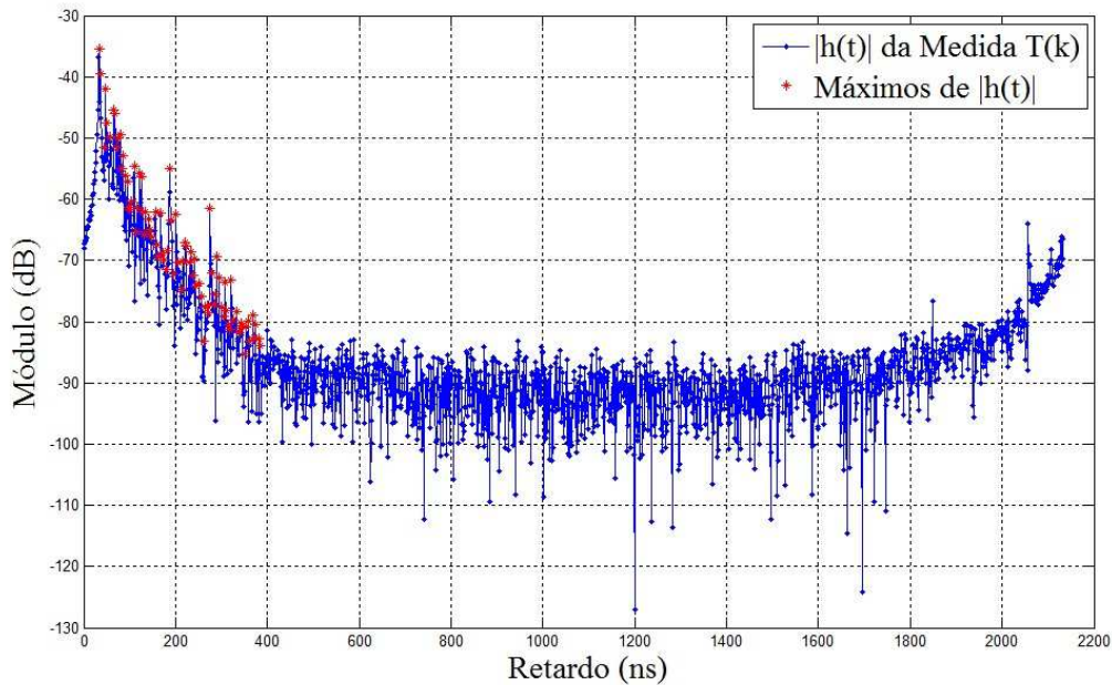
Figura 5.6 - Módulo em dB da transformada inversa de Fourier discreta da medida T(k) .
