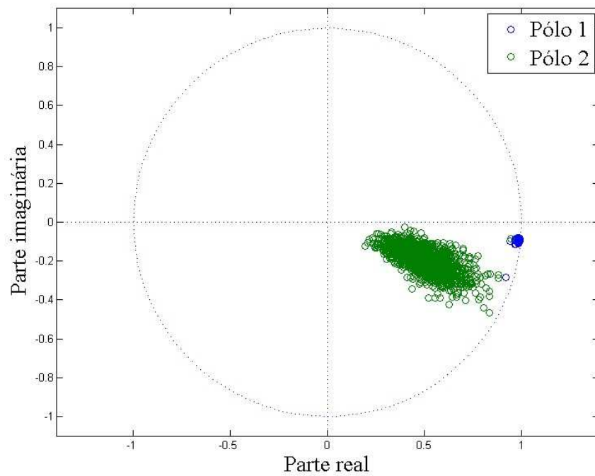
Figura 5.18 - Distribuição do conjunto de pares de pólos (1 e 2) no plano Z para sinais simulados do modelo II.
