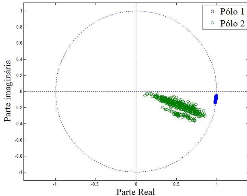
Figura 5.13 - Distribuição do conjunto de pares de pólos ( p_1 e p_2 ) no plano Z, referente aos sinais T_F(k) nos ambientes A, B e C.
