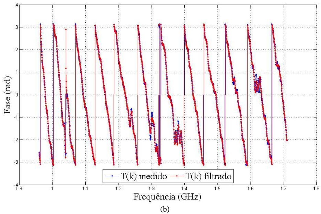
Figura 5.12 - Comparação entre uma medida T(k) e sua respectiva versão filtrada T_F(k) : (a) módulo e (b) fase.
