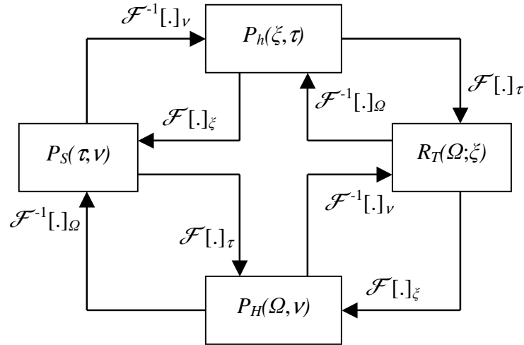
Figura 2.5 - Diagrama das funções que representam um canal WSSUS e suas respectivas relações.
