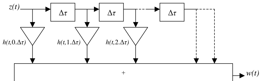
Figura 2.2 - Modelo físico do canal no domínio do tempo.
