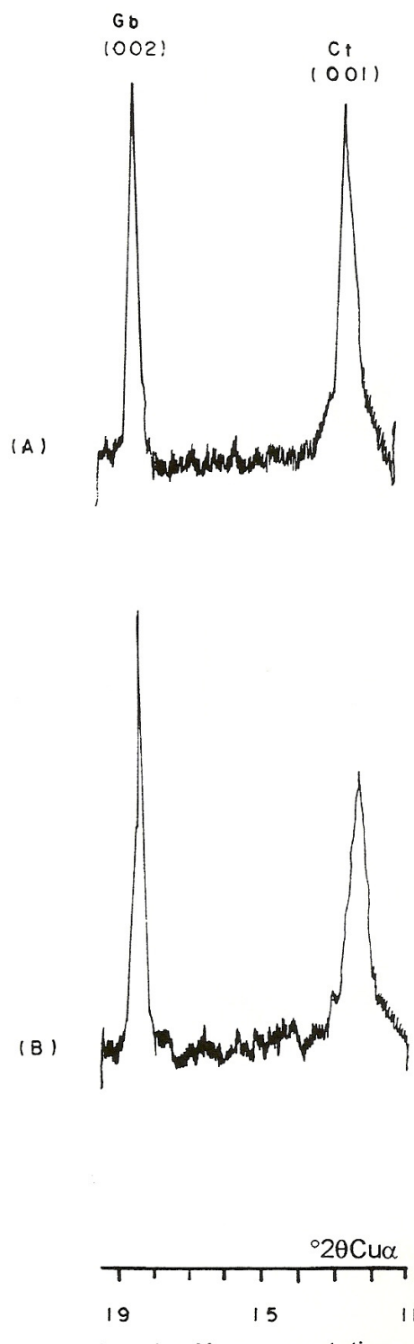
Figura 15. Difratomogramas de raios-X representativos da fração argila tratada com DCB, do solo LE-3, sob a superfície geomórfica II, para as amostras coletadas nos pontos 55 (A) e 61(B).
