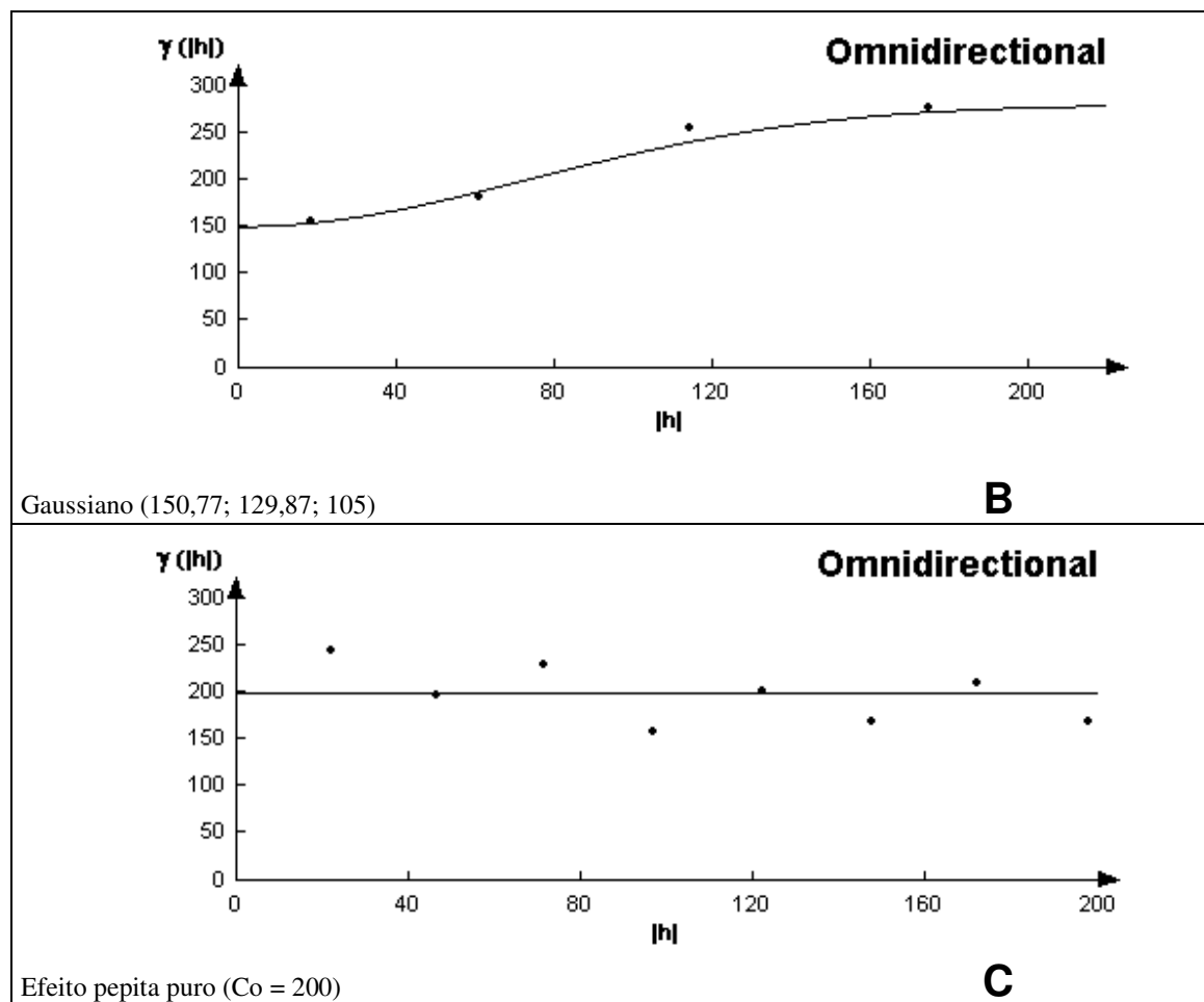
Anexo 28. Modelos dos semivariogramas ajustados para o atributo mineralógico teor de Hematita ( \text{g.kg}^{-1} ), sob as três superfícies geomórficas (A - superfície I; B - superfície II; C - superfície III), com os respectivos parâmetros.
