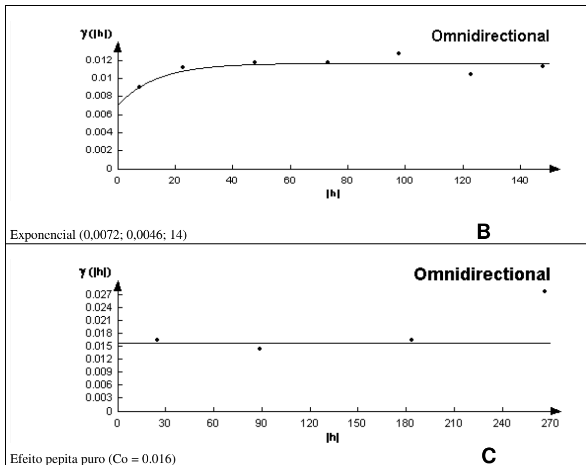
Anexo 24. Modelos dos semivariogramas ajustados para o atributo mineralógico, área do pico da Hm 012 ( \text{cm}^2 ), sob as três superfícies geomórficas (A - superfície I; B - superfície II; C - superfície III), com os respectivos parâmetros.
