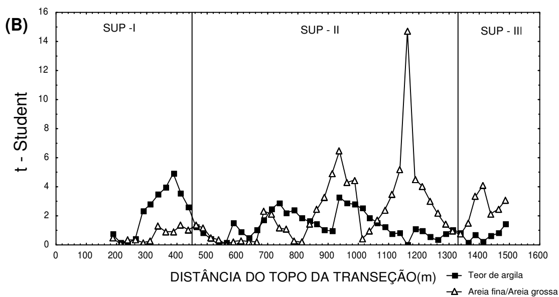
Figura 26. Resultado do "Split moving windows" para localização estatística dos atributos físicos ao longo da vertente, com pontos de coleta a cada 25 m. A – silte/argila e densidade de partículas; B – teor de argila e areia fina/areia grossa.
