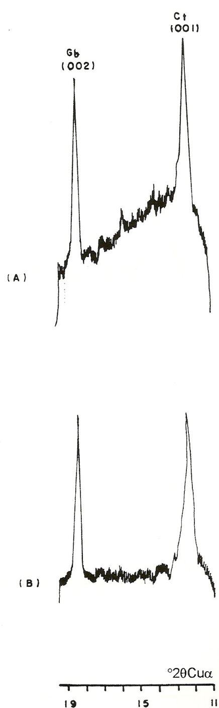
Figura 14. Difratomogramas de raios-X representativos da fração argila tratada com DCB, do solo LE-1, sob a superfície geomórfica II, para as amostras coletadas nos pontos 45(A) e 42(B).
