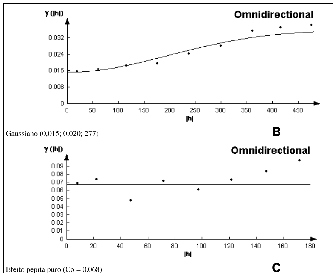
Anexo 26. Modelos dos semivariogramas ajustados para o atributo mineralógico, área do reflexo da Gb 002 (cm 2 ), sob as três superfícies geomórficas (A - superfície I; B - superfície II; C - superfície III), com os respectivos parâmetros.
