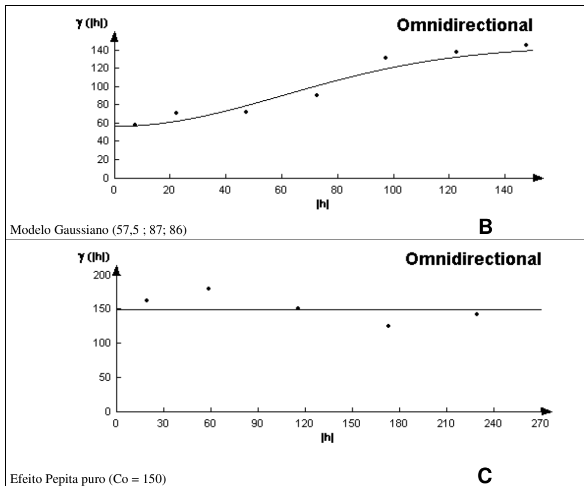
Anexo 20. Modelos dos semivariogramas ajustados para o atributo químico, Fe_d ( g.kg^{-1} ), sob as três superfícies geomórficas (A - superfície I; B - superfície II; C - superfície III), com os respectivos parâmetros.
