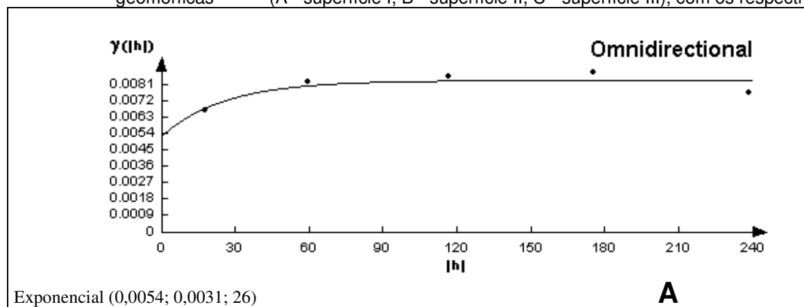
Anexo 23. Modelos dos semivariogramas ajustados para o atributo mineralógico, área do pico da Gt 110 ( \text{cm}^2 ), sob as três superfícies geomórficas (A - superfície I; B - superfície II; C - superfície III), com os respectivos parâmetros.
