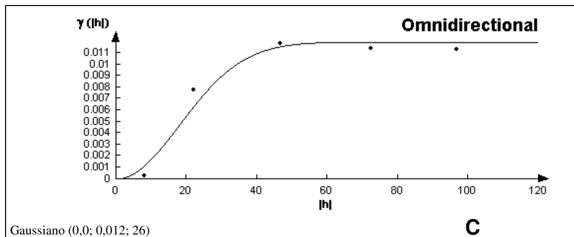
Anexo 23. Modelos dos semivariogramas ajustados para o atributo mineralógico, área do pico da Gt 110 ( \text{cm}^2 ), sob as três superfícies geomórficas (A - superfície I; B - superfície II; C - superfície III), com os respectivos parâmetros.
