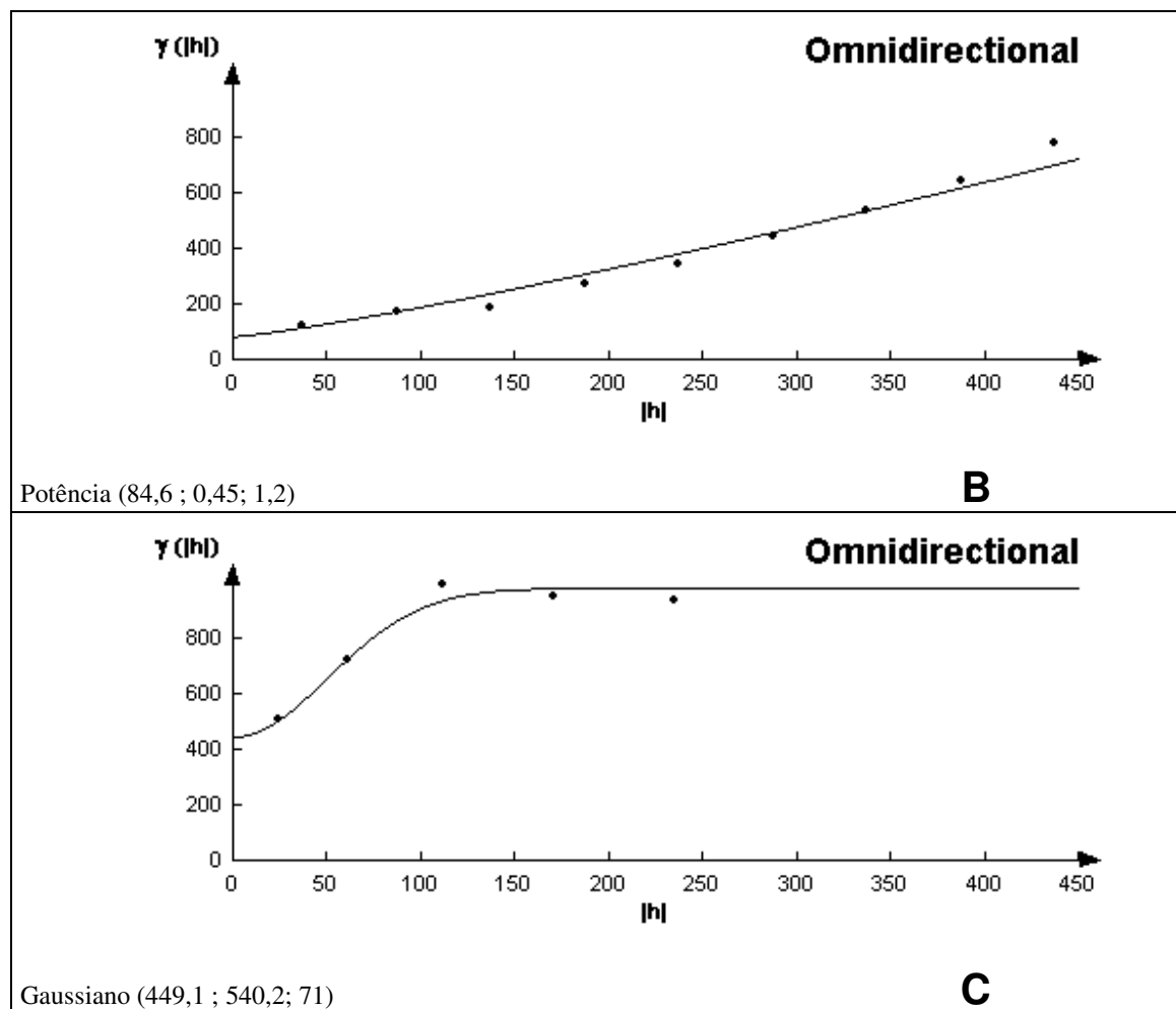
Anexo 22. Modelos dos semivariogramas ajustados para o atributo químico, Fe_s ( g.kg^{-1} ), sob as três superfícies geomórficas (A - superfície I; B - superfície II; C - superfície III), com os respectivos parâmetros.
