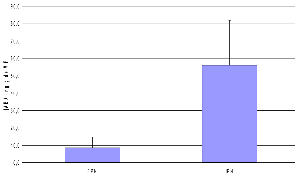
Figura 3c. Concentração média de ABA no embrião e na semente inteira de Acca sellowiana a partir de polinização natural (média \pm desvio padrão, n=3). * I-semente inteira; E-embrião; PN-polinização natural
