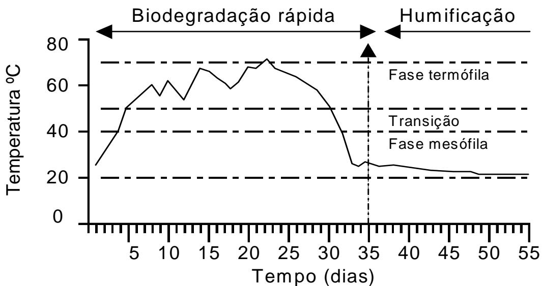
FIGURA 2.7 – CURVA PADRÃO DA VARIAÇÃO DA TEMPERATURA DURANTE O PROCESSO DE COMPOSTAGEM.
