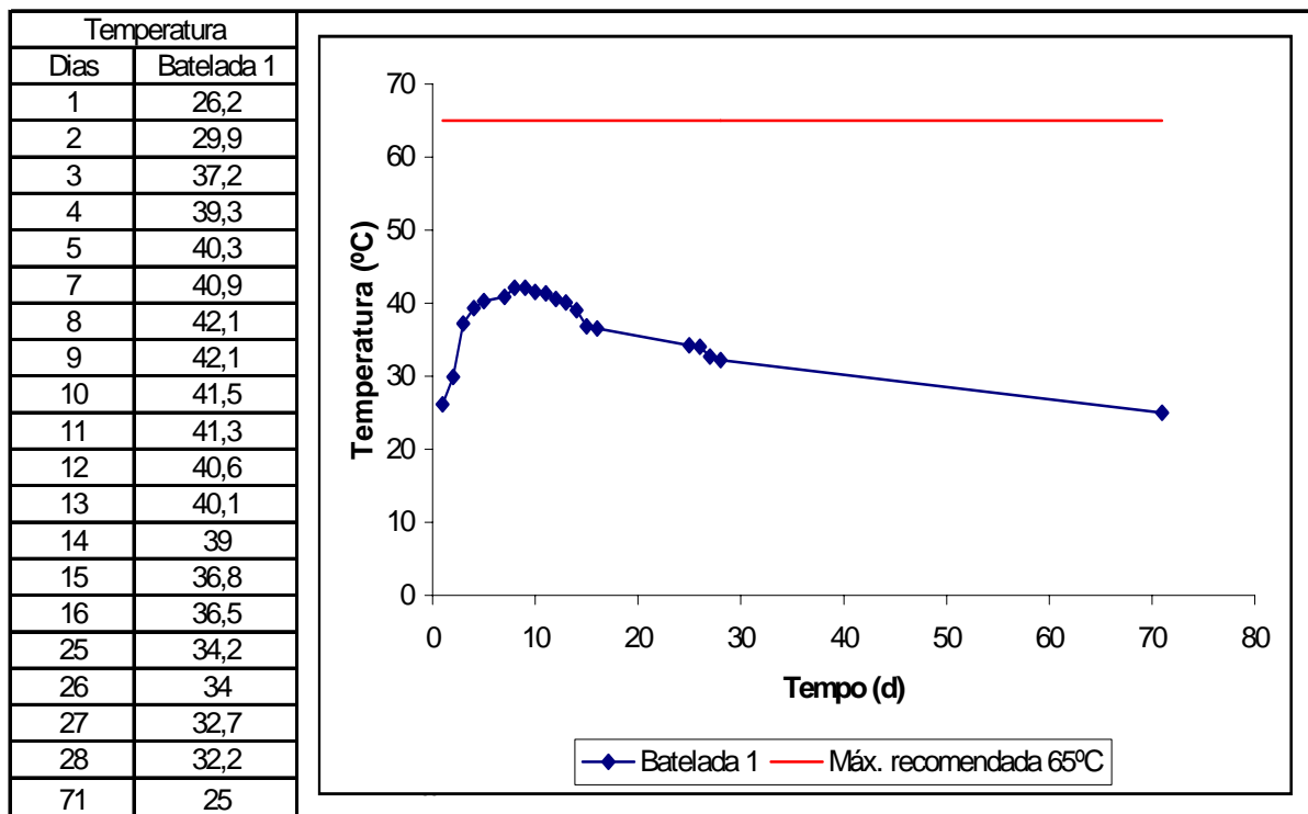
FIGURA 4.7 – VARIAÇÃO DA TEMPERATURA NA BATELADA 1
