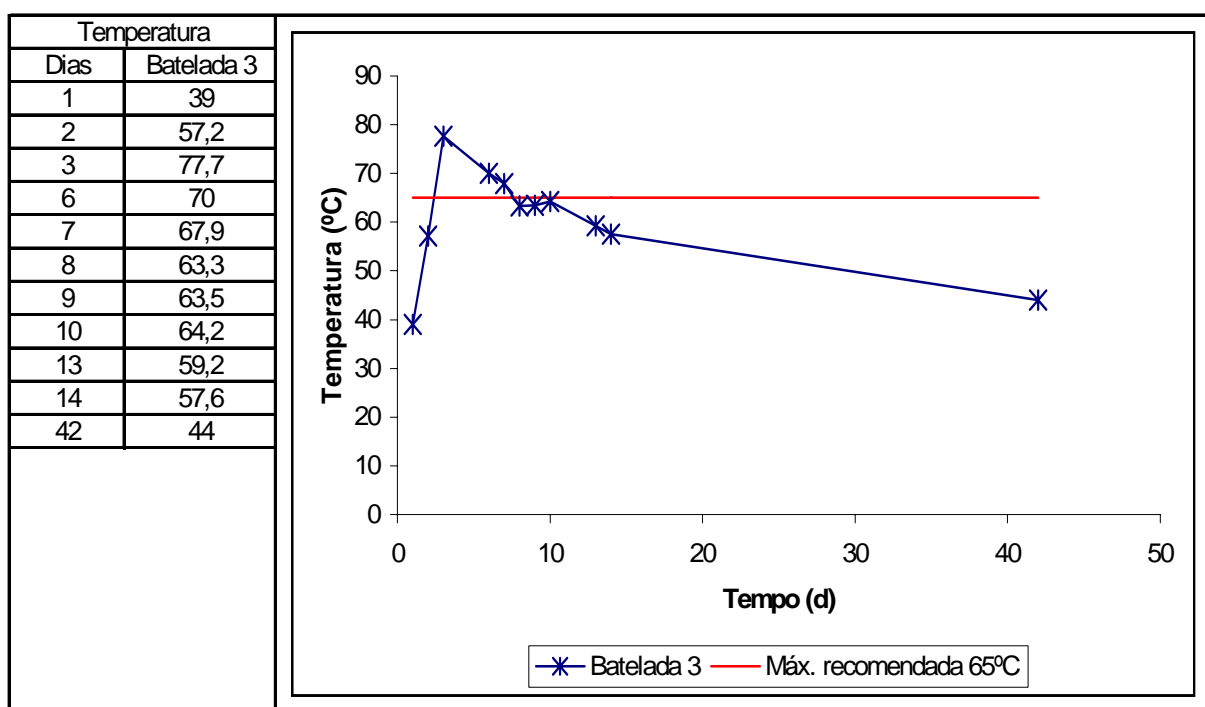
FIGURA 4.8 – VARIAÇÃO DA TEMPERATURA NA BATELADA 3
