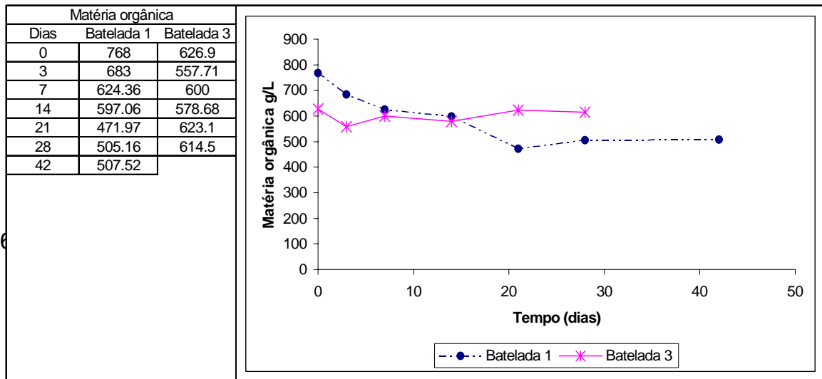
FIGURA 4.11 – VARIAÇÃO DOS SÓLIDOS VOLÁTEIS NAS BATELADAS 1 E 3
