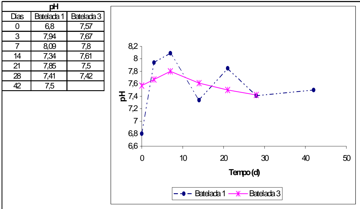
FIGURA 4.9 – VARIAÇÃO DO pH NAS BATELADAS 1 E 3.
