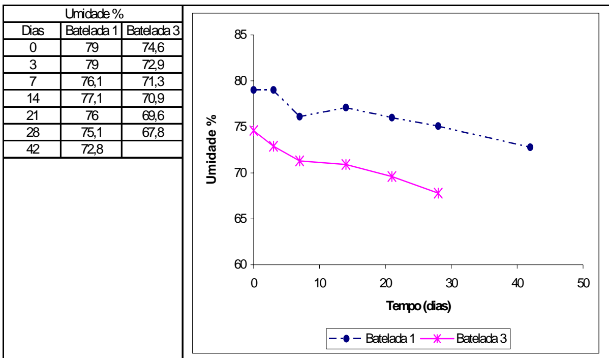
FIGURA 4.5 – VARIACÃO DA UMIDADE NAS BATELADAS 1 E 3
