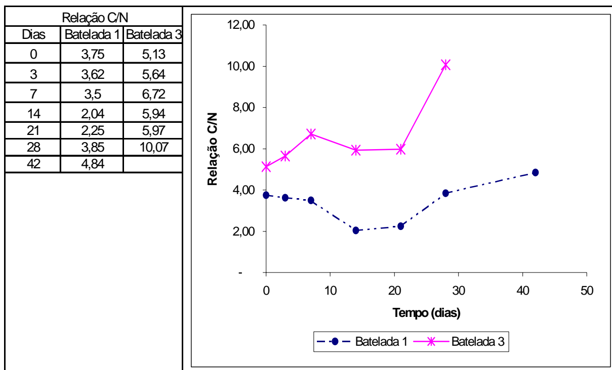
FIGURA 4.6 – VARIAÇÃO DA RELAÇÃO CARBONO / NITROGÊNIO NAS BATELADAS 1 E 3
