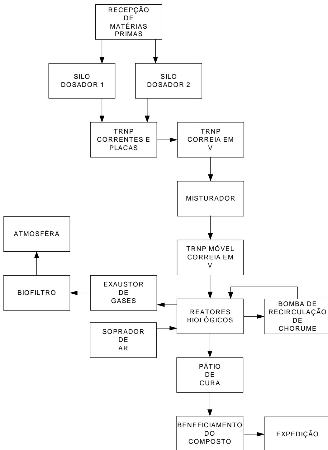
FIGURA 3.4 - FLUXOGRAMA DA UNIDADE
