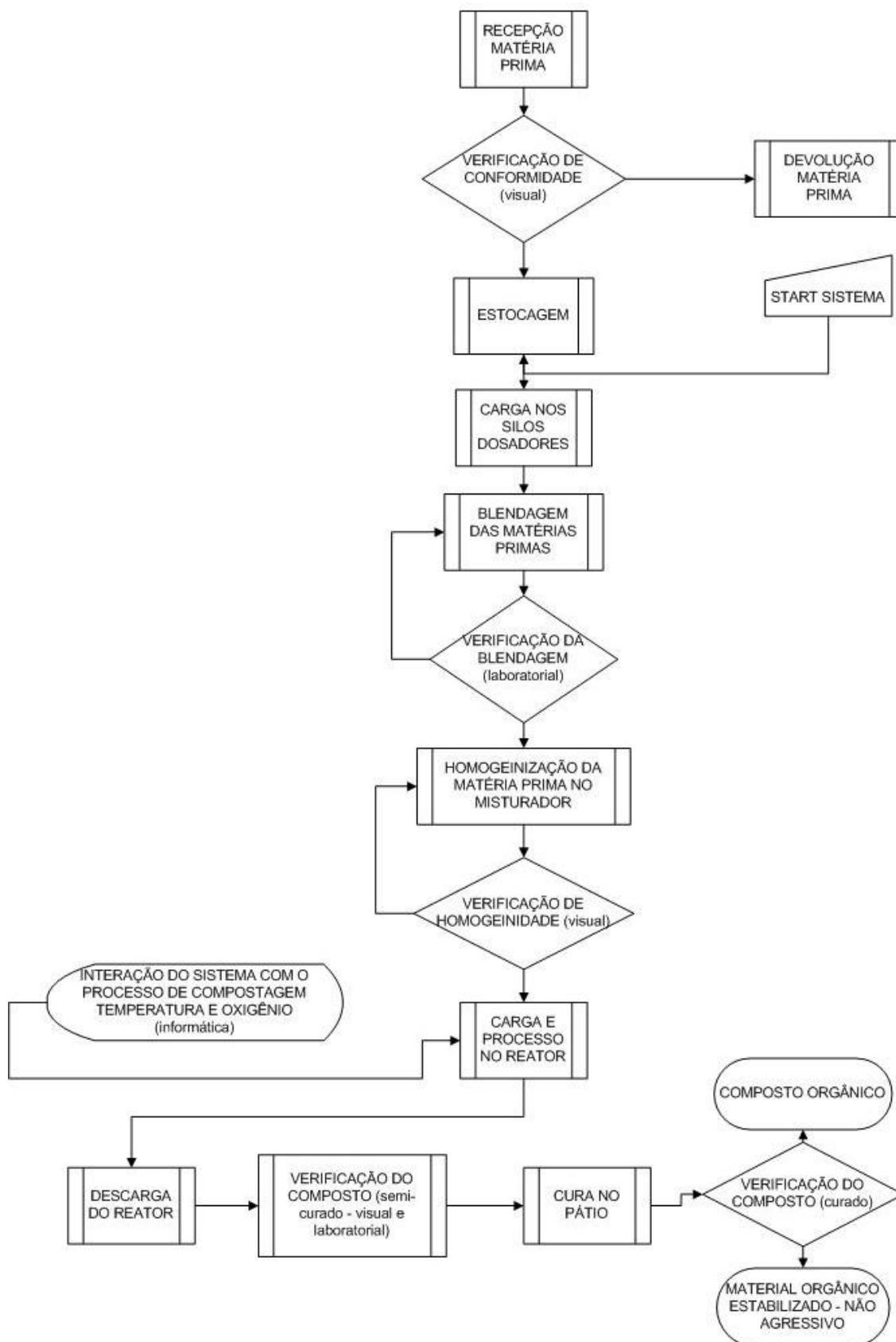
FIGURA A.4.1. – FLUXOGRAMA DO CONTROLE DE QUALIDADE E DO PROCESSO
