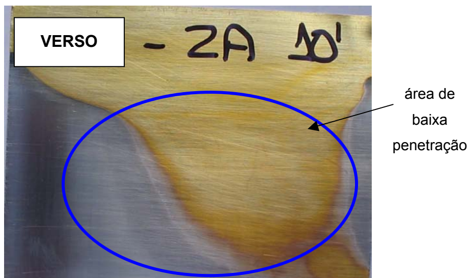
Figura 4.14 – PAINEL TÍPICO OBTIDO EM CÉLULA DE HULLL - VERSO
