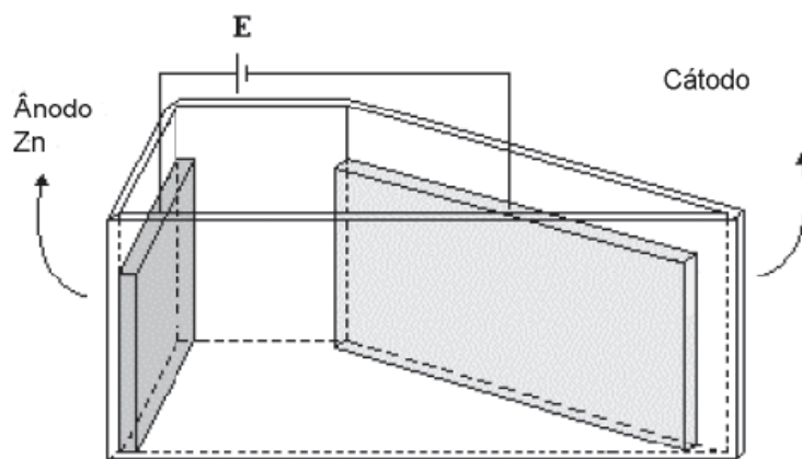
Figura 3.3 – DIAGRAMA ESQUEMÁTICO DA CÉLULA DE HULL.
