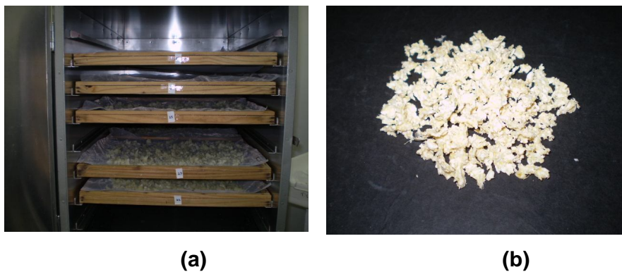
Figura 6 – Ilustração do processo de secagem do mesocarpo triturado em secador de bandejas (a) para obtenção do material desidratado (b).
