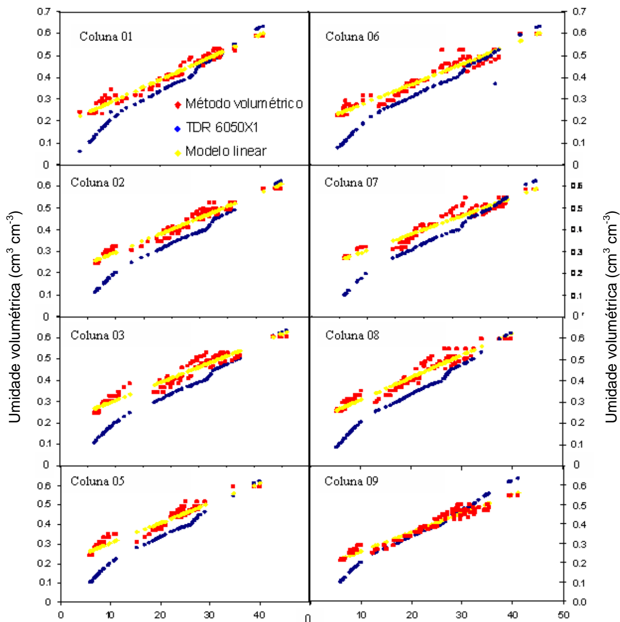
Figura 13 - Gráfico de dispersão da constante dielétrica, fornecida pelo equipamento TDR versus umidade pelo método volumétrico, modelo embutido no equipamento TDR e modelo ajustada para colunas
