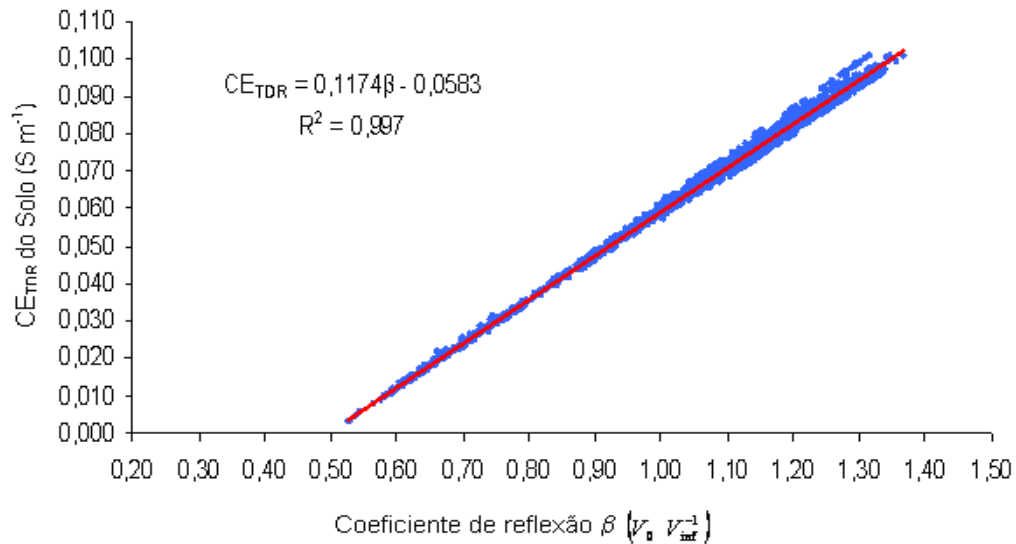
Figura 15 – Modelo de regressão entre condutividade elétrica do solo e coeficiente de reflexão \beta .
