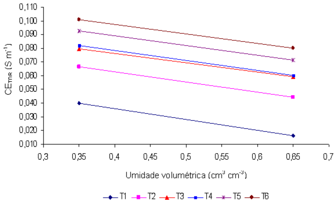
Figura 16 - Correlação entre condutividade elétrica do solo pelo método da TDR e umidade volumétrica do solo
