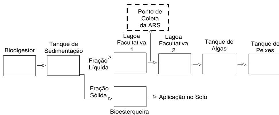
Figura 9 - Ponto de coleta da água residuária de suinocultura no biosistema integrado.
