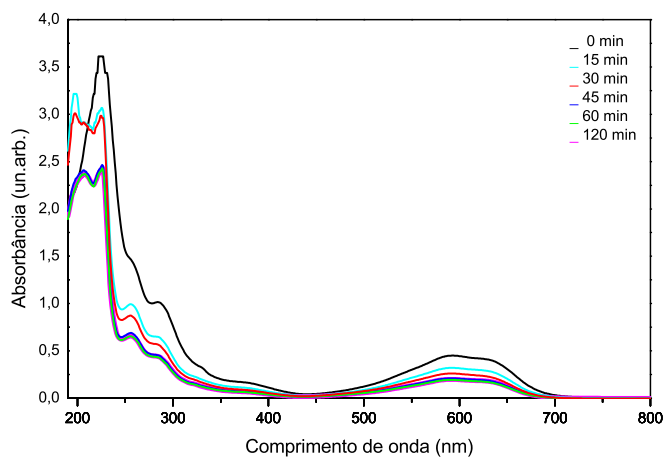
Figura 31: Espectro de absorção no UV-Vis do corante têxtil azul reativo 19 após degradação com luz solar simulada utilizando o Ce-NTTi como agente fotocatalisador.
