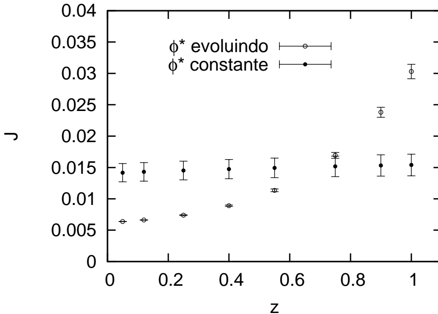
Figura 3.8: Função de completudeza para dados de todas as galáxias no catálogo de L99 baseado no levantamento CNO2, na parametrização com \phi^* constante usada em RS03 e levando em consideração o modelo de evolução da FL completo proposto em L99. Aqui fica ainda mais explícita a dependência com o parâmetro \phi^* da evolução da densidade numérica e portanto da inconsistência entre os dados desse catálogo e a teoria para as contagens.
