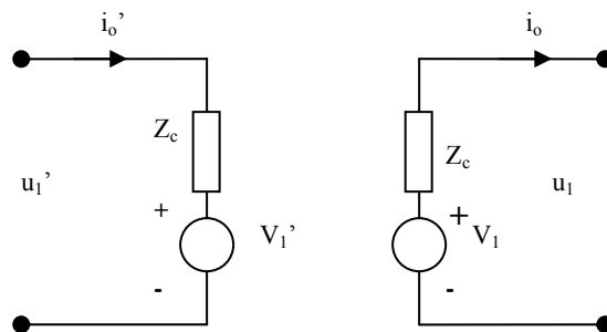
Figura 3.12 - Circuito Equivalente de uma Linha Curta sem Perdas de Acordo com o Método de Bergeron (Representação de Thevenin).
