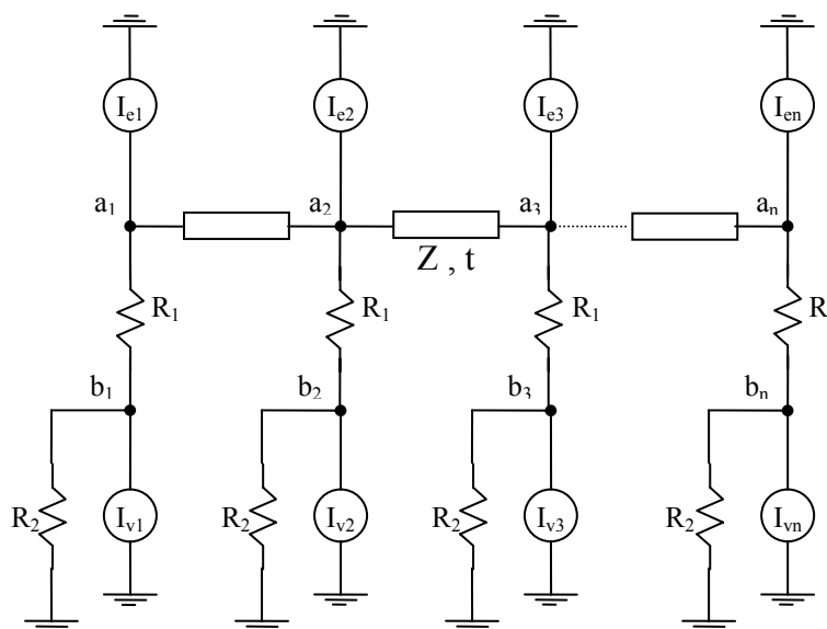
Figura 3.2 - Fontes de Corrente na Implementação do EMTP (Fonte: Adaptado de RUSCK, 1958)
