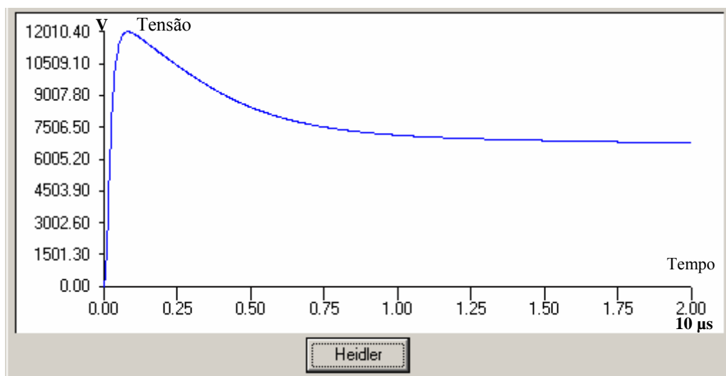
Figura 4.6 - Fonte de descarga atmosférica do tipo Heidler
