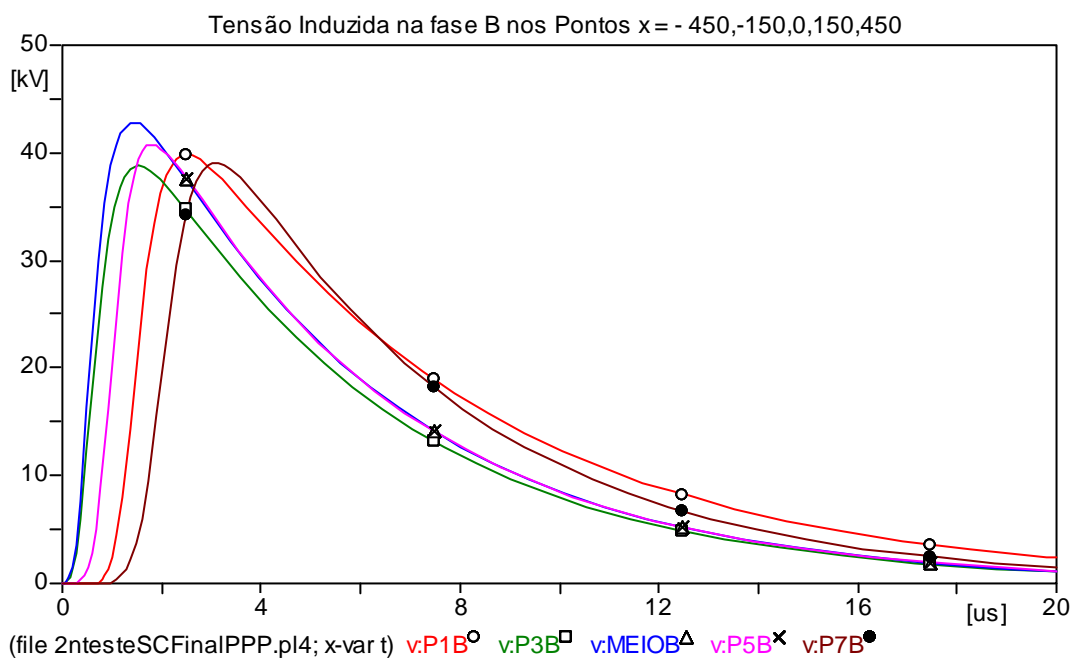
Figura 5.18 - Tensões induzidas nas Fases A, B, C para diversas posições.
