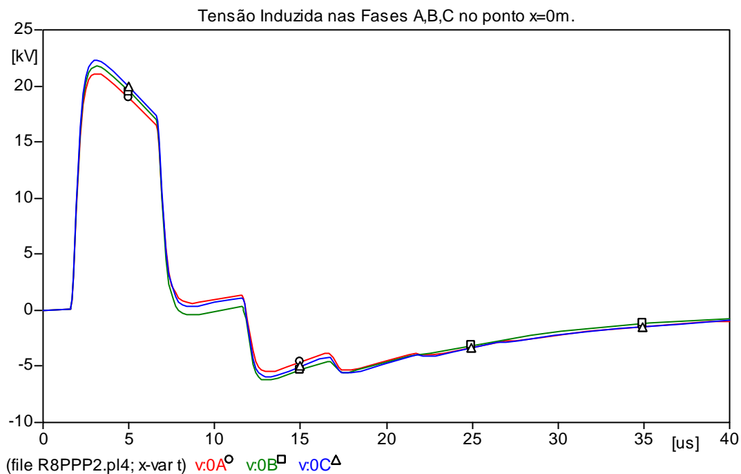
Figura 5.29 - Tensões induzidas nas fases A, B, C para um ponto x = 0m .
