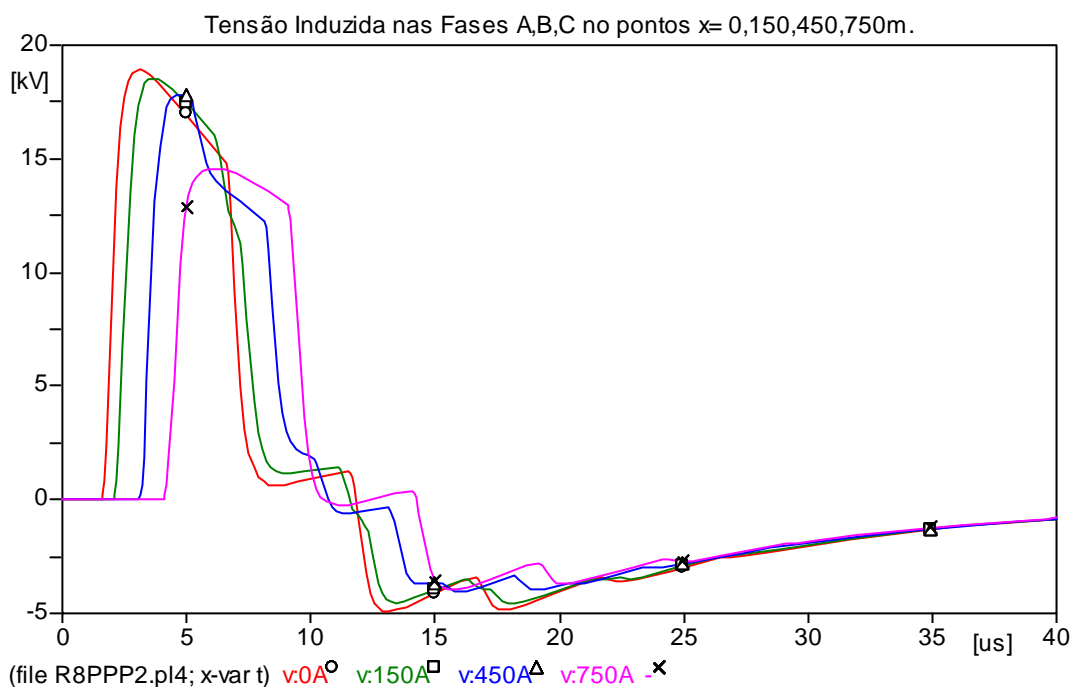
Figura 5.22 - Tensões induzidas nas fases A, B, C para um ponto x = 0, 150, 450, 750\text{m} .
