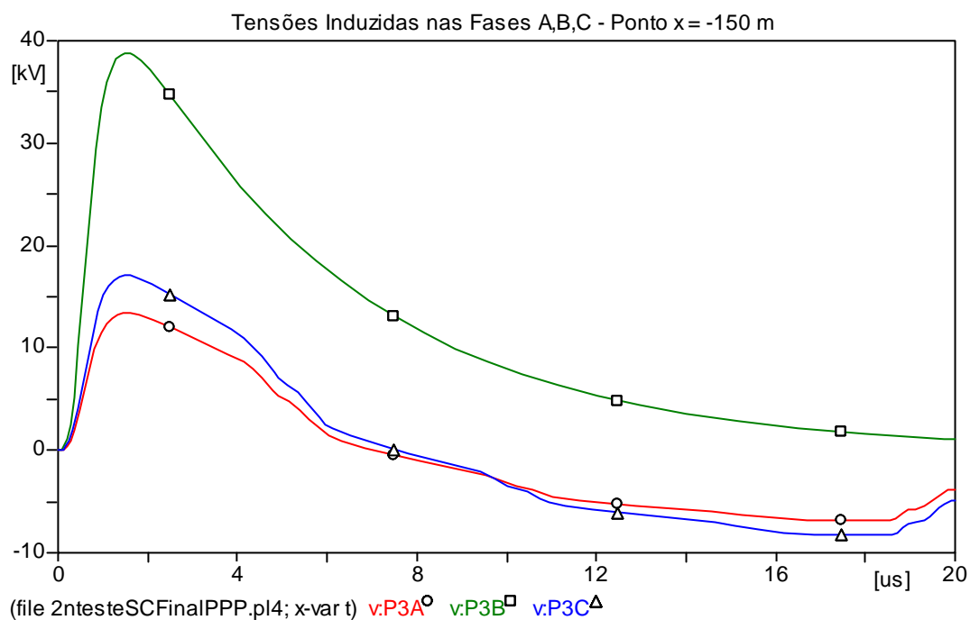
Figura 5.16 - Tensões induzidas nas fases A, B, C para um ponto x=-150 m.
