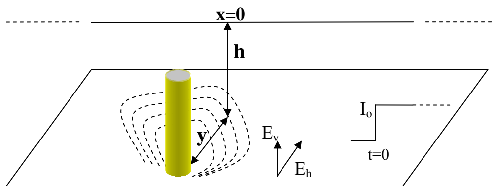
Figura 4.4 - Modelo de Rusck para Tensões Induzidas (Fonte: Adaptado de RUSCK, 1968)
