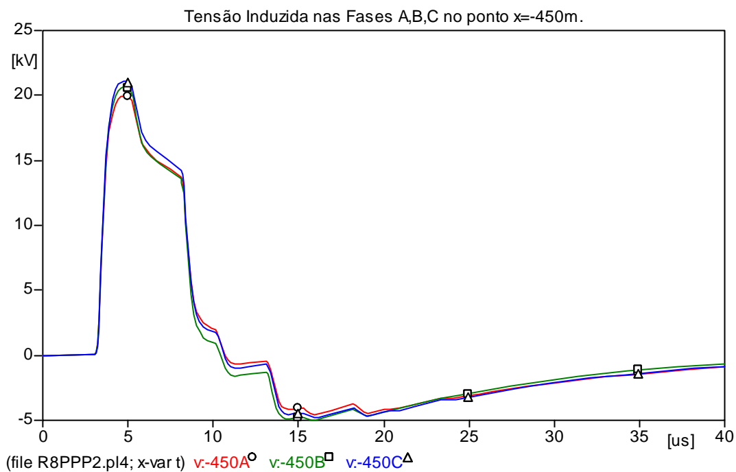
Figura 5.27 - Tensões induzidas nas fases A, B, C para um ponto x = -450m .
