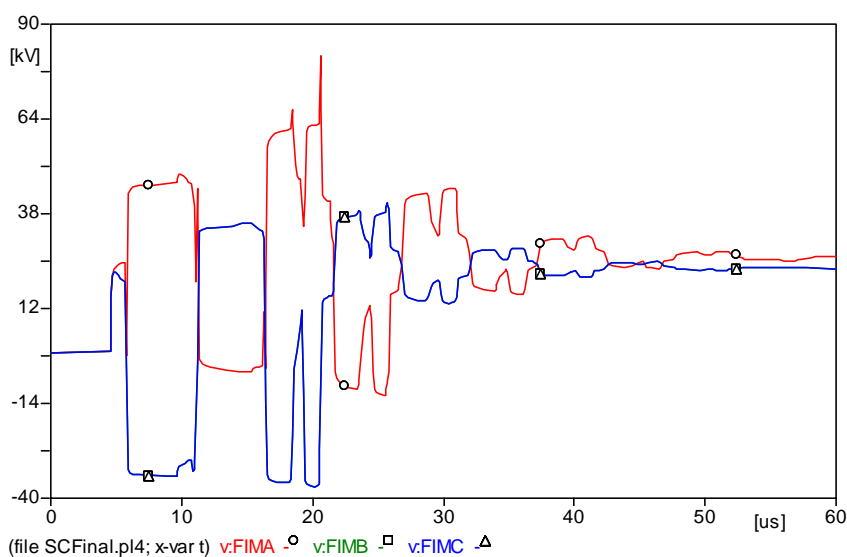
Figura 5.9 - Tensão nas Fases após a Atuação do Pára-Raio.
