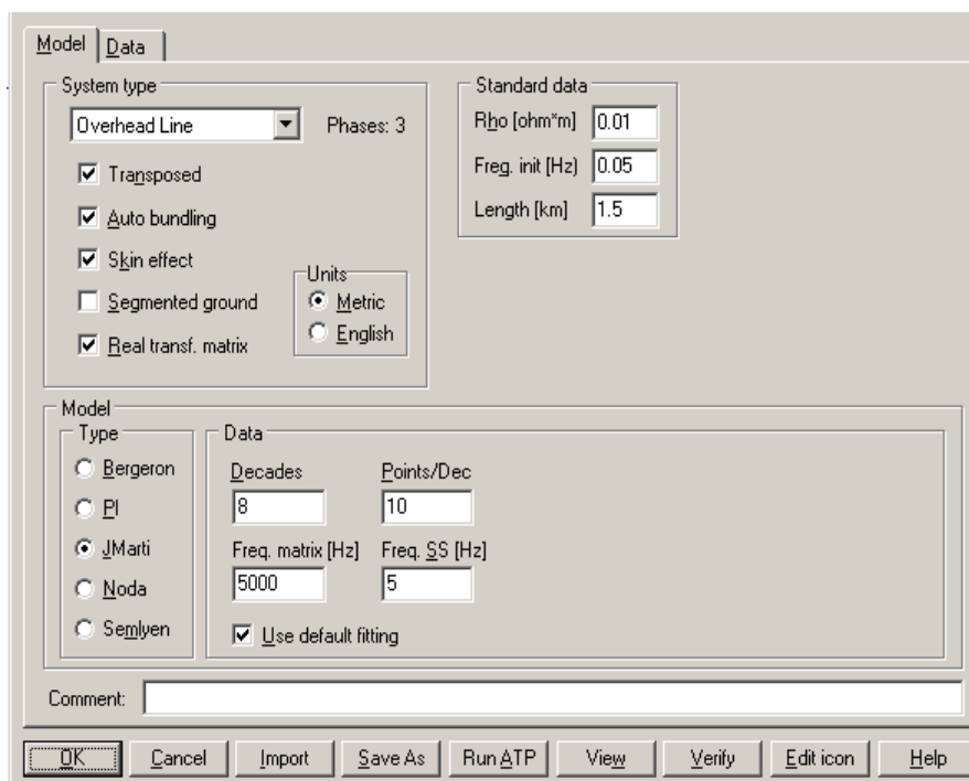
Figura 5.3 - Dados Construtivos da Linha simulada. (Fonte: ATPDraw versão 3.6p2)
