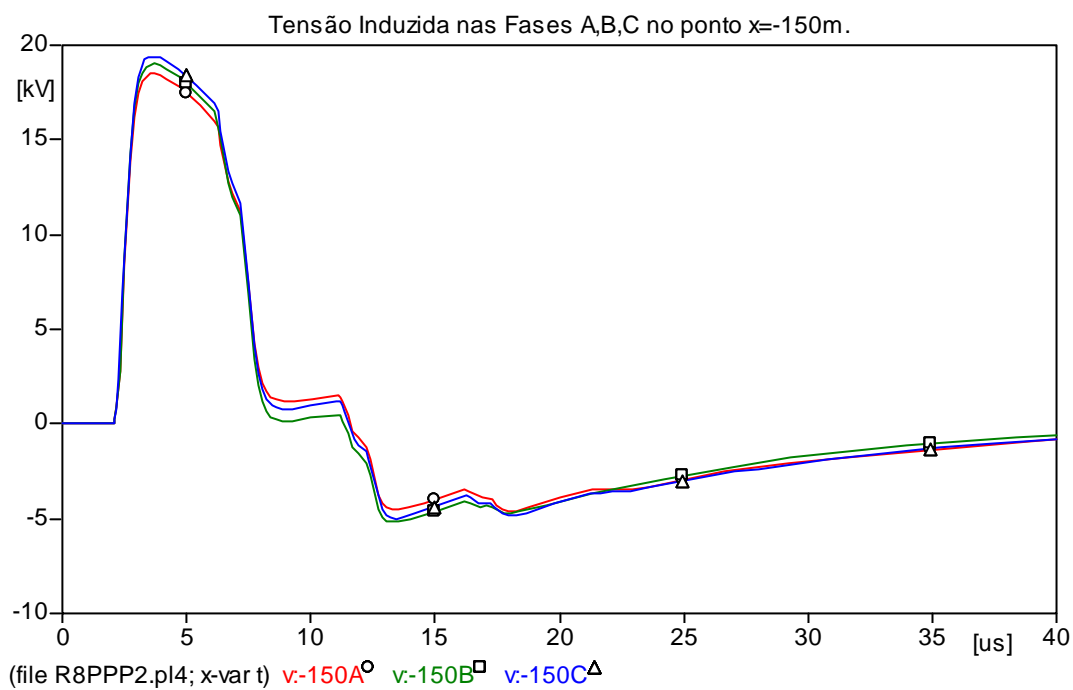
Figura 5.20 - Tensões induzidas nas fases A, B, C para um ponto x = -150m .
