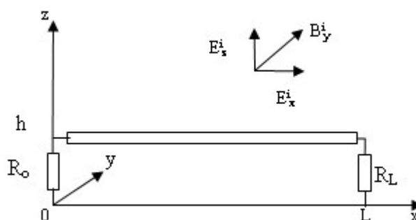
Figura 3.7 - Geometria Usada para o Cálculo da Sobretensão Induzida.
