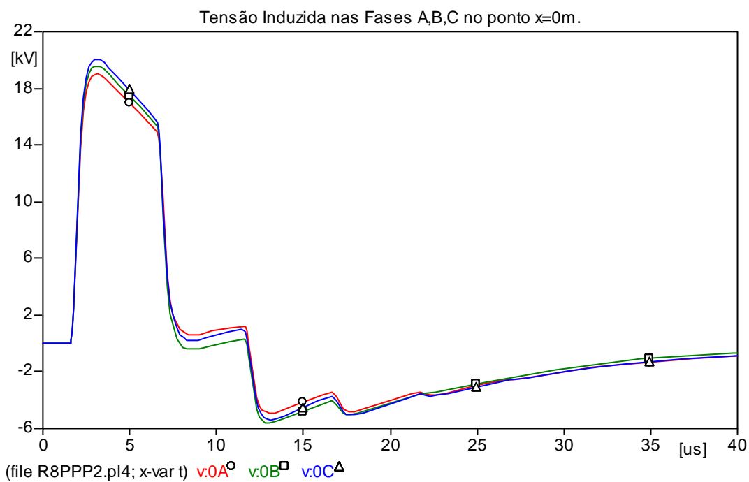
Figura 5.25 - Tensões induzidas nas fases A,B,C para um ponto x =0m.
