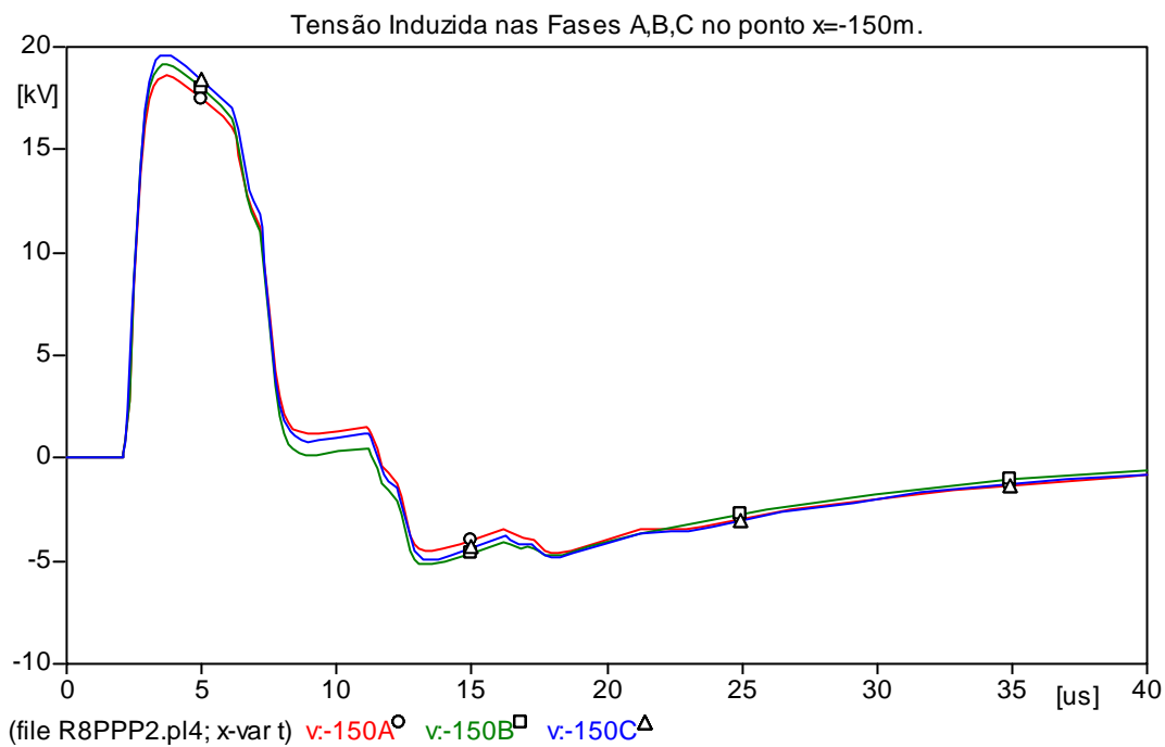
Figura 5.24 - Tensões induzidas nas fases A, B, C para um ponto x =-150m.
