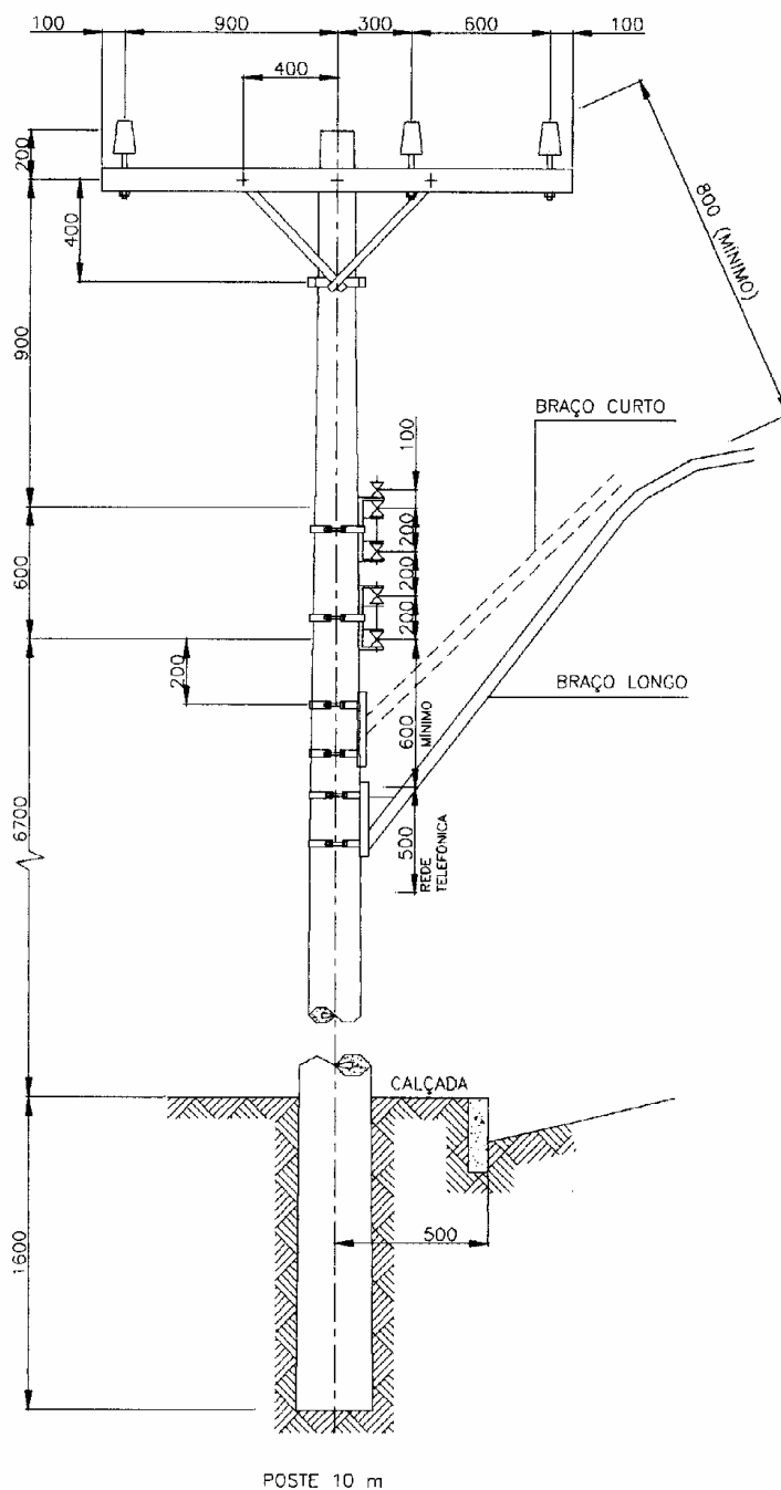
Figura 5.1 - Estrutura Padronizada para Simulação da Linha de Distribuição. (Fonte: CLFSC, 2003)
