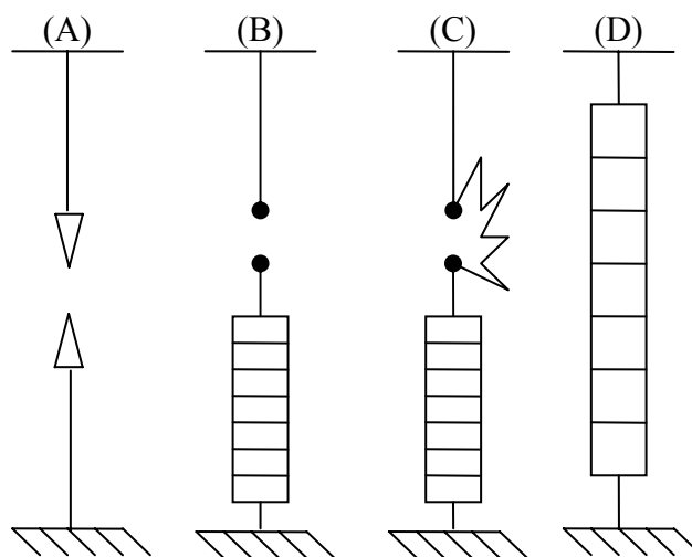
Figura 3.15 - Evolução dos Dispositivos de Proteção Contra Sobretensões.
