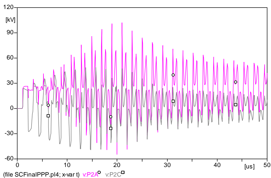
Figura 5.11 - Tensão no Ponto "2" para o Circuito 2.
