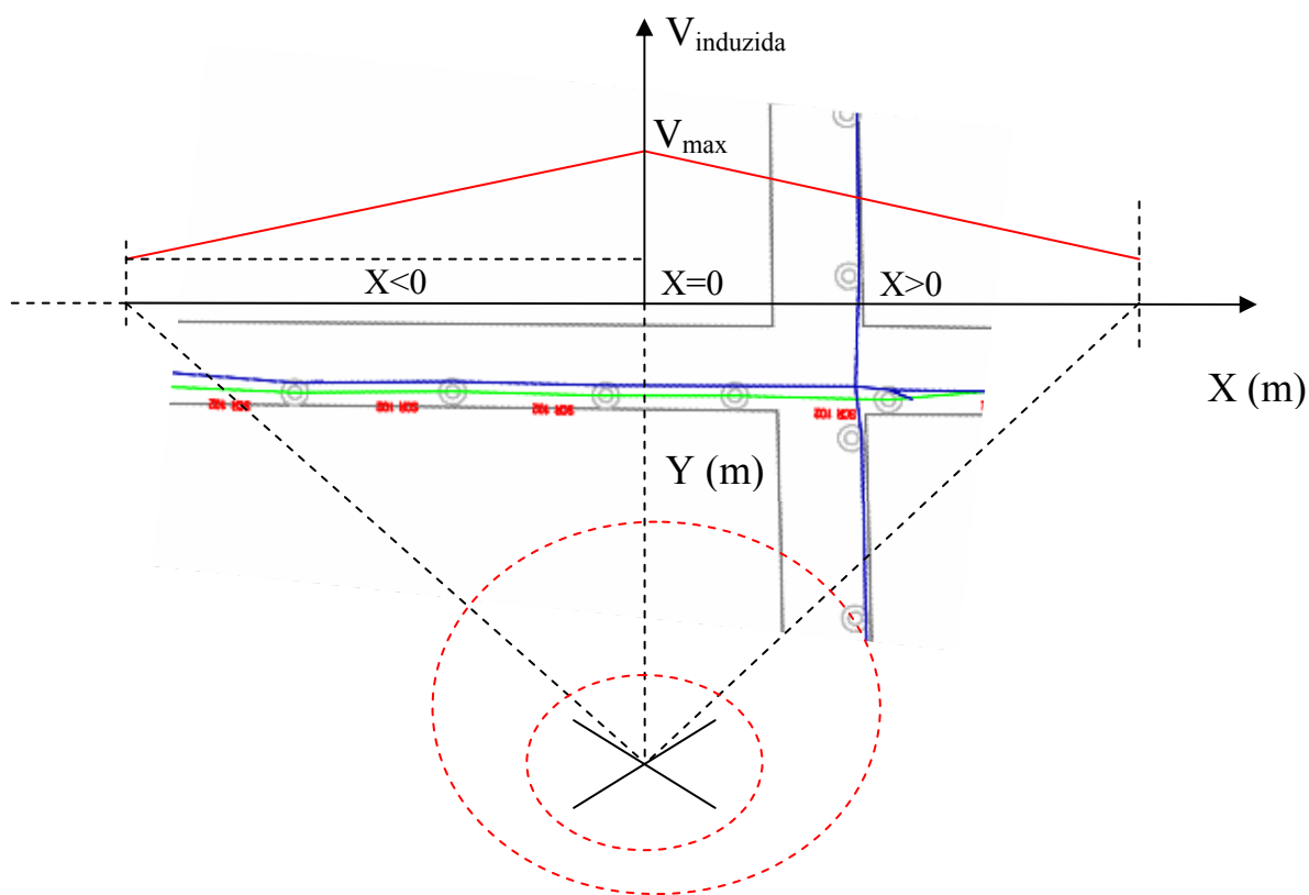
Figura 4.13 - Análise das tensões induzidas na linha (impedância casada nas extremidades)
