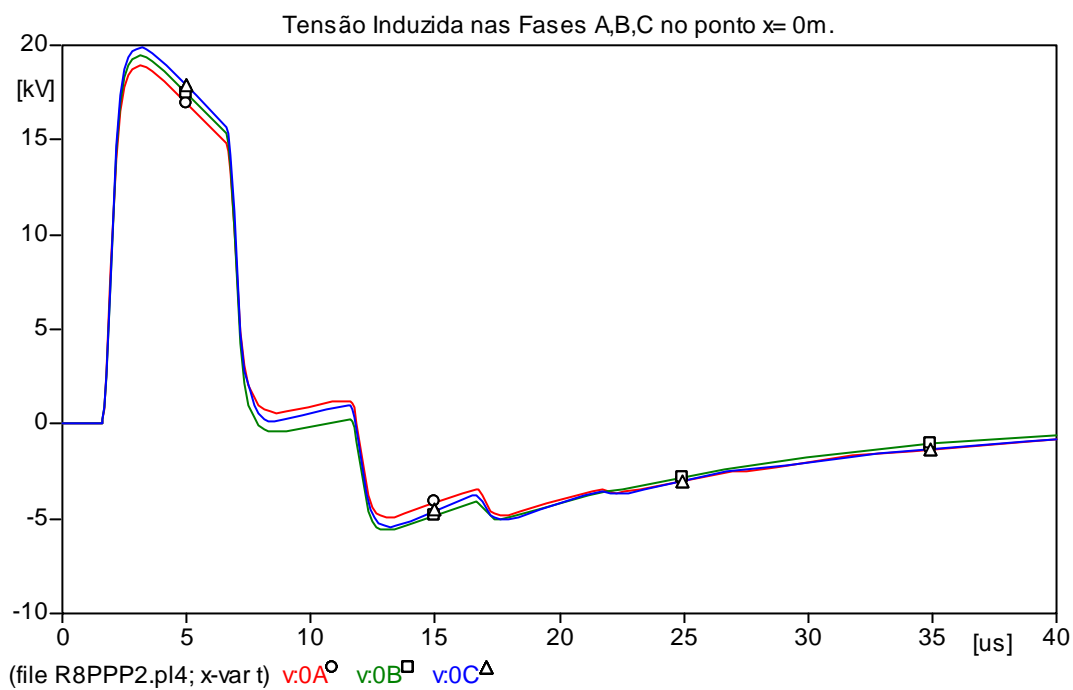
Figura 5.21 - Tensões induzidas nas fases A, B, C para um ponto x = 0m .
