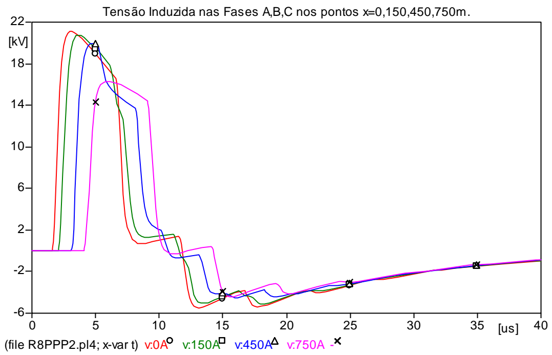
Figura 5.30 - Tensões induzidas nas fases A, B, C para um ponto x = 0, 150, 450, 750m .
