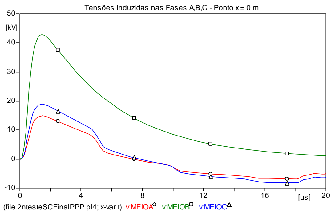
Figura 5.17 - Tensões induzidas nas fases A,B,C para um ponto x=0 m.
