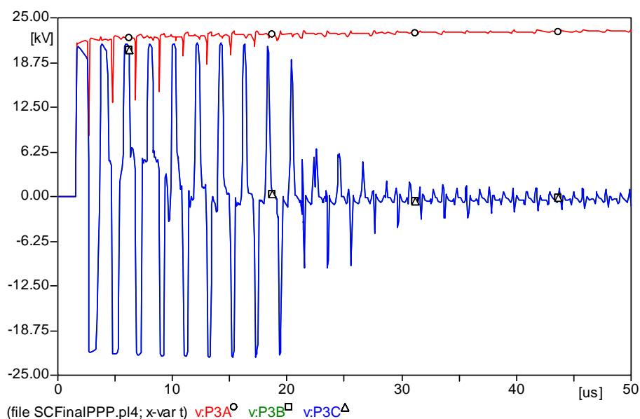
Figura 5.12 - Tensão no Ponto “3” para o Circuito 2.
