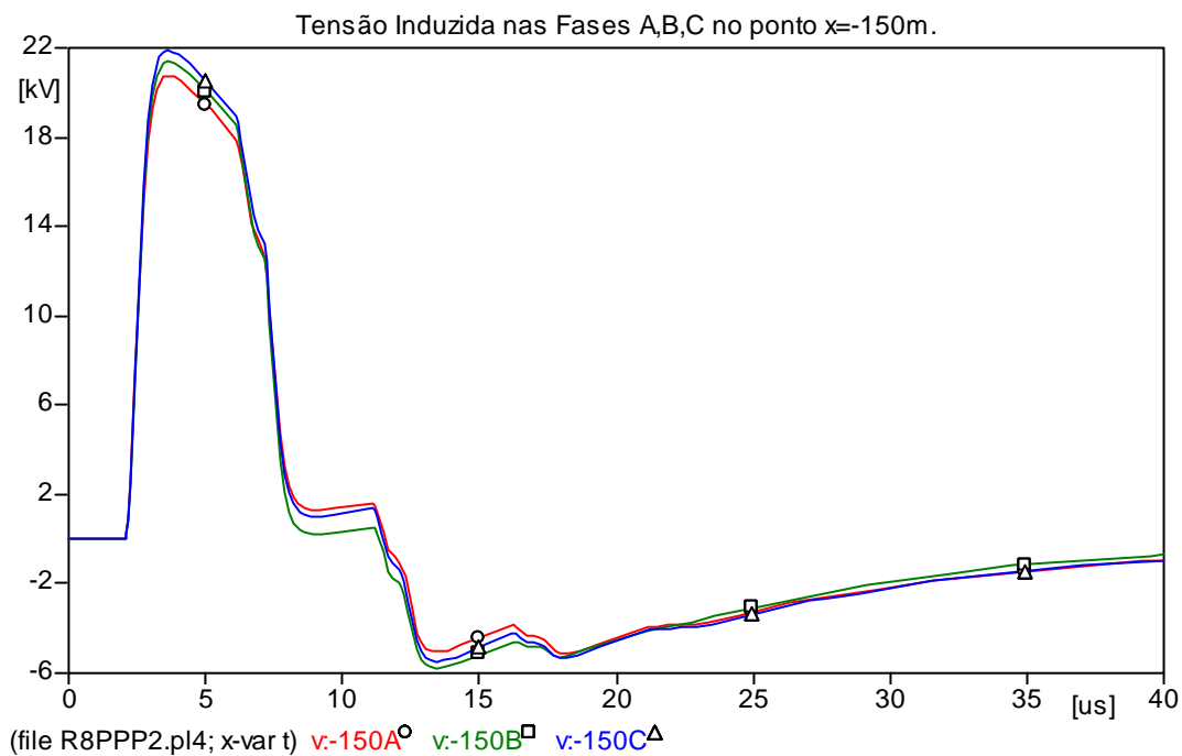
Figura 5.28 - Tensões induzidas nas fases A, B, C para um ponto x = -150m .
