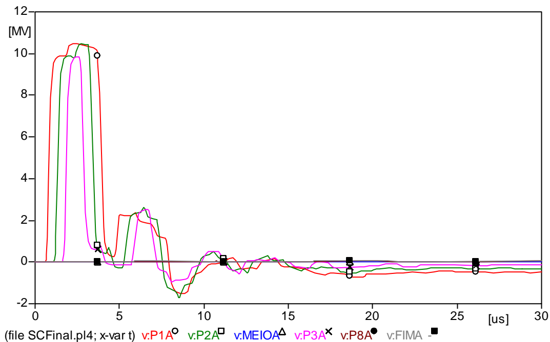
Figura 5.7 - Propagação da Onda de Sobretensão na Linha.
