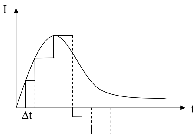
Figura 4.5 - Representação da Forma de Onda da Corrente por uma Sucessão de Degraus
