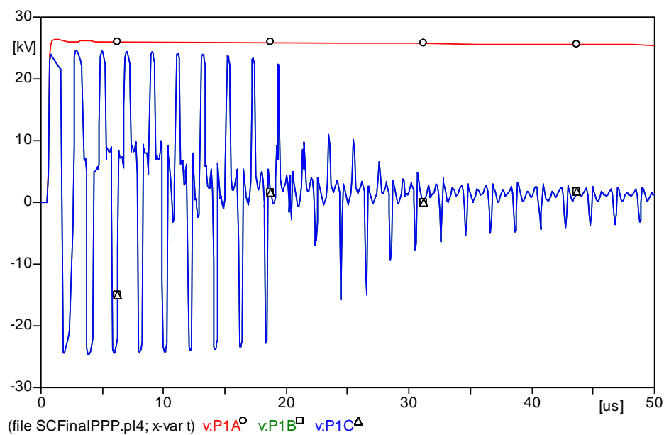
Figura 5.10 - Tensão no Ponto "1" para o Circuito 2.
