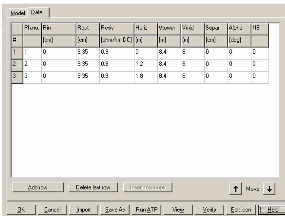
Figura 5.4 - Dados da Linha e Cabo de Distribuição. (Fonte: ATPDraw versão 3.6p2)
