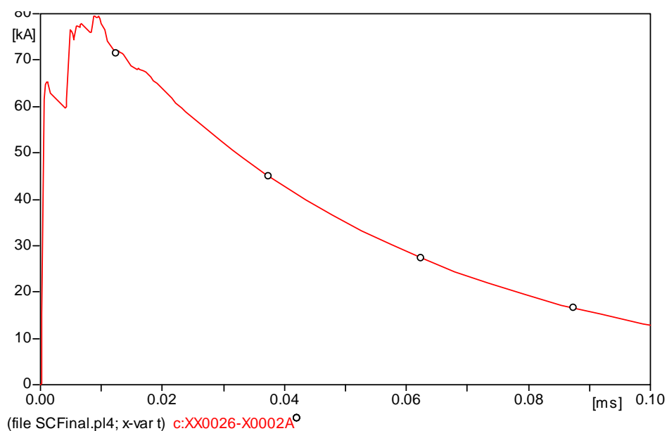
Figura 5.6 - Corrente Gerada pela Descarga.
