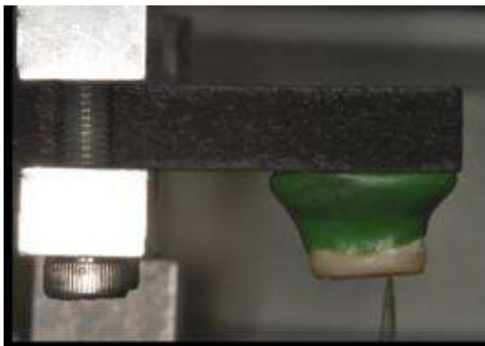
Figura 10 - Fixação dos espécimes no dispositivo de corte
