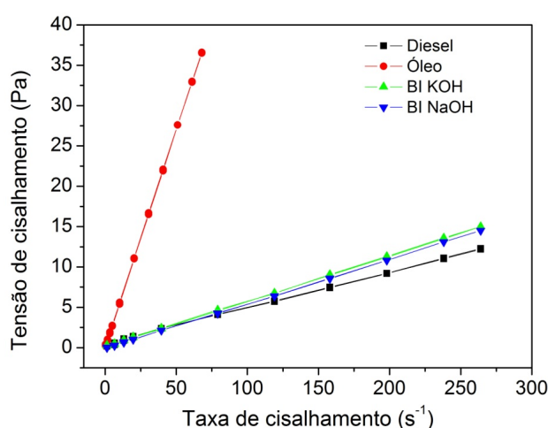
Figura 5.6: Relação entre Tensão de cisalhamento e Taxa de cisalhamento. As amostras apresentaram um comportamento Newtoniano.
