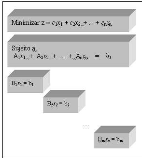
Figura 2.2: Estrutura Bloco-Angular.
