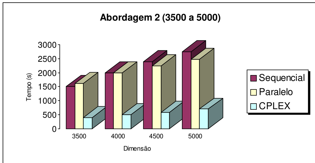
Gráfico 4.4b: Tempos médios de execução obtidos nos testes da abordagem 2 (DW Sequencial usando o CPLEX para resolver subproblemas x CPLEX) para problema de dimensão entre 3500 e 5000.
