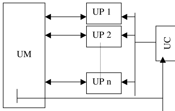
Figura 3.2: Arquitetura SIMD (UC = Unidade de Controle, UP = Unidade de Processamento, UM = Unidade de Memória)
