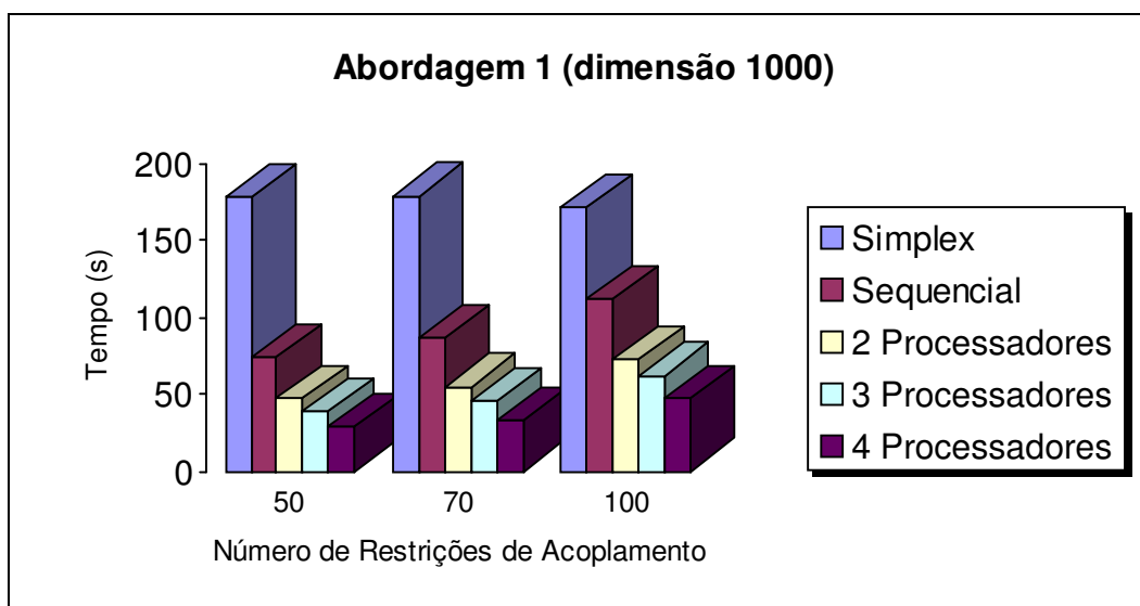
Gráfico 4.1: Tempos médios de execução obtidos nos testes da abordagem 1 (algoritmo paralelo x algoritmo sequencial) para problema de dimensão 1000.
