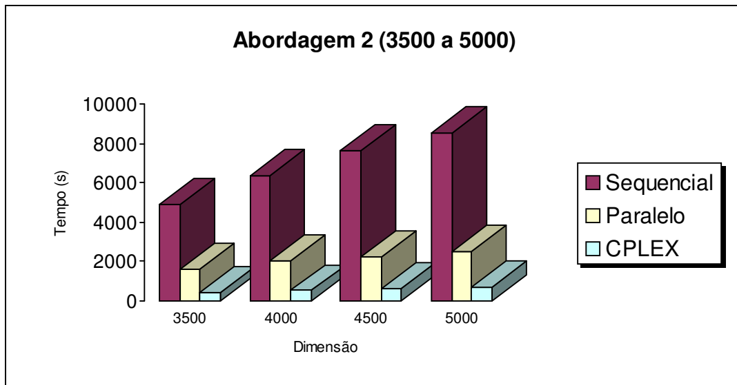
Gráfico 4.3b: Tempos médios de execução obtidos nos testes da abordagem 2 (DW em paralelo x CPLEX) para problema de dimensão entre 3500 e 5000.
