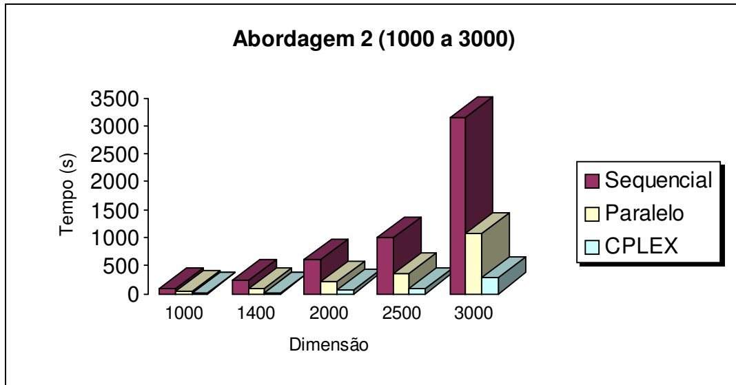
Gráfico 4.3a: Tempos médios de execução obtidos nos testes da abordagem 2 (DW em paralelo x CPLEX) para problema de dimensão entre 1000 e 3000.
