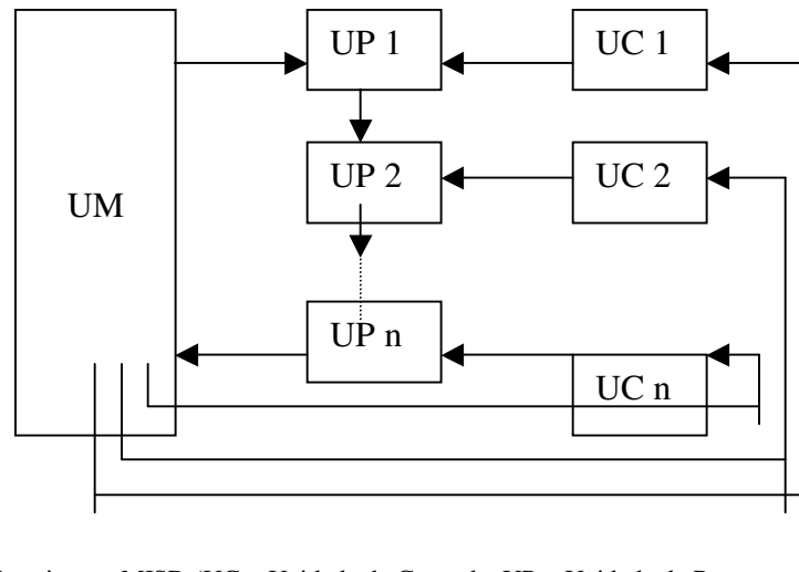
Figura 3: Arquitetura MISD (UC = Unidade de Controle, UP = Unidade de Processamento, UM = Unidade de Memória)
