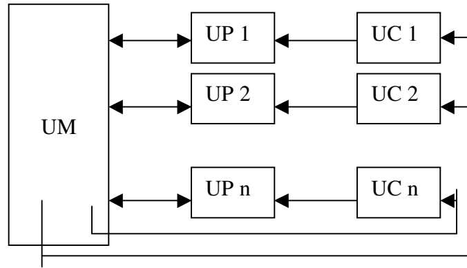
Figura 3.4: Arquitetura MIMD (UC = Unidade de Controle, UP = Unidade de Processamento, UM = Unidade de Memória)
