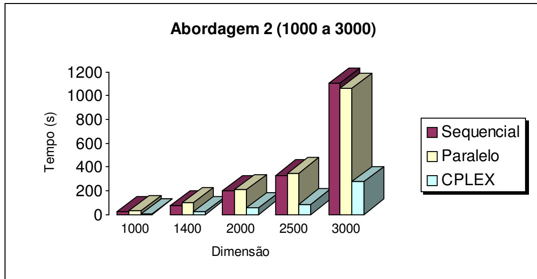
Gráfico 4.4a: Tempos médios de execução obtidos nos testes da abordagem 2 (DW Sequencial usando o CPLEX para resolver subproblemas x CPLEX) para problema de dimensão entre 1000 e 3000.
