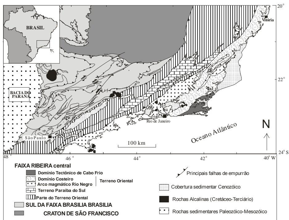
Figura 03. Mapa tectônico da região Sudeste do Brasil, com destaque para a Faixa Ribeira. (Trouw et.al., 2000)
