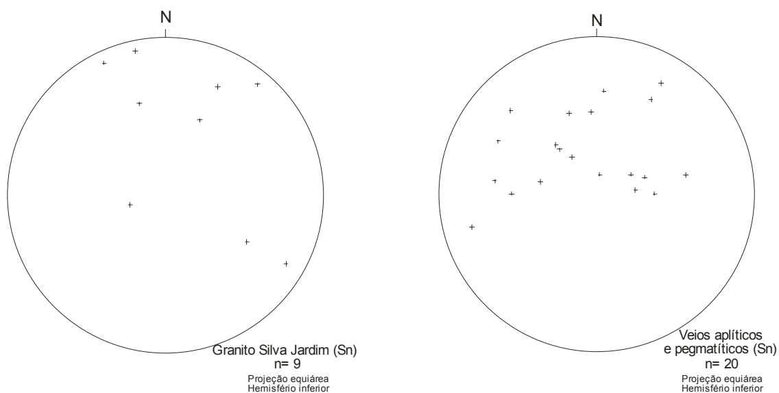
Figura 26. Estereogramas mostrando a distribuição dos pólos da foliação de fluxo do granito Silva Jardim e os planos dos veios tardios, respectivamente.
