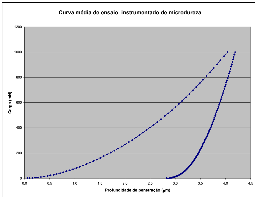
FIGURA 22b: Grupo II – Amostra 6 – Lado Controle
