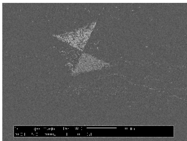
FIGURA 9: Impressão de Dureza Vickers do (GI-2 I) com aumento de 2000x
