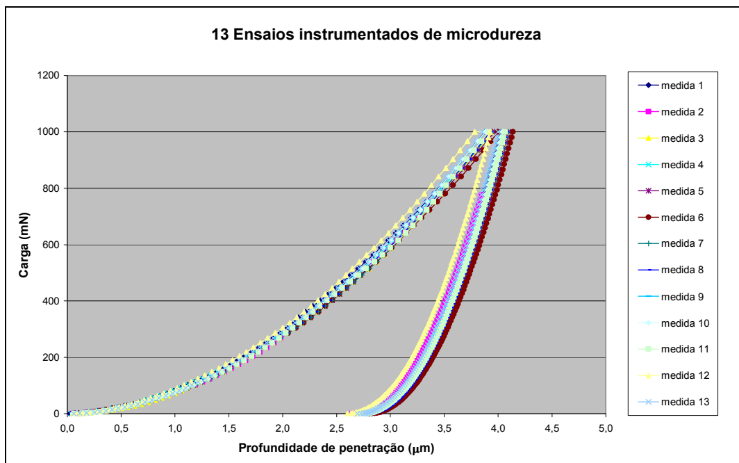
FIGURA 22a: Grupo II – Amostra 6 – Lado Controle
