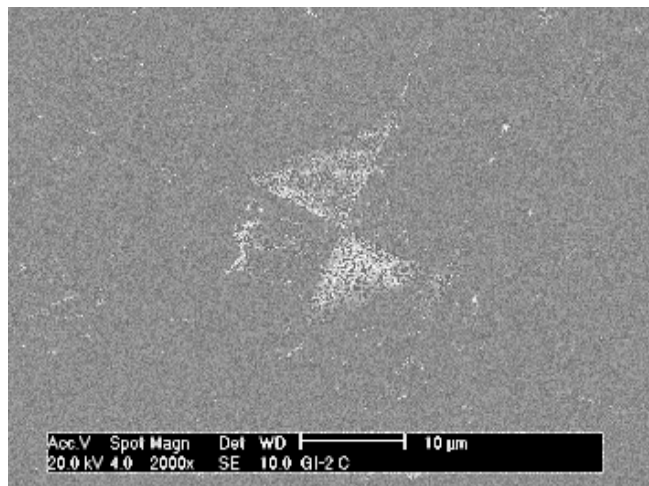
FIGURA 8: Impressão de Dureza Vickers do (GI-2 C) com aumento de 2000x
