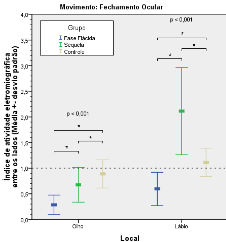
Figura 9. Gráfico de barras de erros apresentando média e desvio padrão do IEMG do movimento de fechamento ocular nos grupos estudados
