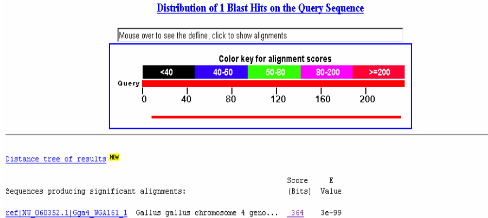
FIGURA IV.10b. Sequência do kDNA e da região flanqueadora do DNA hospedeiro no genoma de ave F1. Análise BLASTn da região flanqueadora do clone C4 apresentando 96% de identidade com elemento CR-1 de Gallus gallus .
