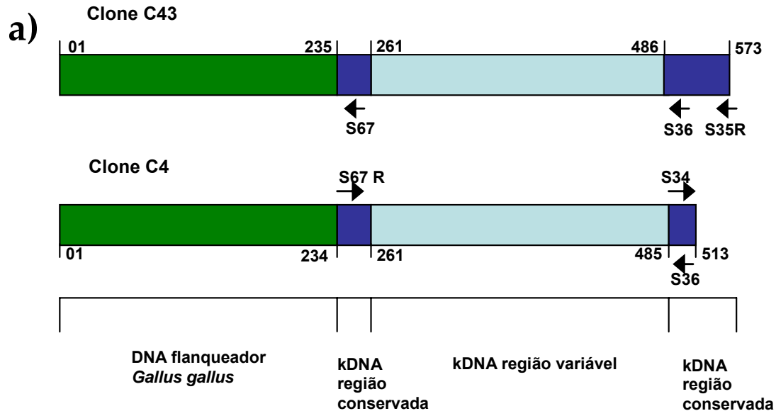
FIGURA IV.11a. Representação esquemática da integração de seqüências de minicírculos de kDNA do Trypanosoma cruzi no genoma de Gallus gallus . Em verde, região flanqueadora com alta identidade com elemento retrotransponível CR-1 no genoma da ave. Em azul escuro, região conservada de minicírculo de kDNA; e em azul claro, região variável do minicírculo.
