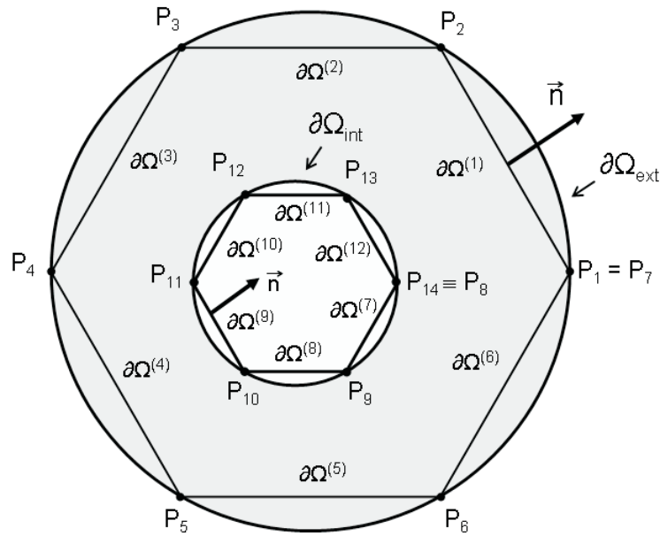
Figura 5.2: Domínio discretizado com inclusão interna
