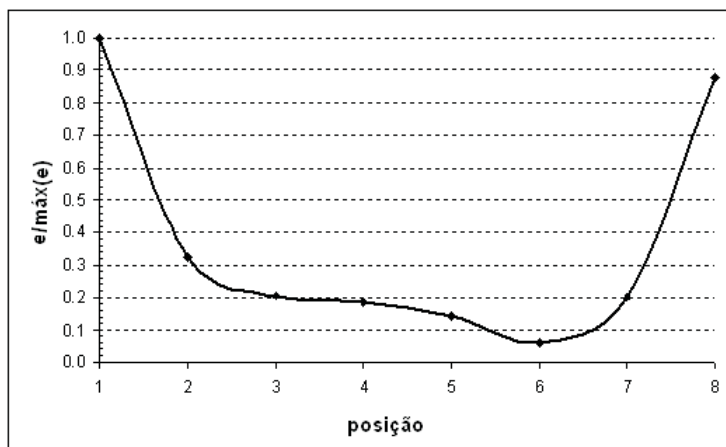
Figura 6.7: Valor normalizado do funcional de erro e para as oito posições da inclusão de prospecção
