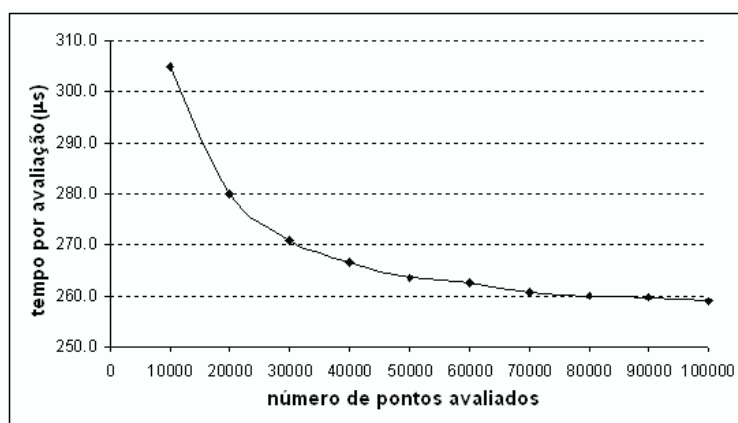
Figura 6.12: Tempo de execução do programa por ponto interno avaliado
