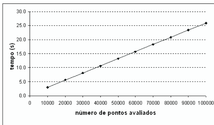
Figura 6.11: Tempo de execução do programa em função do número de pontos internos avaliados
