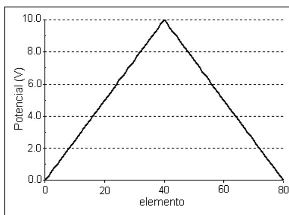
Figura 6.5: Perfil triangular de potencial aplicado sobre o contorno
