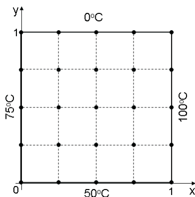
Figura 6.1: Domínio quadrado de lado unitário discretizado pelo MDF
