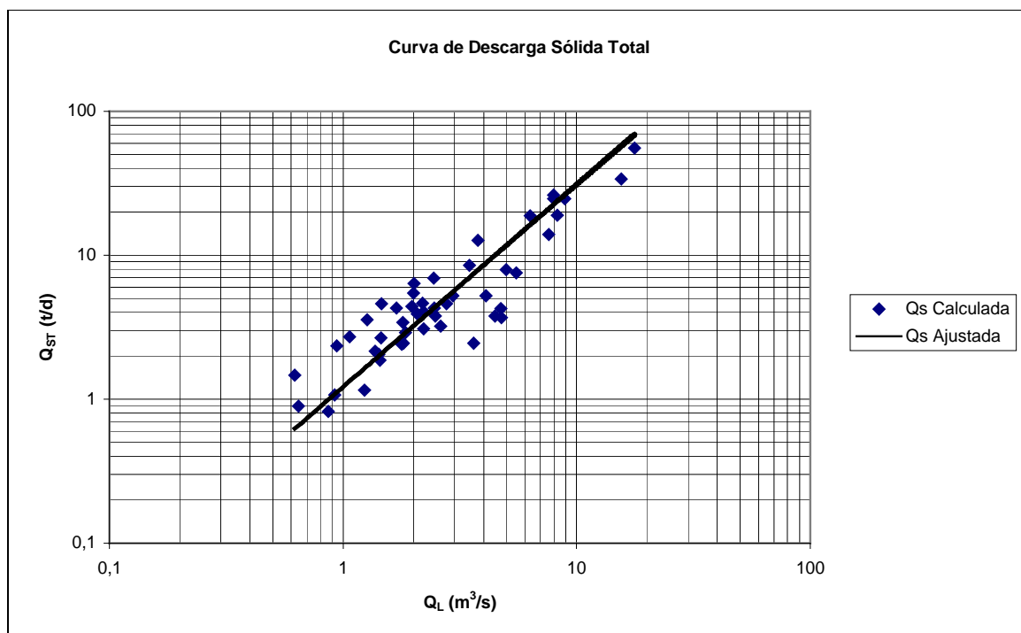
FIGURA 6.20 – CURVA DE DESCARGA SÓLIDA TOTAL
