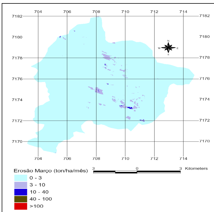
FIGURA 6.10 – PERDA DE SOLO NO MÊS DE MARÇO
