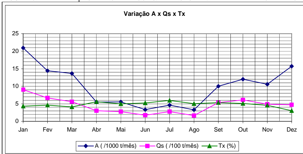
FIGURA 6.21 – VARIAÇÃO MENSAL EROSIÃO/TRANSPORTE/TAXA DE TRANSFERÊNCIA
