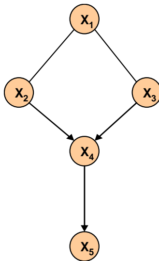
Figura 2.4. Rede Bayesiana em construção
