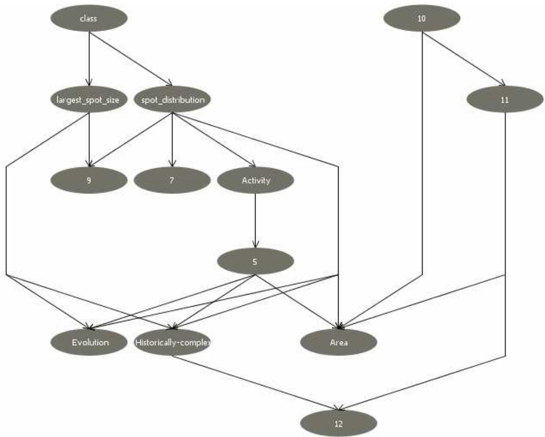
Figura 4.29. Rede Solar-Flare 1 gerada pelo PC tradicional
