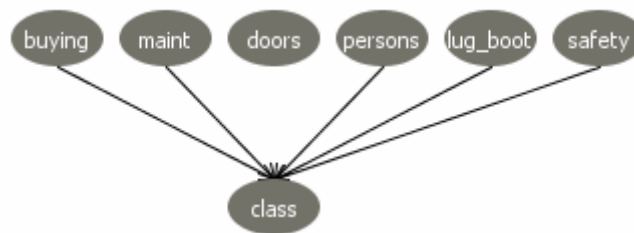
Figura 4.22. Rede Car gerada pelo PC tradicional
