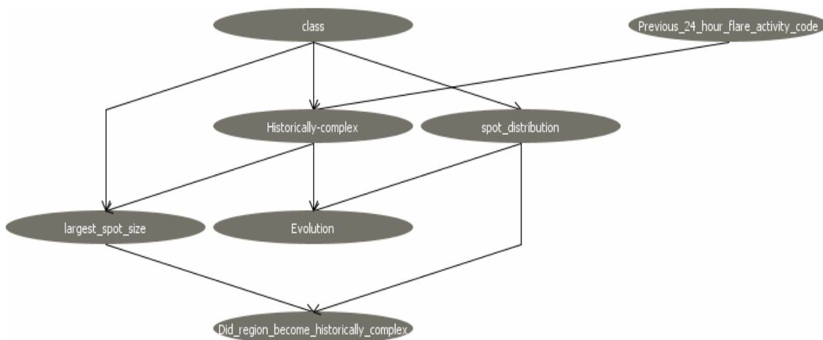
Figura 4.32. Rede Solar-Flare 2 gerada pelo MarkovPC
