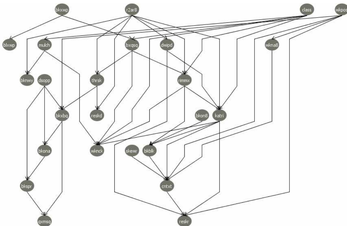
Figura 4.25. Rede Kr-vs-Kp gerada pelo algoritmo MarkovPC
