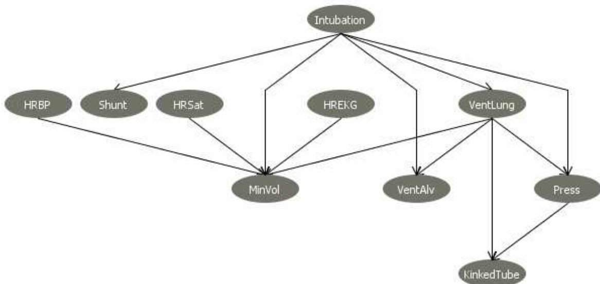
Figura 4.10. Intubation gerada por MarkovPC
