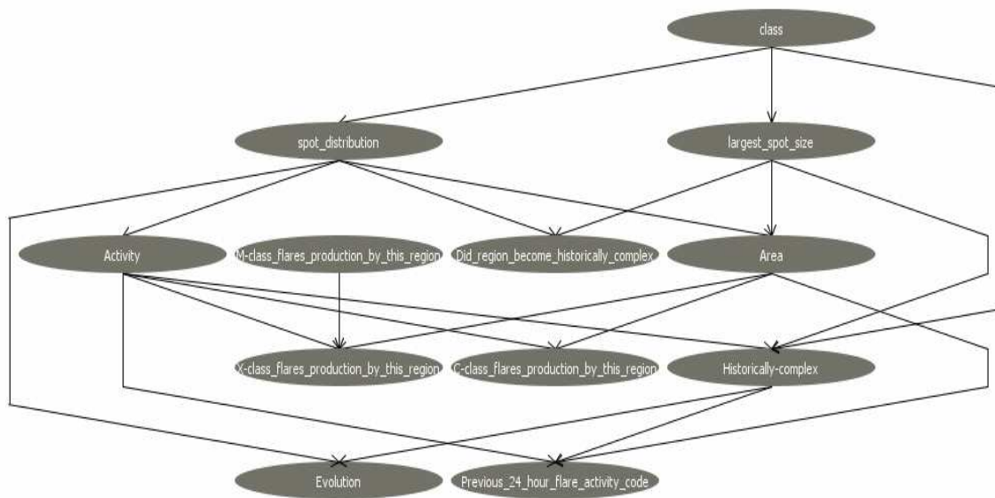
Figura 4.31. Rede Solar-Flare 2 gerada pelo PC tradicional
