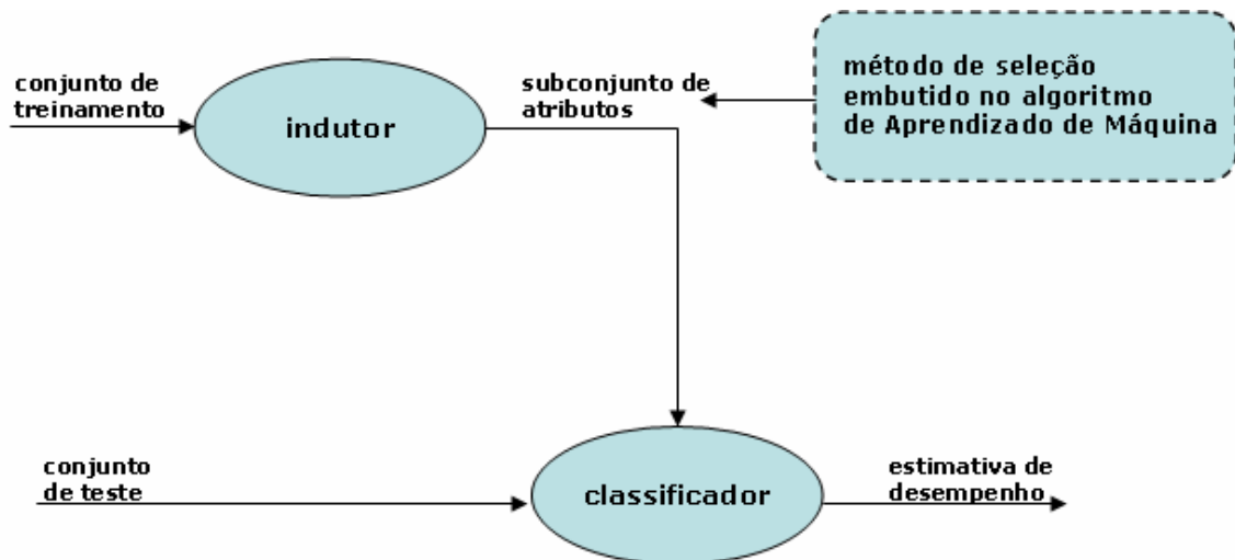
Figura 3.4. A abordagem embutida
