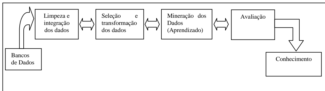
Figura 3.1. Fases do processo de extração de conhecimento de bancos de dados.
