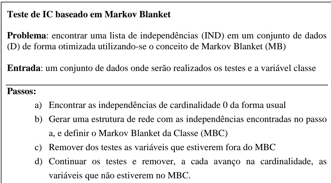
Figura 5.2. Pseudo-código do algoritmo PC, adaptado de [17,60].
