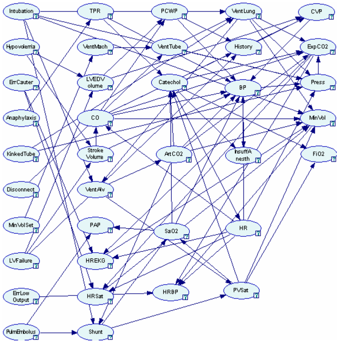
Figura 4.4. Rede ALARM gerada pelo PC tradicional
