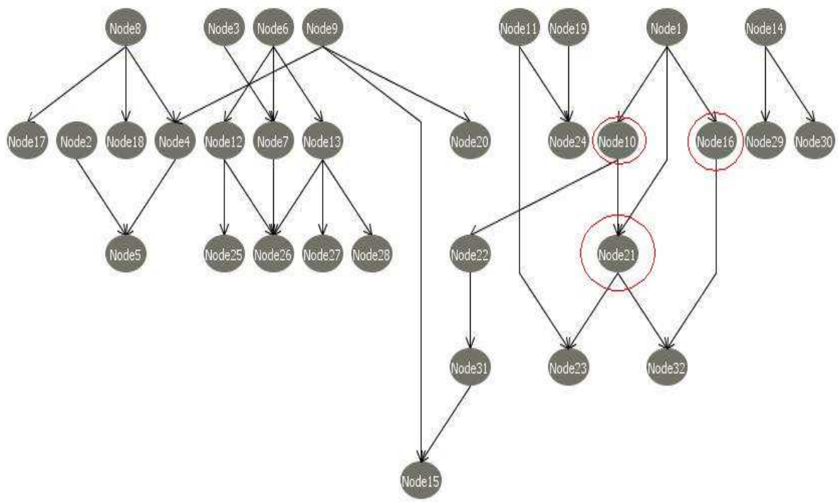
Figura 4.17. Synthetic2 gerada pelo PC tradicional
