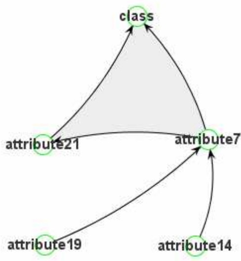
Figura 4.27. Rede Lung-Cancer gerada pelo MarkovPC
