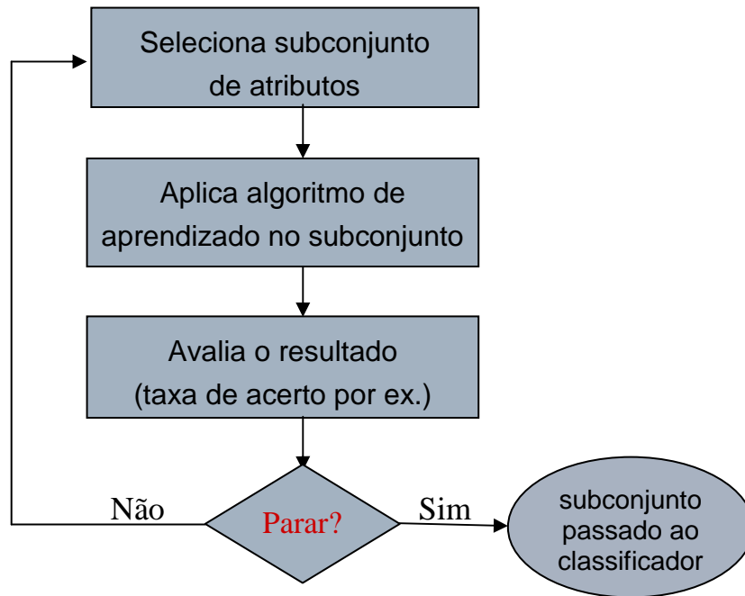
Figura 3.2. Fluxograma da abordagem wrapper
