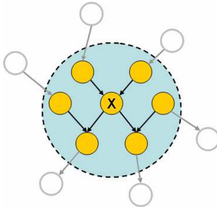
Figura 2.2. O Markov Blanket do nó X
