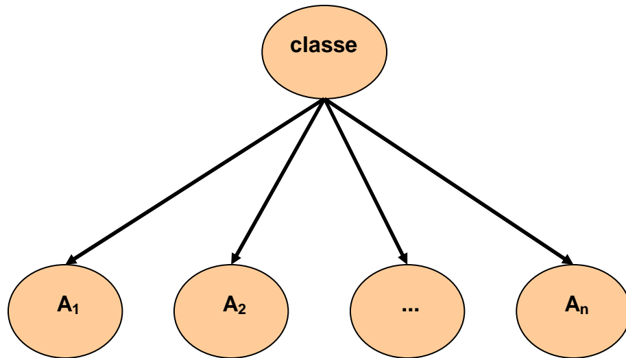
Figura 3.5. Classificador NaiveBayes
