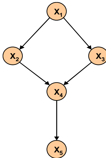
Figura 2.3. Um grafo direcionado
