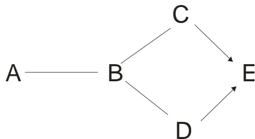
Figura 2.9. Padrão final produzido pelo PC para o exemplo anterior [44].
