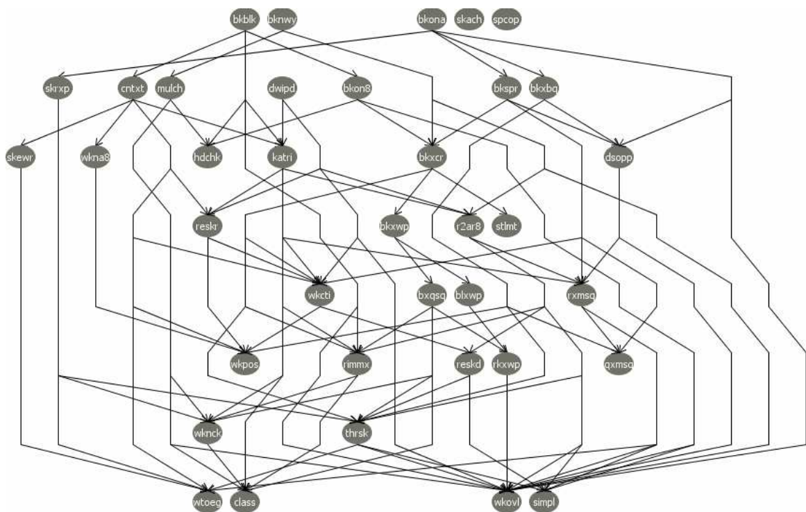
Figura 4.24. Rede Kr-vs-Kp gerada pelo algoritmo PC tradicional
