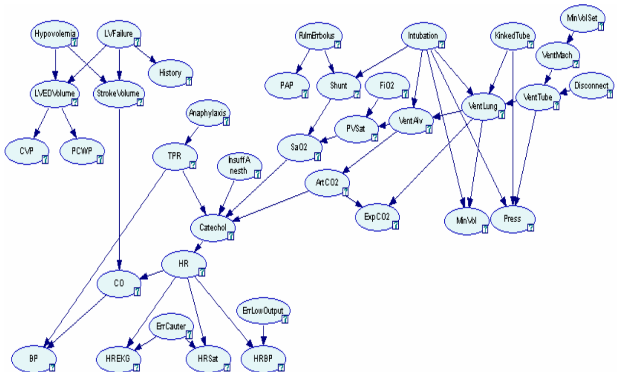
Figura 4.3. Rede Bayesiana original ALARM [56]
