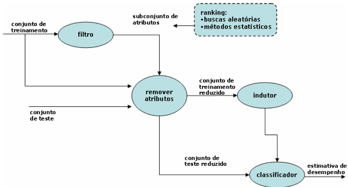
Figura 3.3. A abordagem filtro
