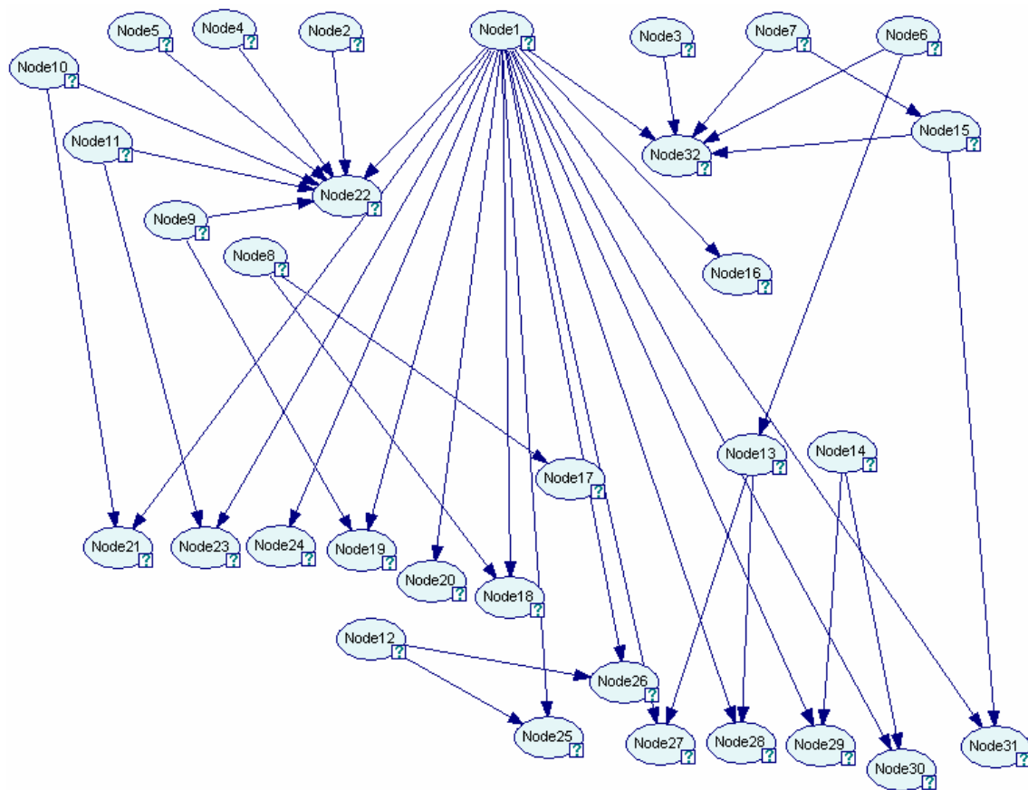
Figura 4.19. Rede Synthetic3
