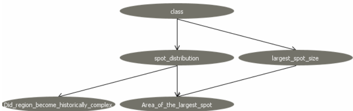
Figura 4.30. Rede Solar-Flare 1 gerada pelo MarkovPC
